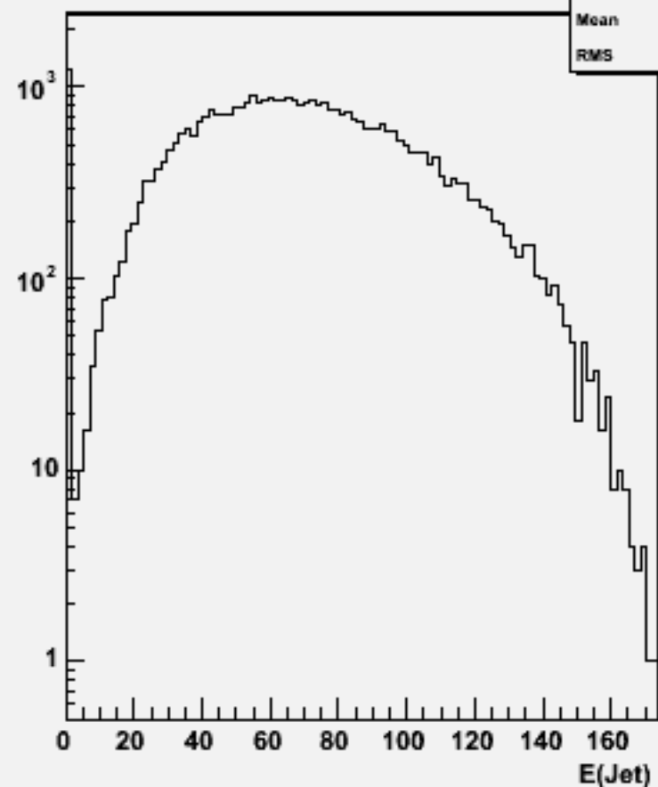
Jet energies(All jets)w103522 ae1_n1csuu_o
