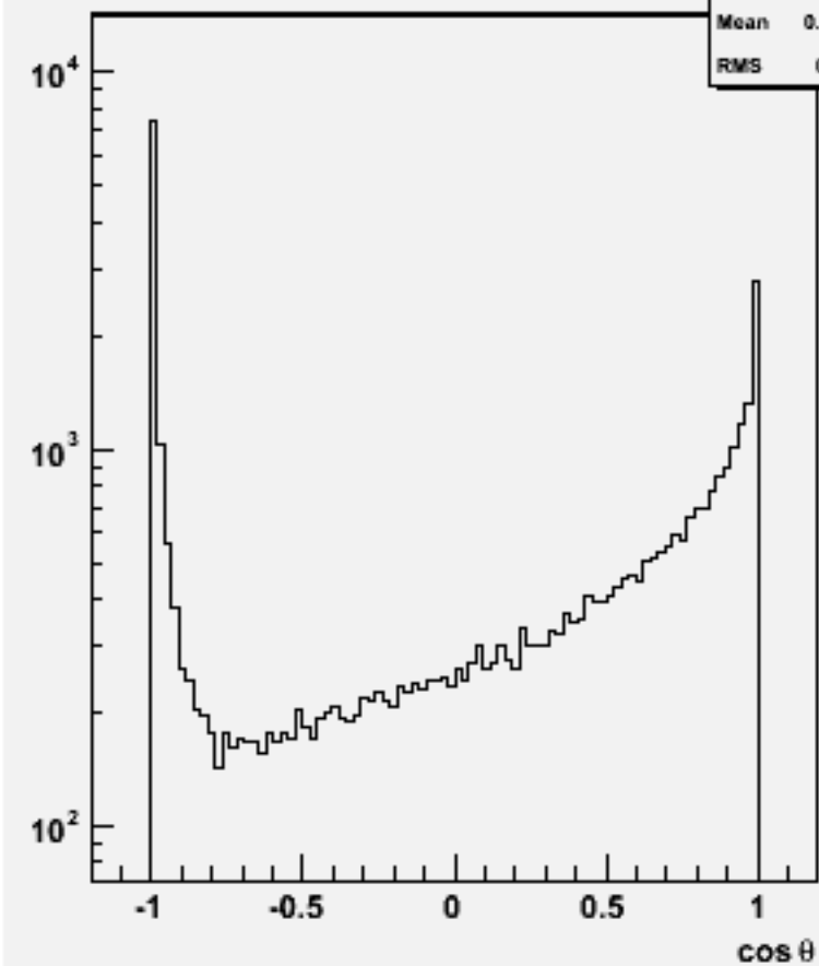
Jet cos \theta (All jets)w103432 e1a_e1bbbb_o
