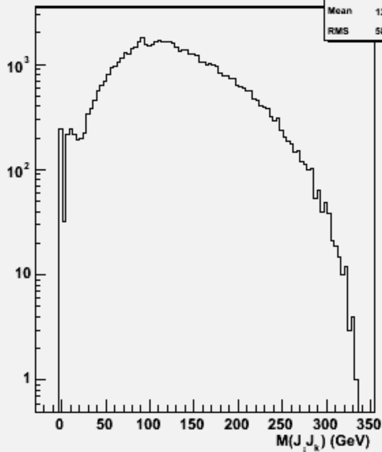
2jets mass(All comb)w103432 e1a_e1bbbb_o
