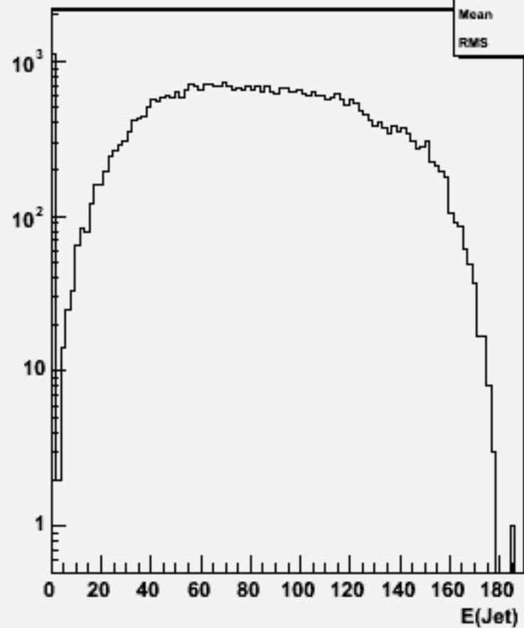
Jet energies(All jets)w103432 e1a_e1bbbb_o
