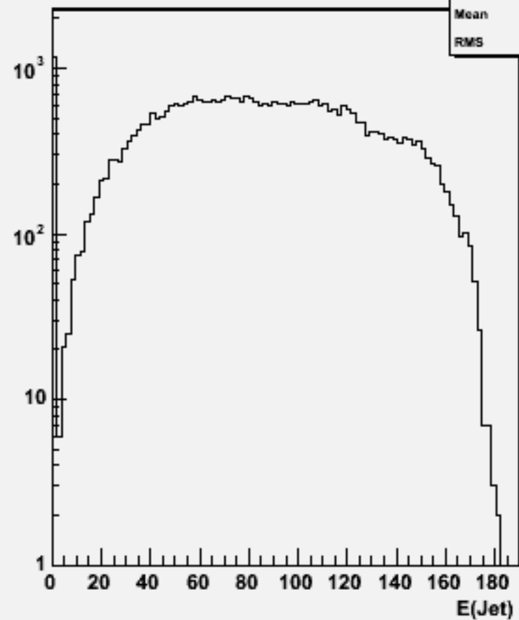
Jet energies(All jets)w103428 e1a_e1ssbb_o
