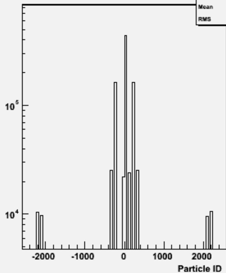
Particle ID : w103426 e1a_e1ssbb_o
