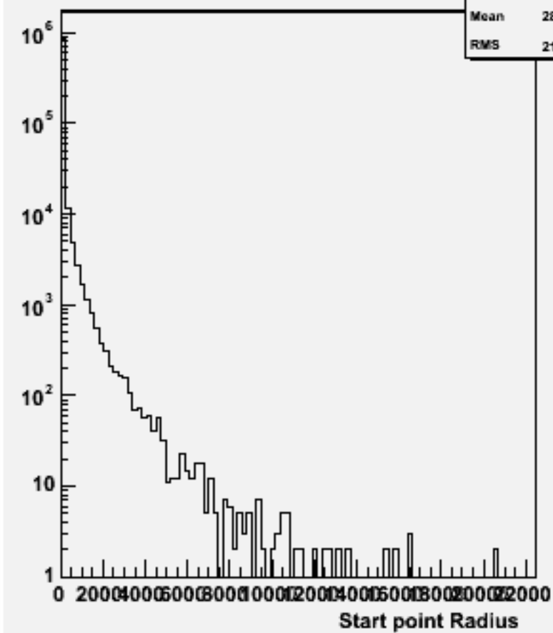
Start point R : w103426 e1a_e1ssbb_o
