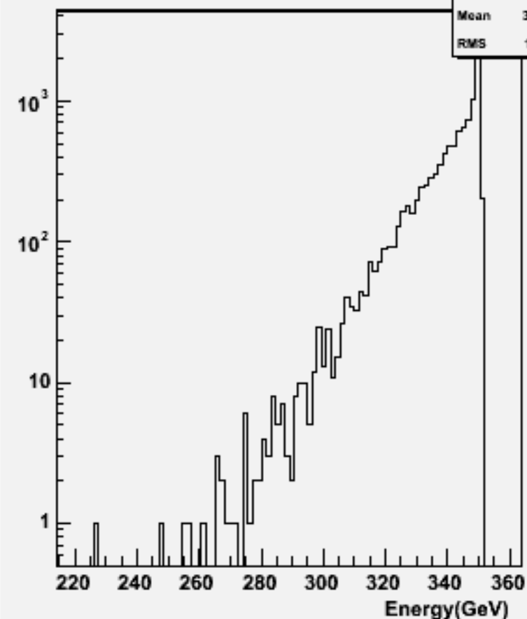
Thrust w103426 e1a_e1ssbb_o
