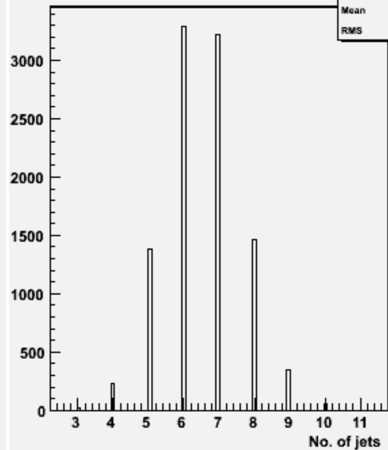
No. jets (ycut=0.001) : w103426 e1a_e1ssbb_o
