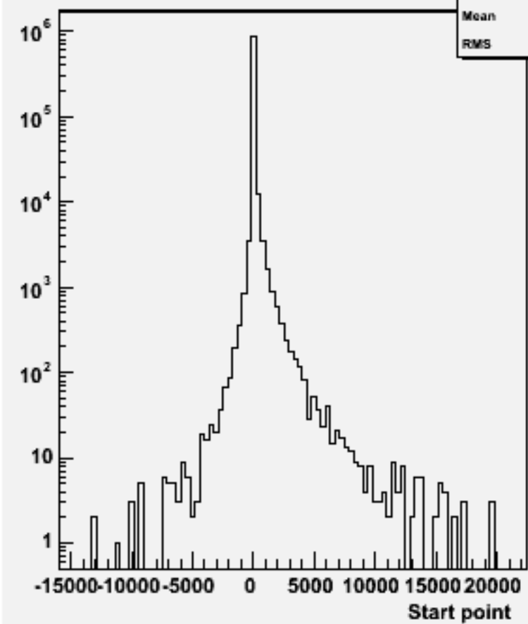
Start point Z : w103426 e1a_e1ssbb_o
