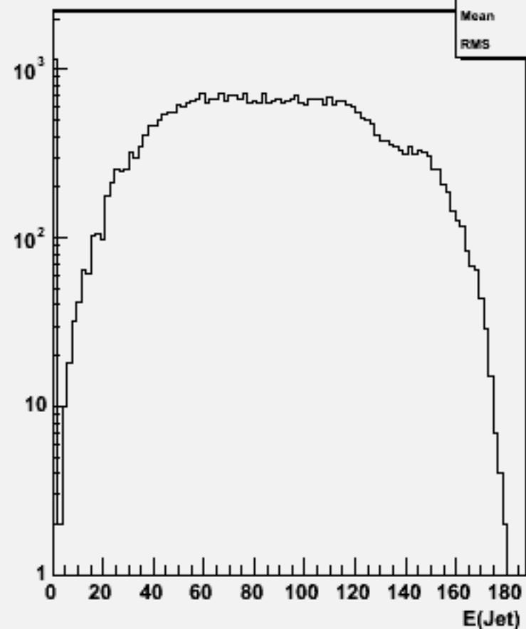
Jet energies(All jets)w103426 e1a_e1ssbb_o
