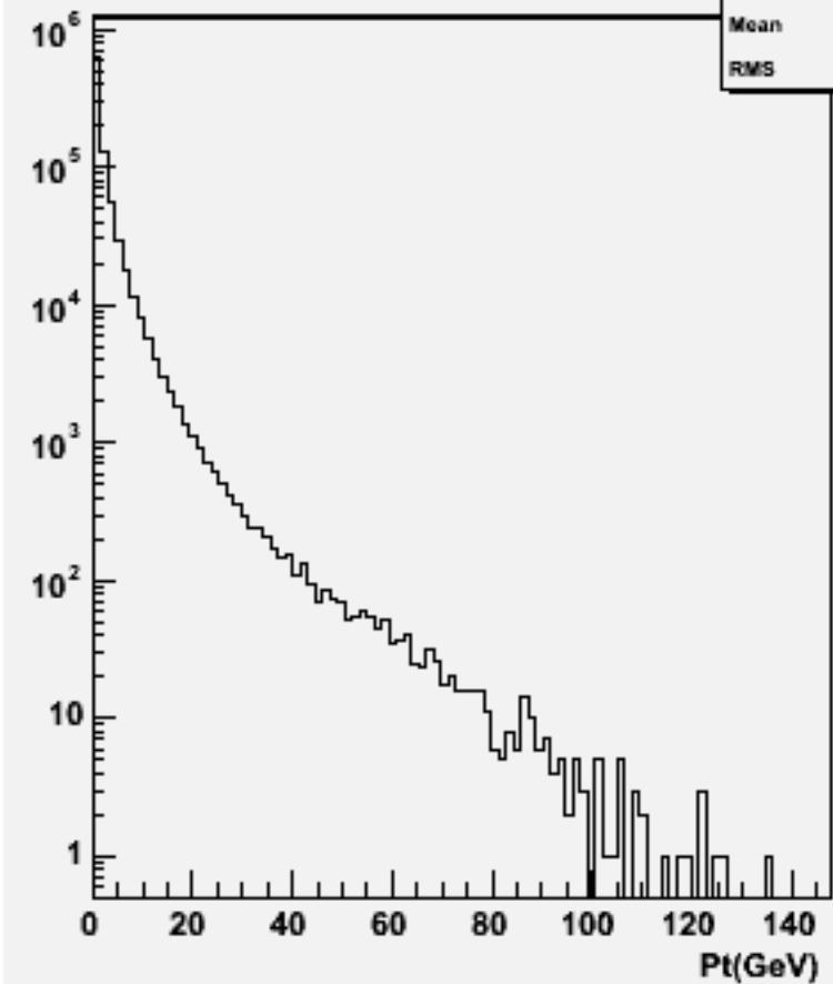
Particle Pt : w103426 e1a_e1ssbb_o
