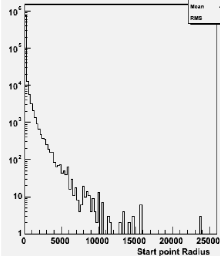
Start point R : w103422 e1a_e1ssss_o
