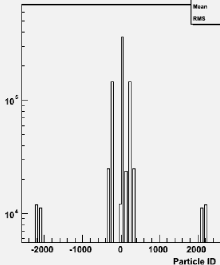
Particle ID : w103422 e1a_e1ssss_o
