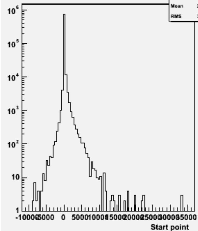
Start point Z : w103422 e1a_e1ssss_o
