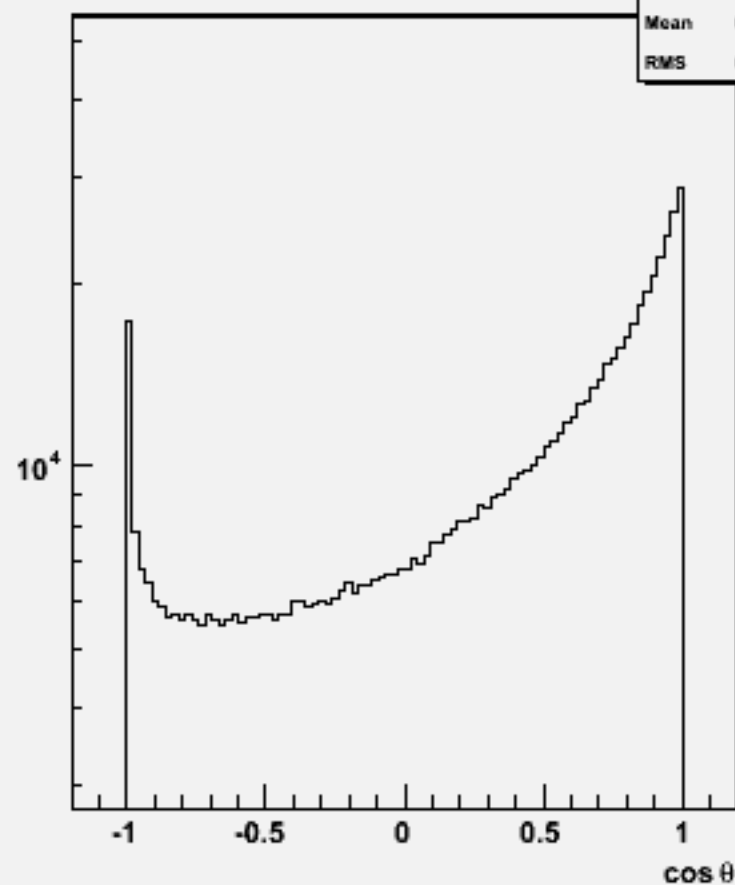
Particle cosθ : w103422 e1a_e1ssss_o
