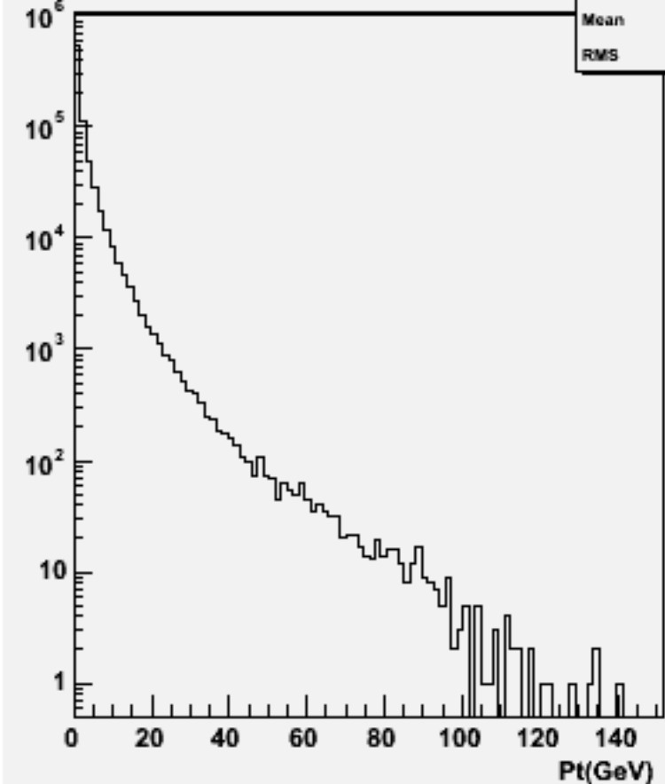
Particle Pt : w103422 e1a_e1ssss_o
