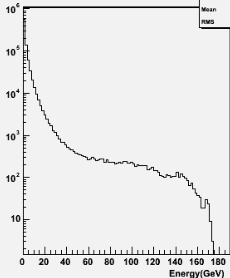
Particle Energy : w103420 e1a_e1ddbb_o
