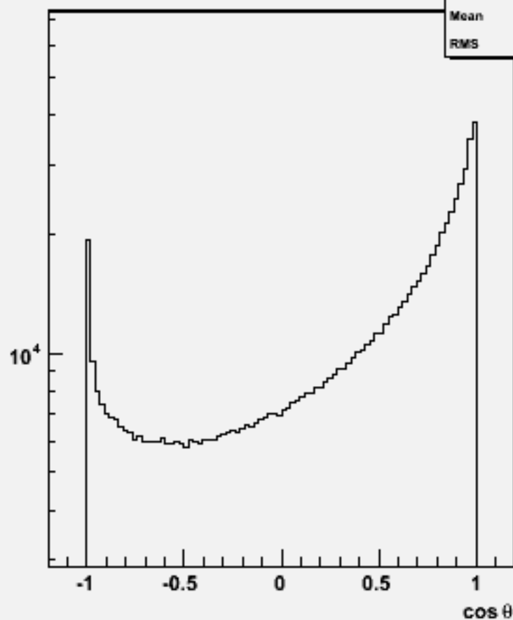
Particle cos \theta : w103420 e1a_e1ddbb_o
