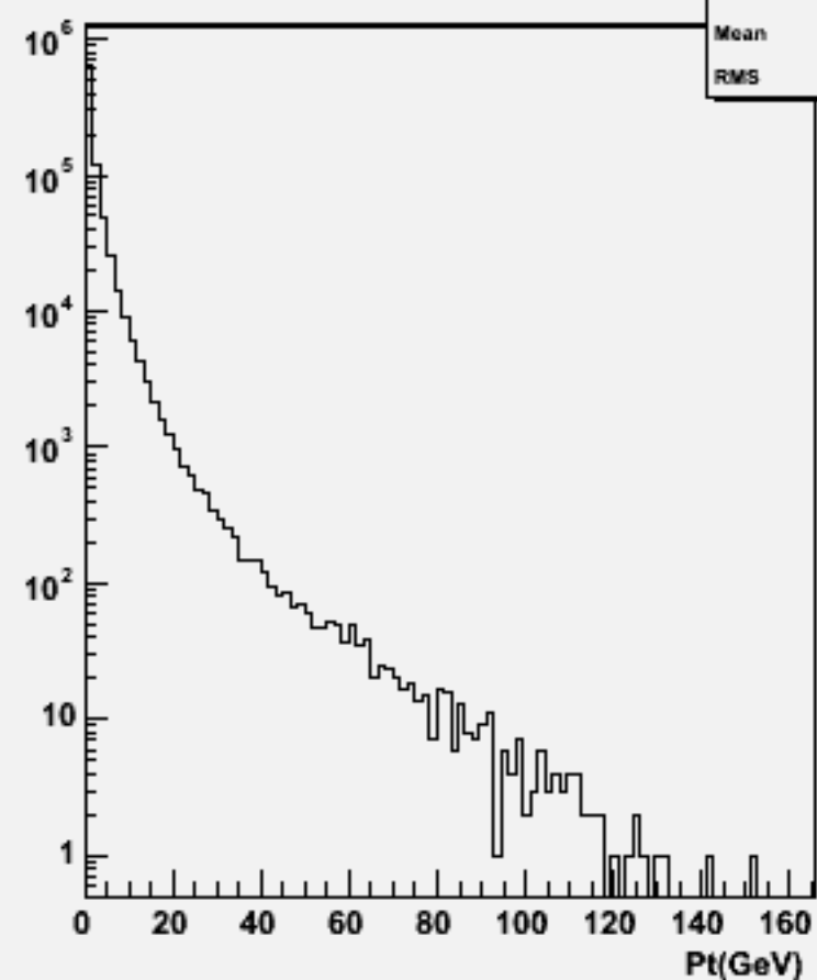
Particle Pt : w103420 e1a_e1ddbb_o
