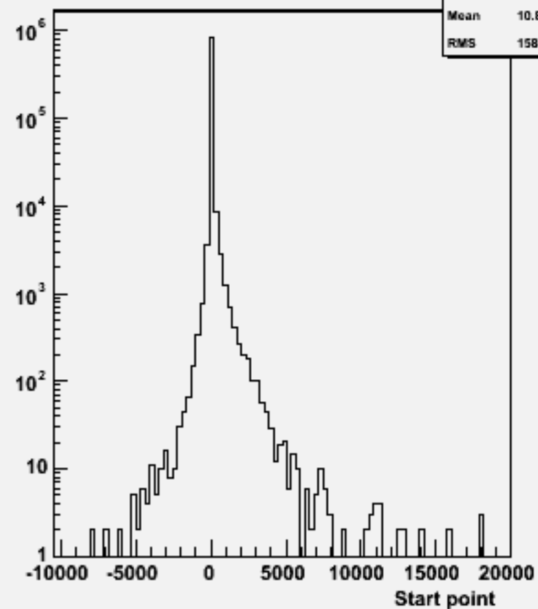
Start point Z : w103420 e1a_e1ddbb_o
