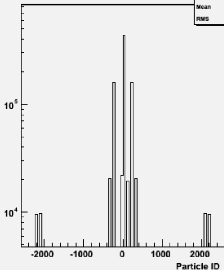
Particle ID : w103420 e1a_e1ddbb_o
