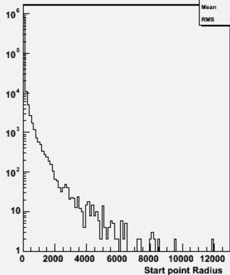
Start point R : w103420 e1a_e1ddbb_o
