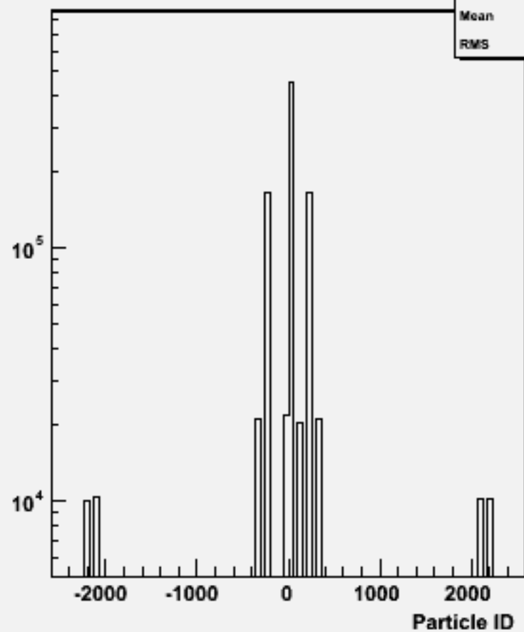
Particle ID : w103418 e1a_e1ddbb_o
