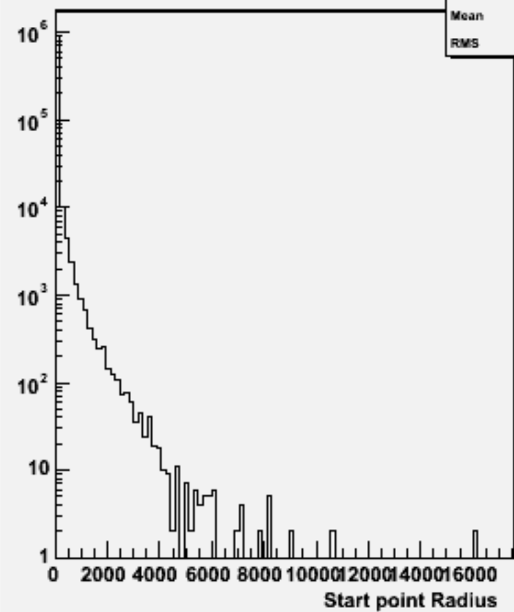
Start point R : w103418 e1a_e1ddbb_o
