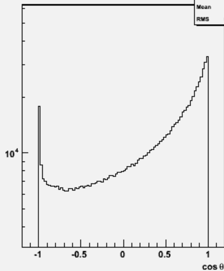
Particle cosθ : w103418 e1a_e1ddbb_o
