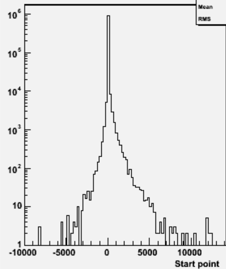
Start point Z : w103418 e1a_e1ddbb_o
