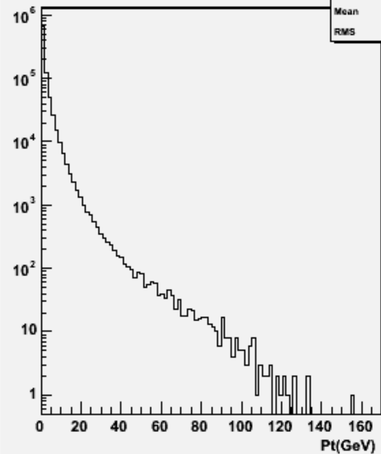
Particle Pt : w103418 e1a_e1ddbb_o
