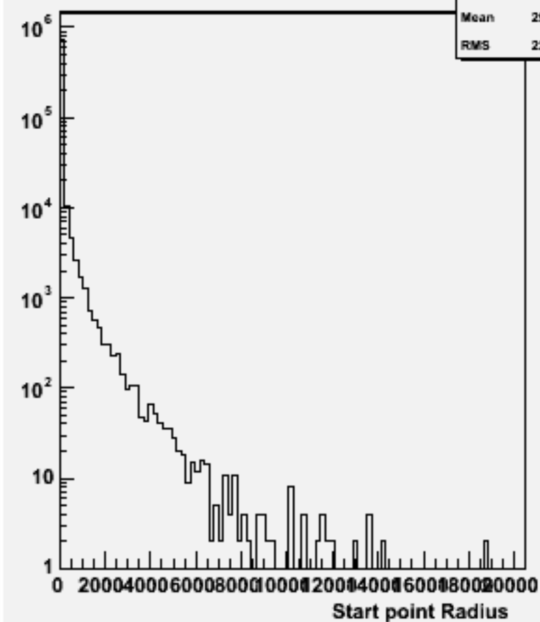
Start point R : w103416 e1a_e1ddss_o
