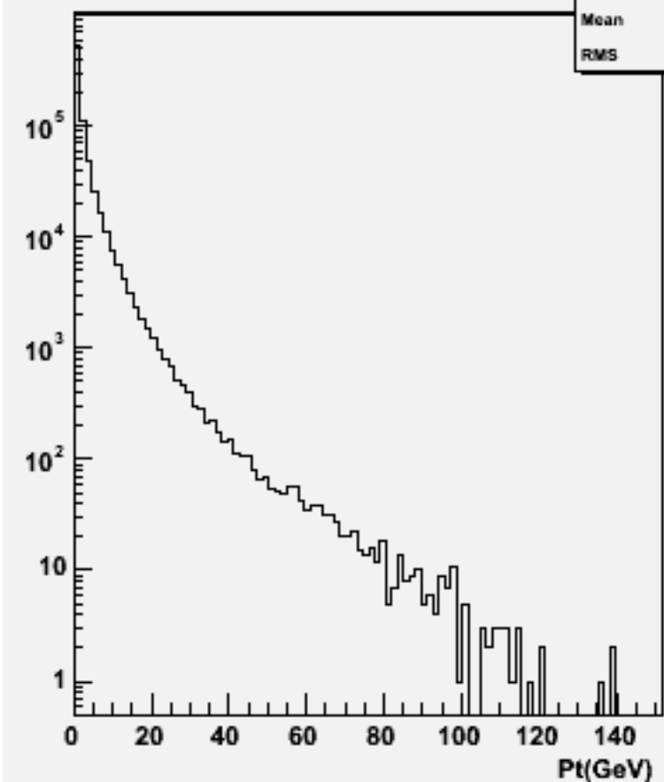
Particle Pt : w103416 e1a_e1ddss_o
