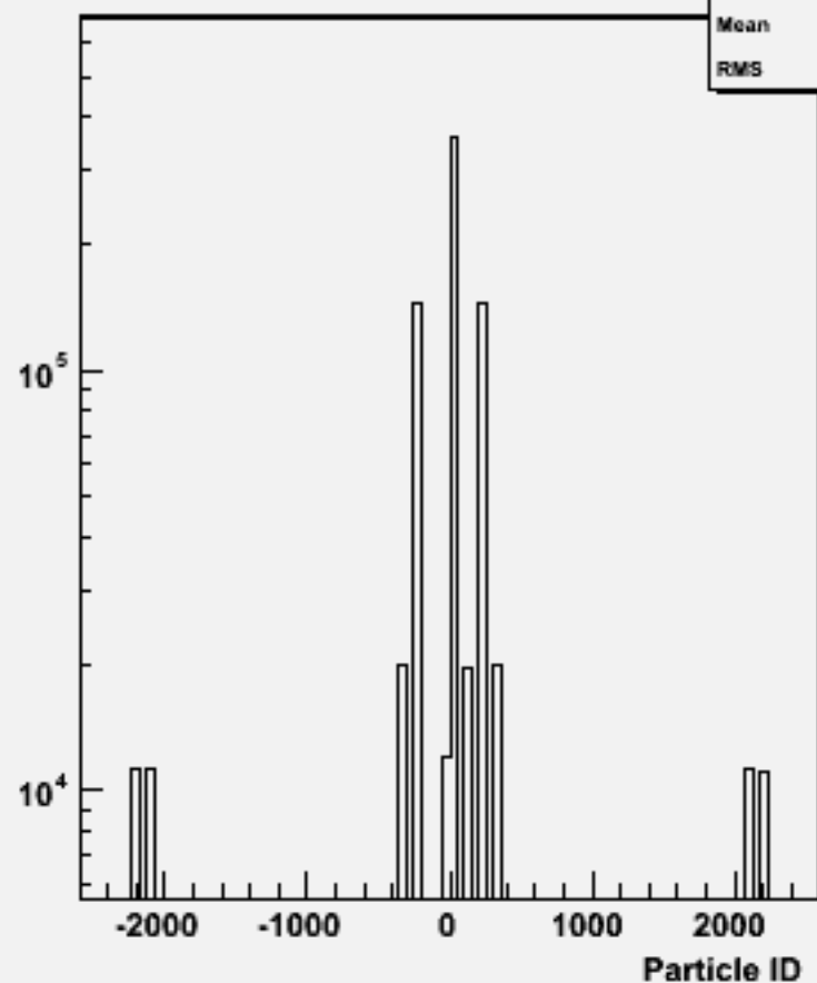
Particle ID : w103416 e1a_e1ddss_o
