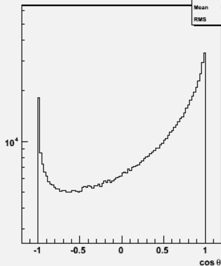
Particle cosθ : w103416 e1a_e1ddss_o
