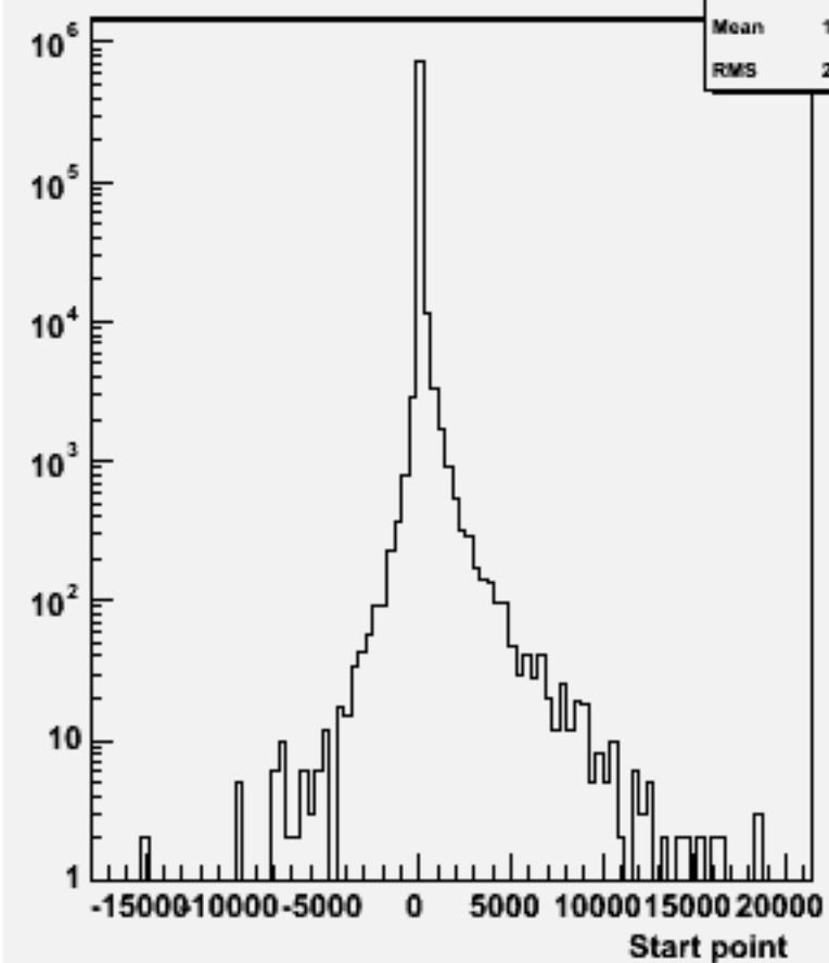
Start point Z : w103416 e1a_e1ddss_o
