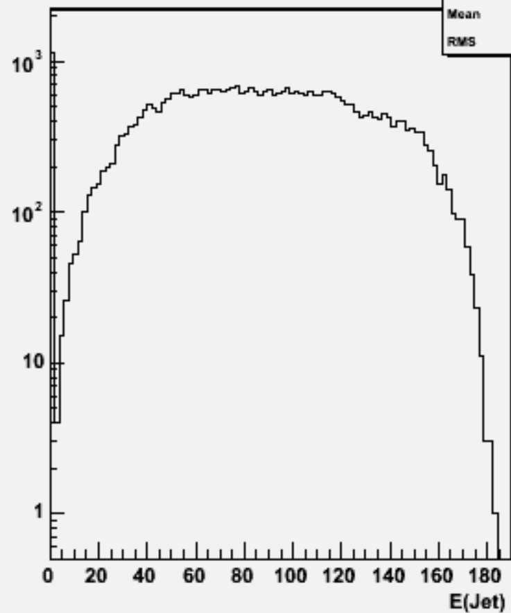
Jet energies(All jets)w103412 e1a_e1dddd_o
