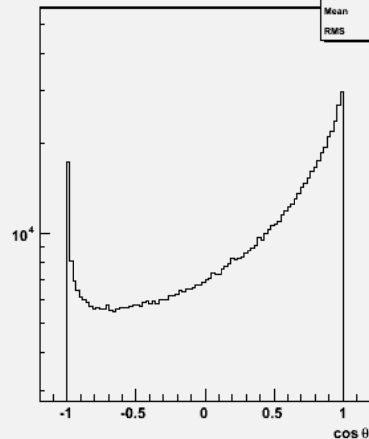
Particle cos \theta : w103410 e1a_e1dddd_o
