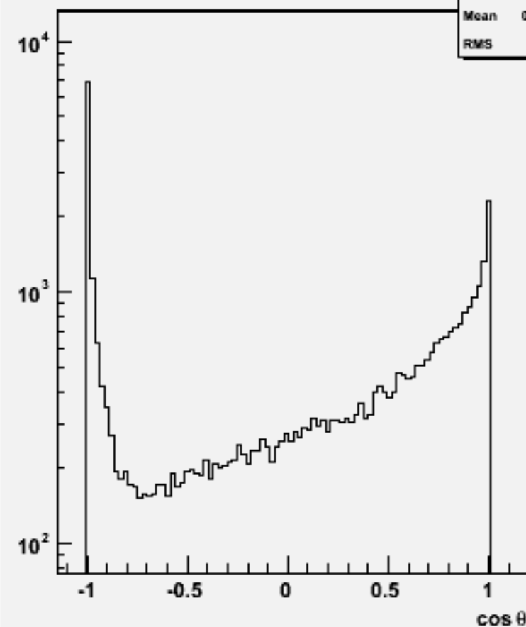
Jet cos \theta (All jets)w103410 e1a_e1dddd_o
