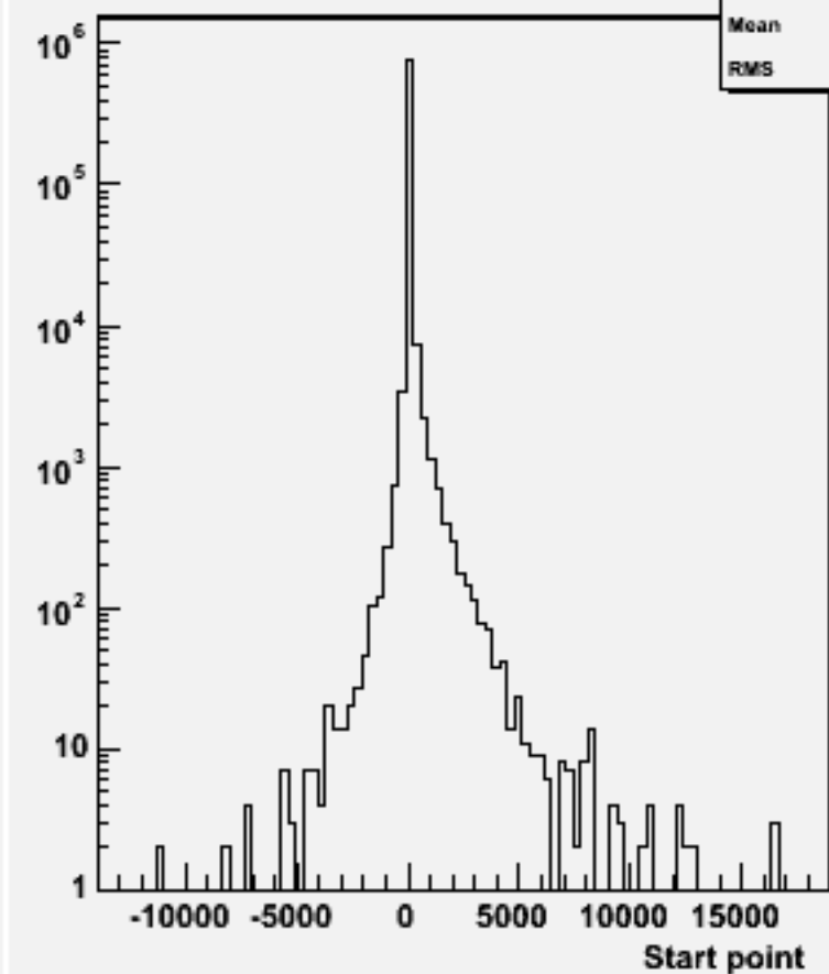
Start point Z : w103410 e1a_e1dddd_o
