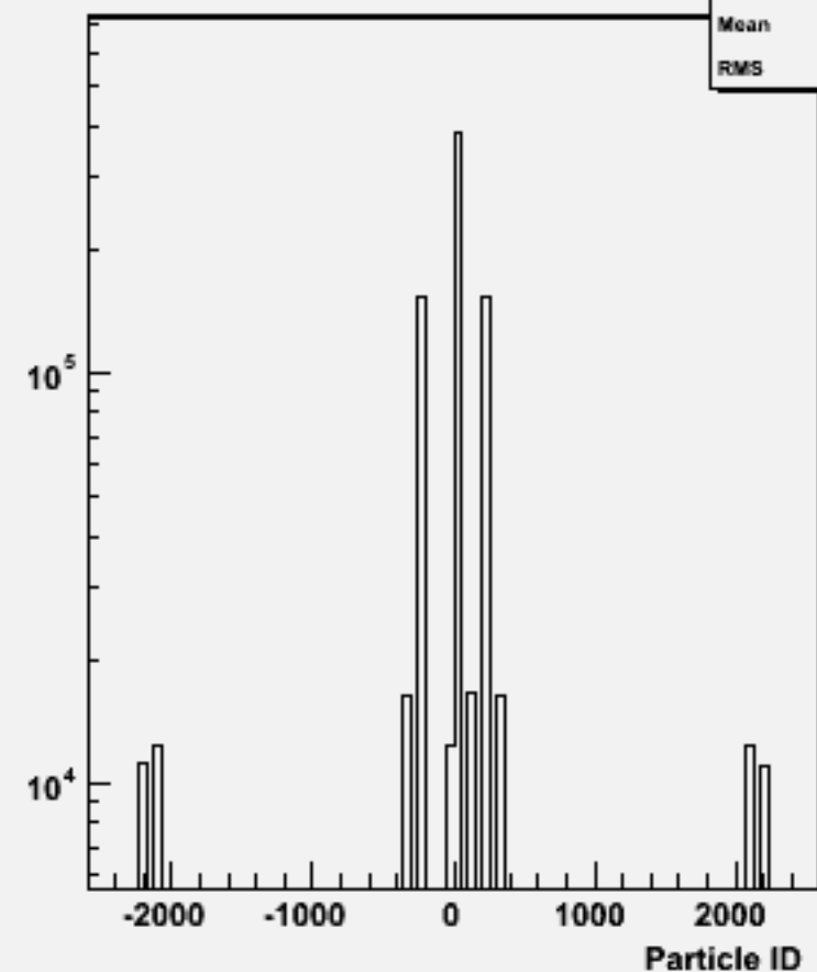
Particle ID : w103410 e1a_e1dddd_o
