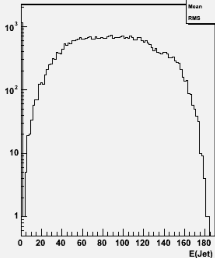
Jet energies(All jets)w103410 e1a_e1dddd_o
