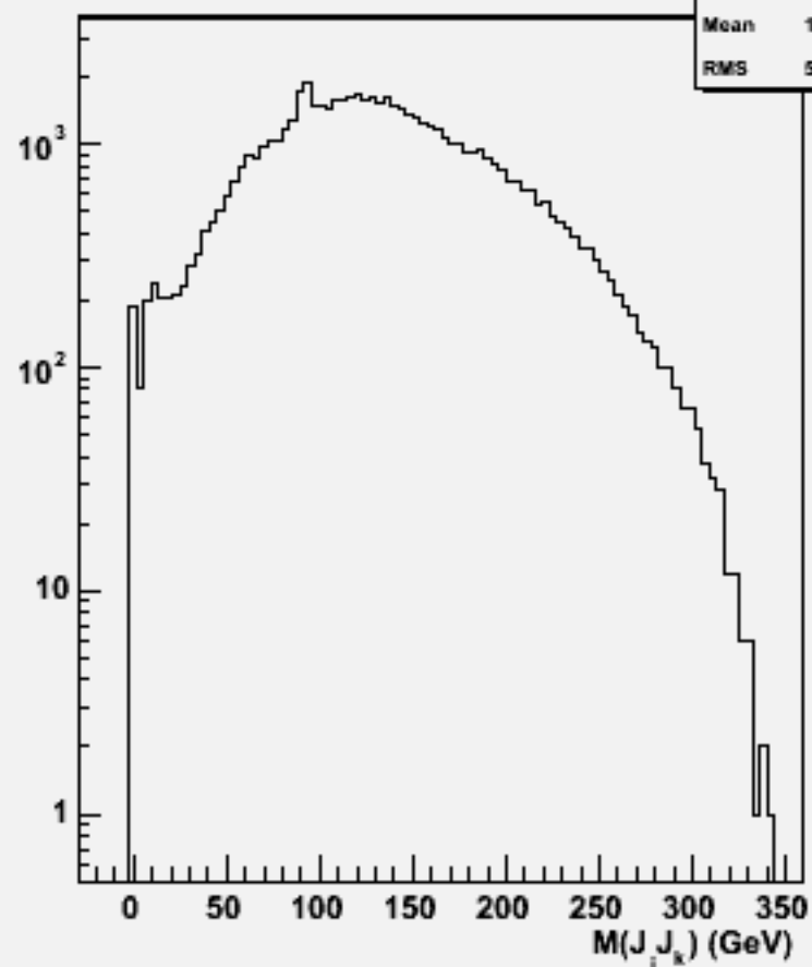
2jets mass(All comb)w103410 e1a_e1dddd_o
