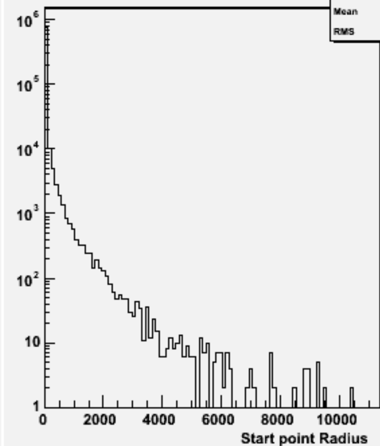
Start point R : w103410 e1a_e1dddd_o
