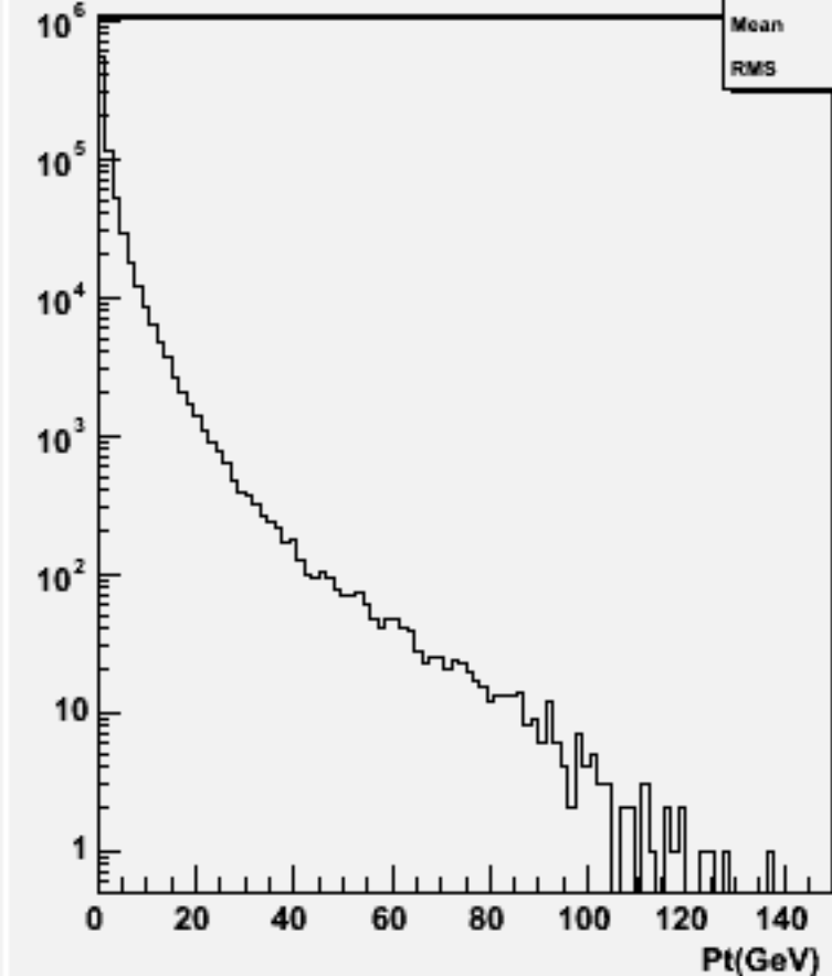
Particle Pt : w103410 e1a_e1dddd_o
