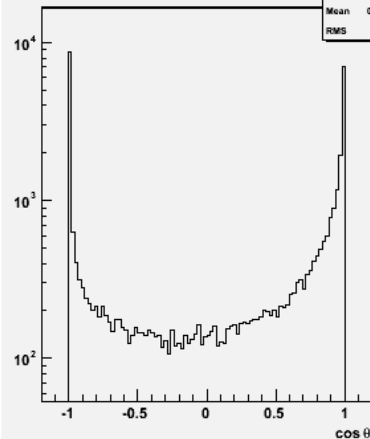
Jet cos \theta (All jets)w103408 e1a_e1e3e3bb_o
