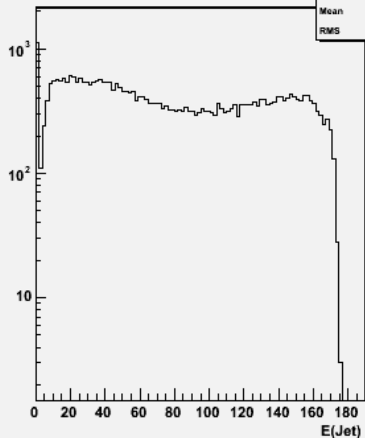
Jet energies(All jets)w103408 e1a_e1e3e3bb_o
