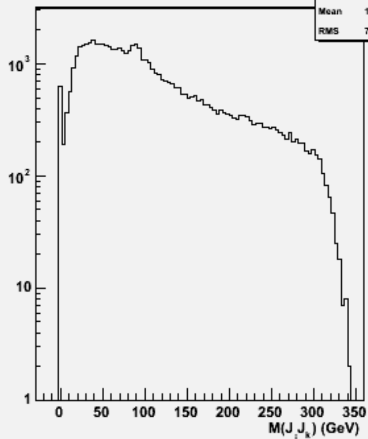
2jets mass(All comb)w103408 e1a_e1e3e3bb_o
