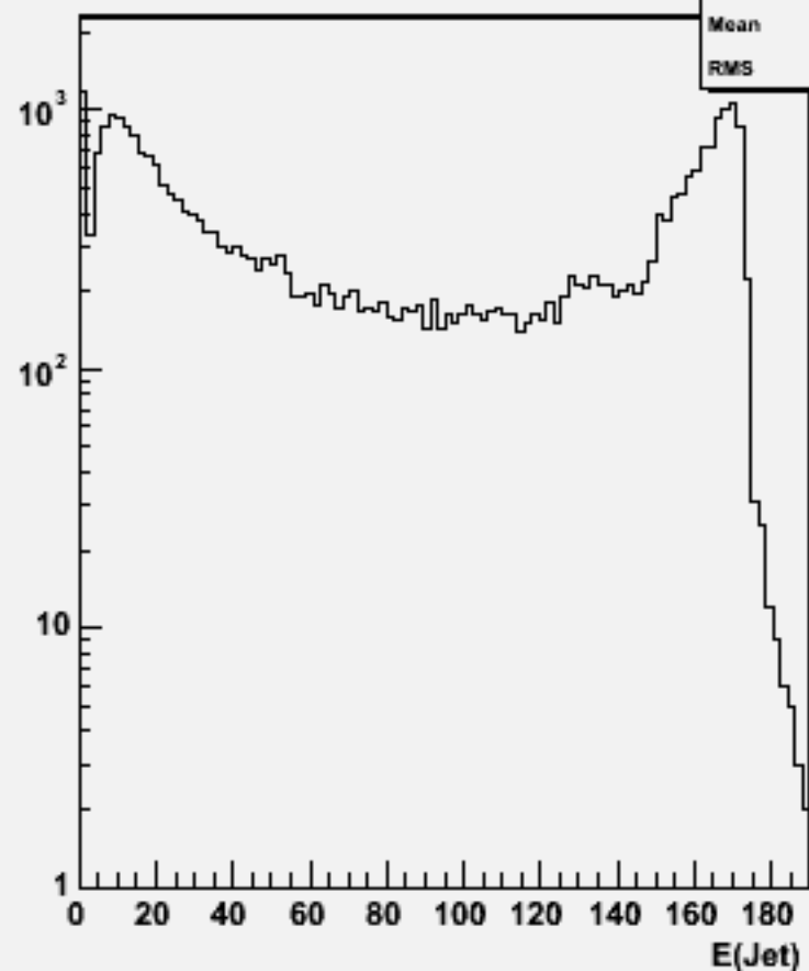
Jet energies(All jets)w103405 e1a_e1e3e3ss_o
