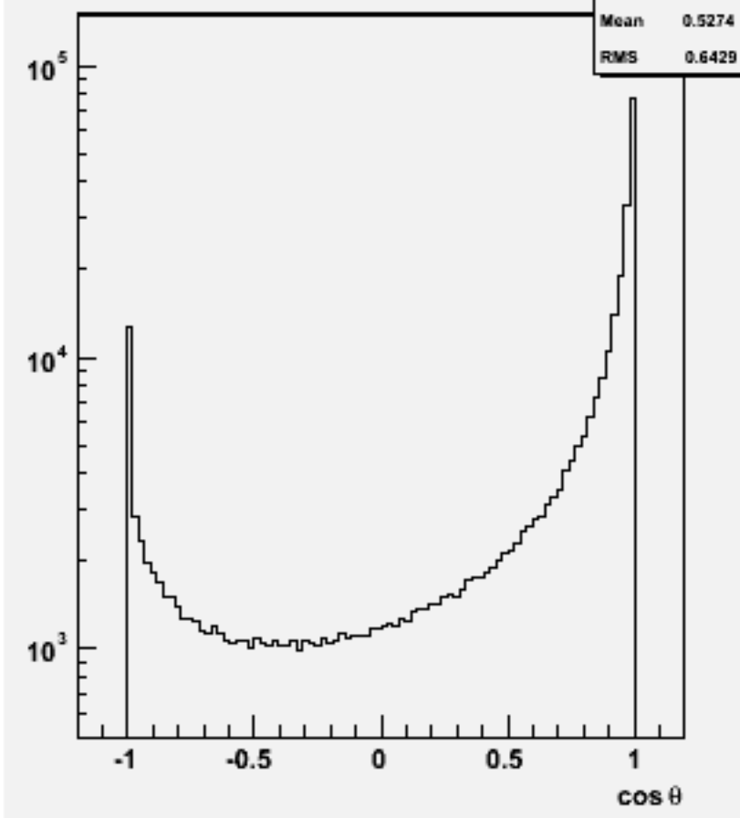
Particle cos \theta : w103405 e1a_e1e3e3ss_o
