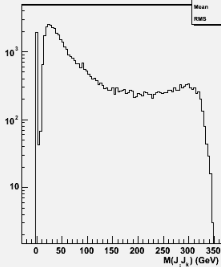
2jets mass(All comb)w103405 e1a_e1e3e3ss_o
