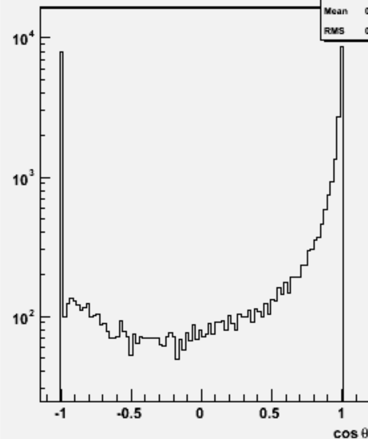
Jet cos \theta (All jets)w103405 e1a_e1e3e3ss_o
