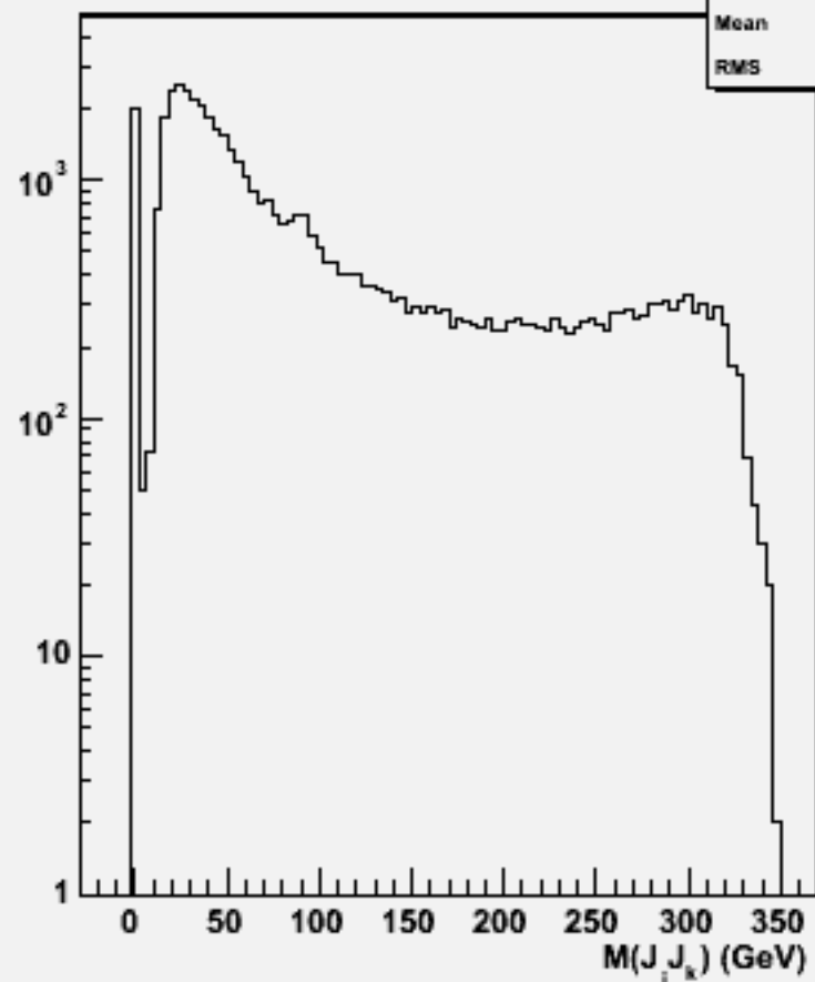
2jets mass(All comb)w103403 e1a_e1e3e3ss_o
