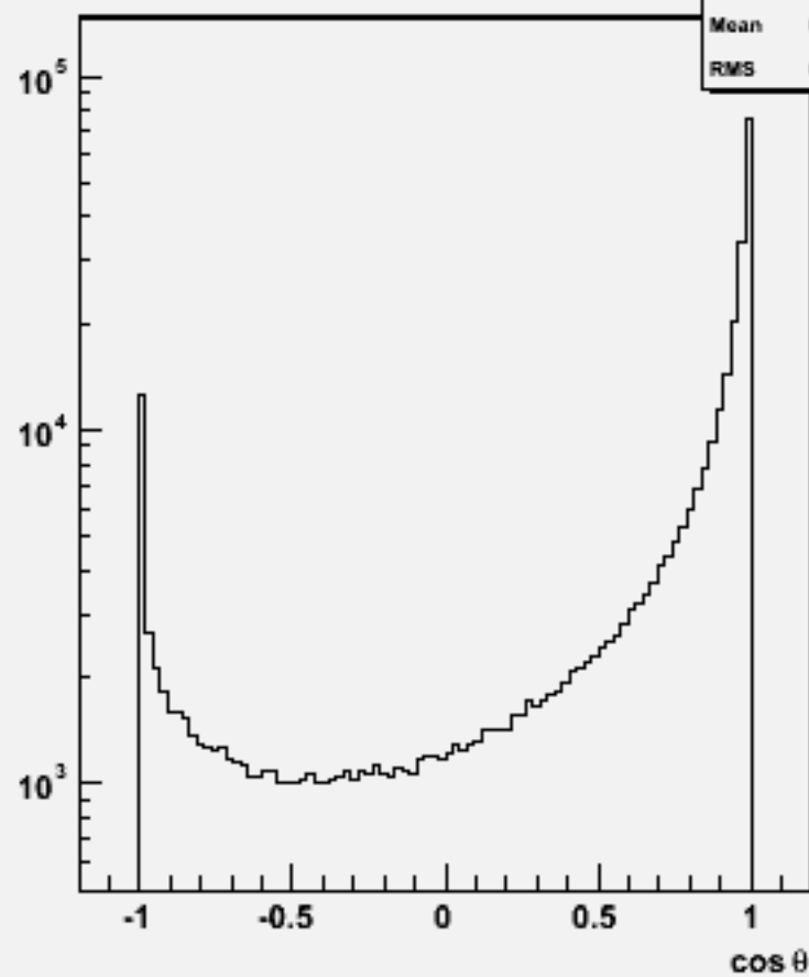
Particle cos \theta : w103403 e1a_e1e3e3ss_o
