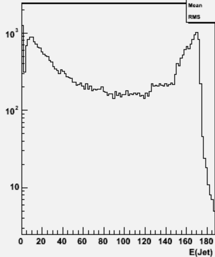
Jet energies(All jets)w103403 e1a_e1e3e3ss_o
