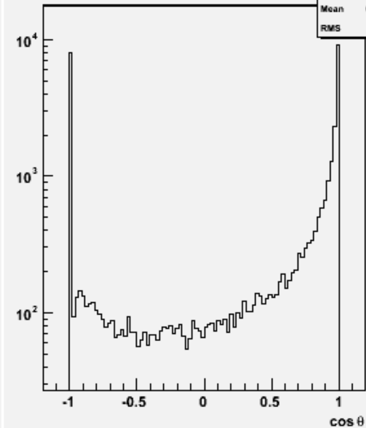
Jet cos \theta (All jets)w103403 e1a_e1e3e3ss_o
