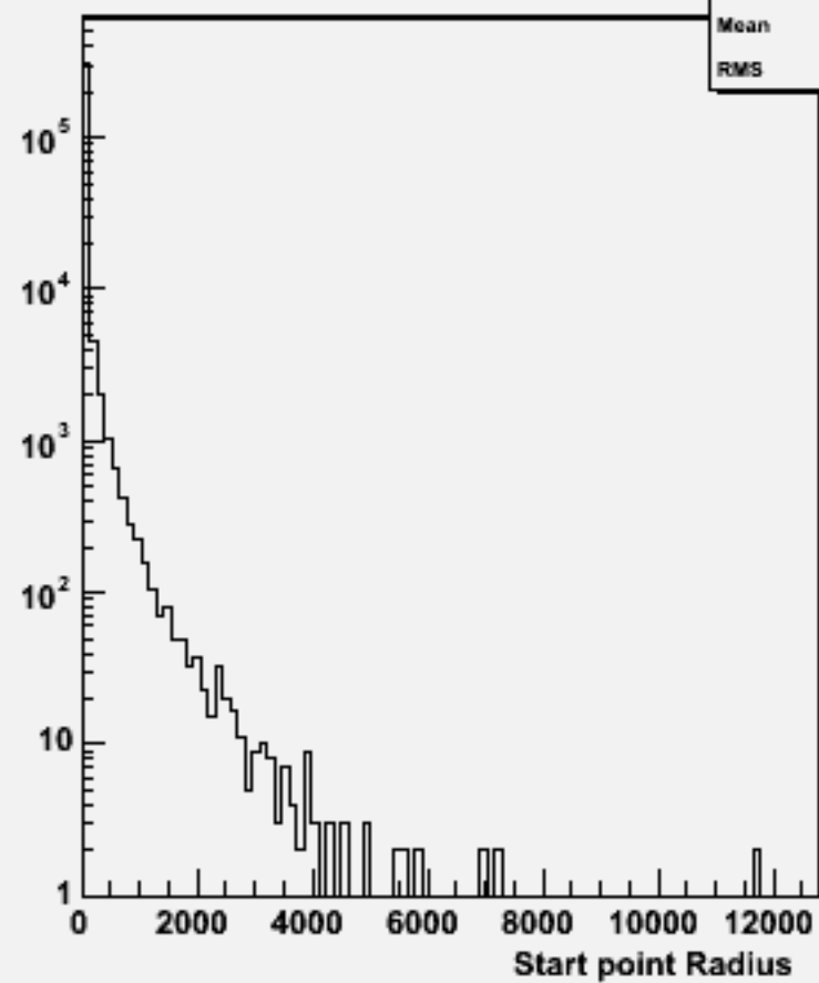
Start point R : w103403 e1a_e1e3e3ss_o
