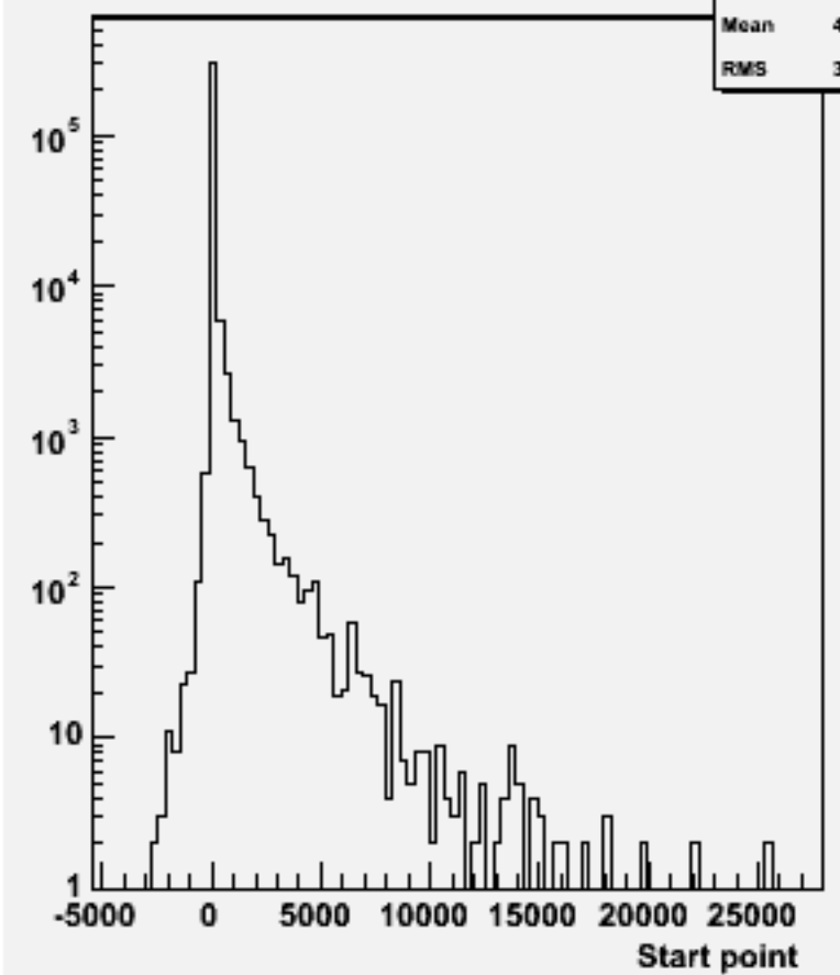
Start point Z : w103403 e1a_e1e3e3ss_o
