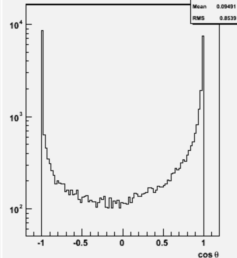
Jet cos theta (All jets)w103400 e1a_e1e3e3dd_o
