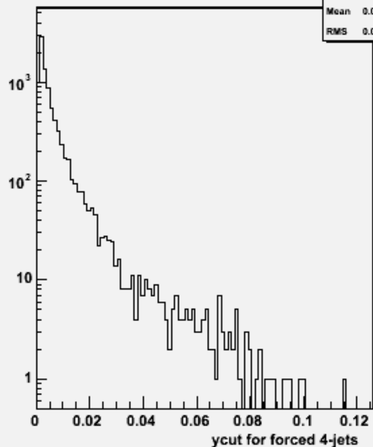
Ycut for 4-jets :w103400 e1a_e1e3e3dd_o
