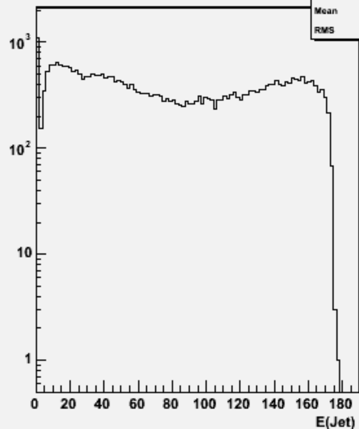
Jet energies(All jets)w103400 e1a_e1e3e3dd_o
