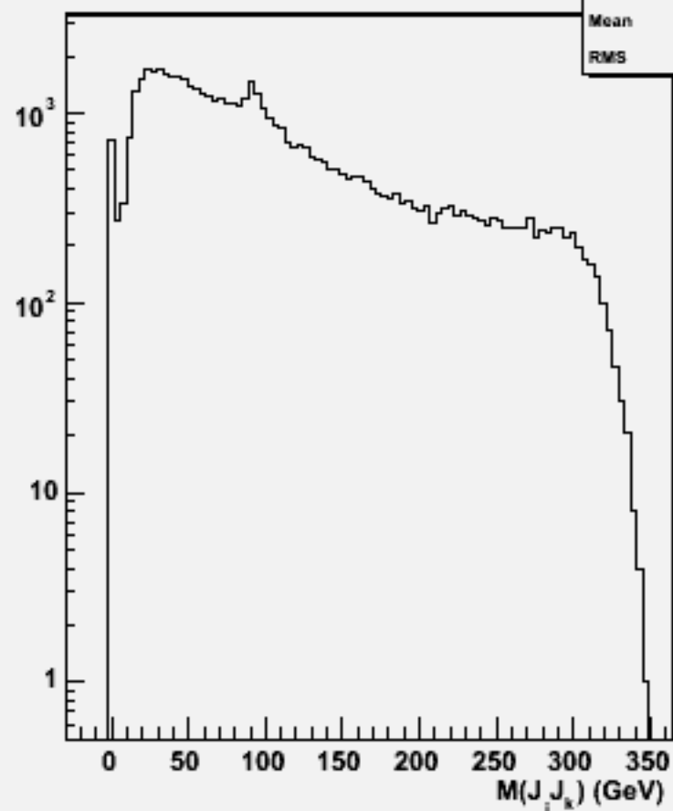
2jets mass(All comb)w103400 e1a_e1e3e3dd_o
