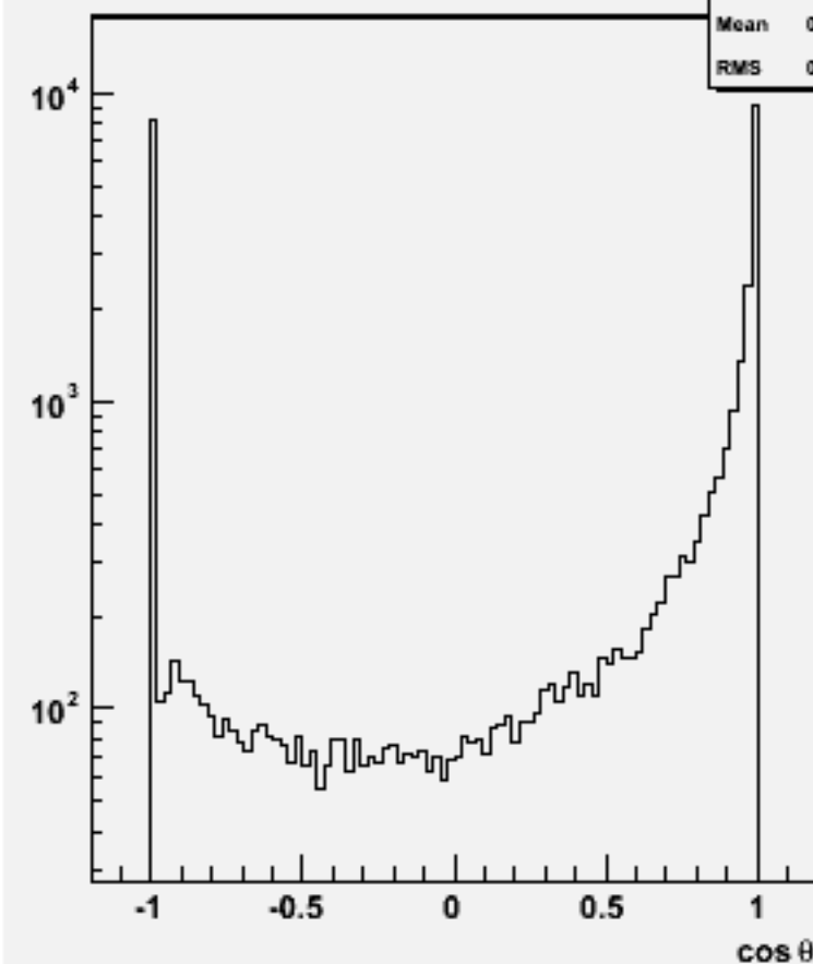
Jet cos \theta (All jets)w103399 e1a_e1e3e3dd_o
