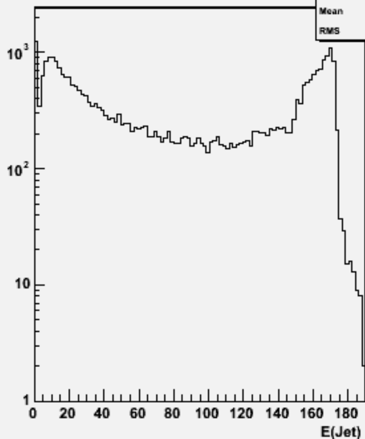
Jet energies(All jets)w103399 e1a_e1e3e3dd_o
