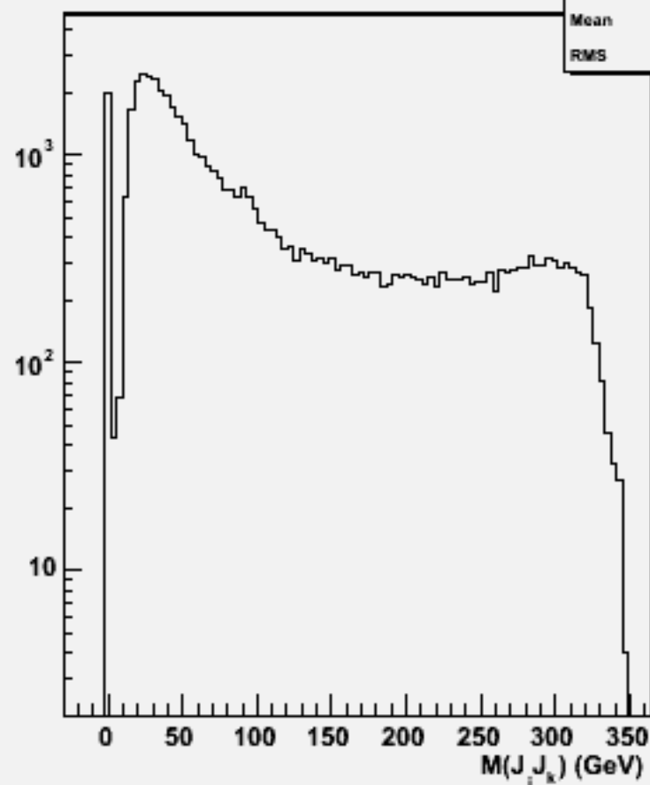
2jets mass(All comb)w103399 e1a_e1e3e3dd_o
