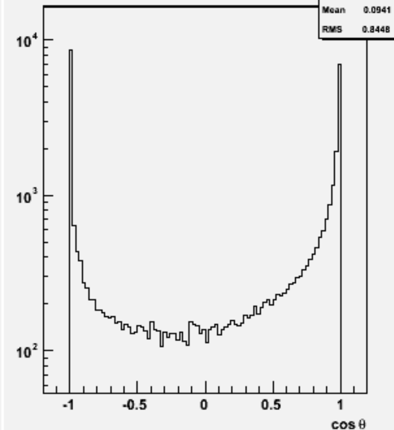
Jet cos theta (All jets)w103398 e1a_e1e3e3dd_o
