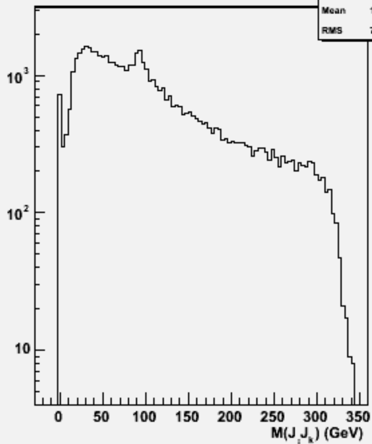
2jets mass(All comb)w103398 e1a_e1e3e3dd_o
