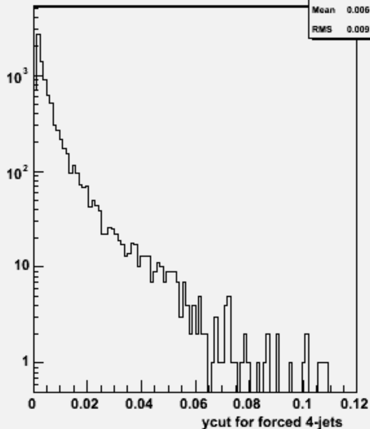
Ycut for 4-jets :w103398 e1a_e1e3e3dd_o
