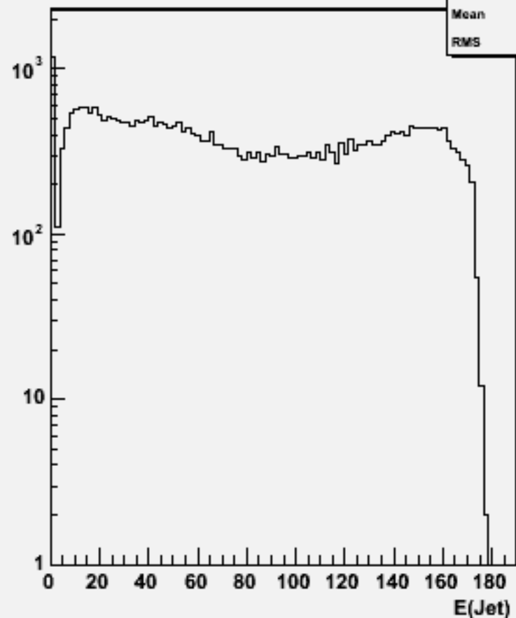
Jet energies(All jets)w103398 e1a_e1e3e3dd_o
