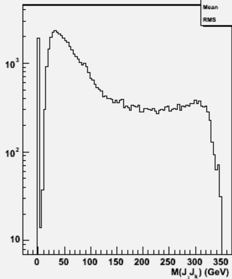
2jets mass(All comb)w103393 e1a_e1e2e2bb_o
