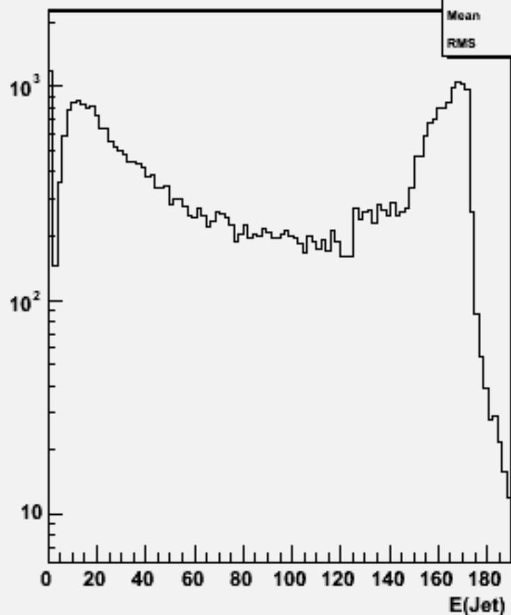
Jet energies(All jets)w103393 e1a_e1e2e2bb_o
