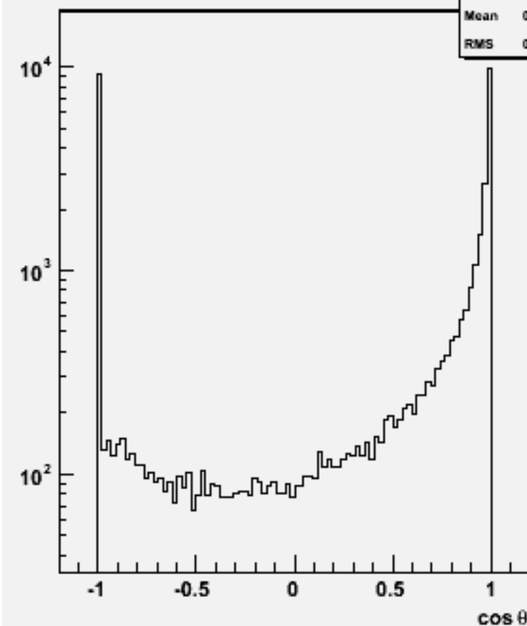
Jet cos \theta (All jets)w103393 e1a_e1e2e2bb_o
