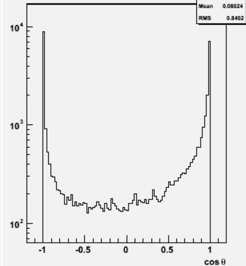
Jet cos theta (All jets)w103392 e1a_e1e2e2bb_o
