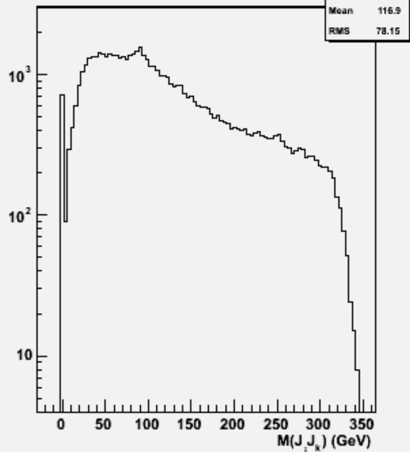
2jets mass(All comb)w103392 e1a_e1e2e2bb_o
