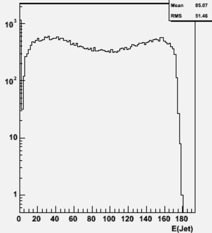
Jet energies(All jets)w103392 e1a_e1e2e2bb_o
