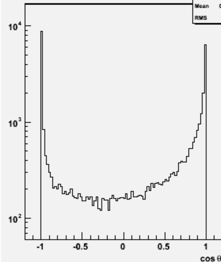
Jet cos \theta (All jets)w103390 e1a_e1e2e2bb_o
