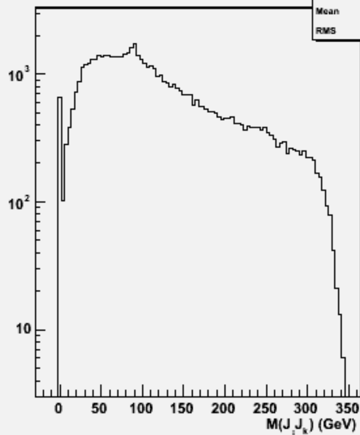
2jets mass(All comb)w103390 e1a_e1e2e2bb_o
