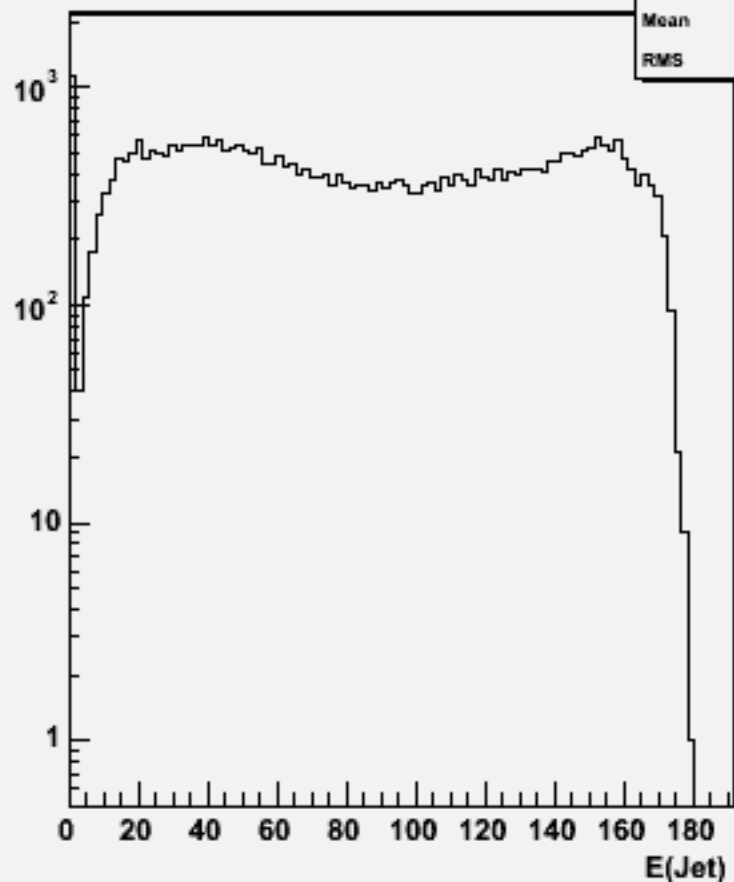
Jet energies(All jets)w103390 e1a_e1e2e2bb_o
