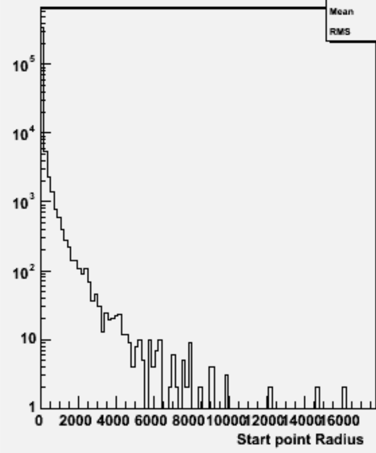
Start point R : w103388 e1a_e1e2e2ss_o
