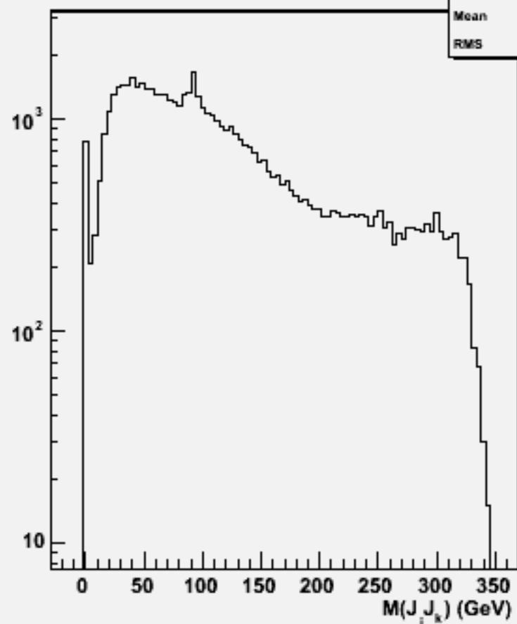
2jets mass(All comb)w103388 e1a_e1e2e2ss_o
