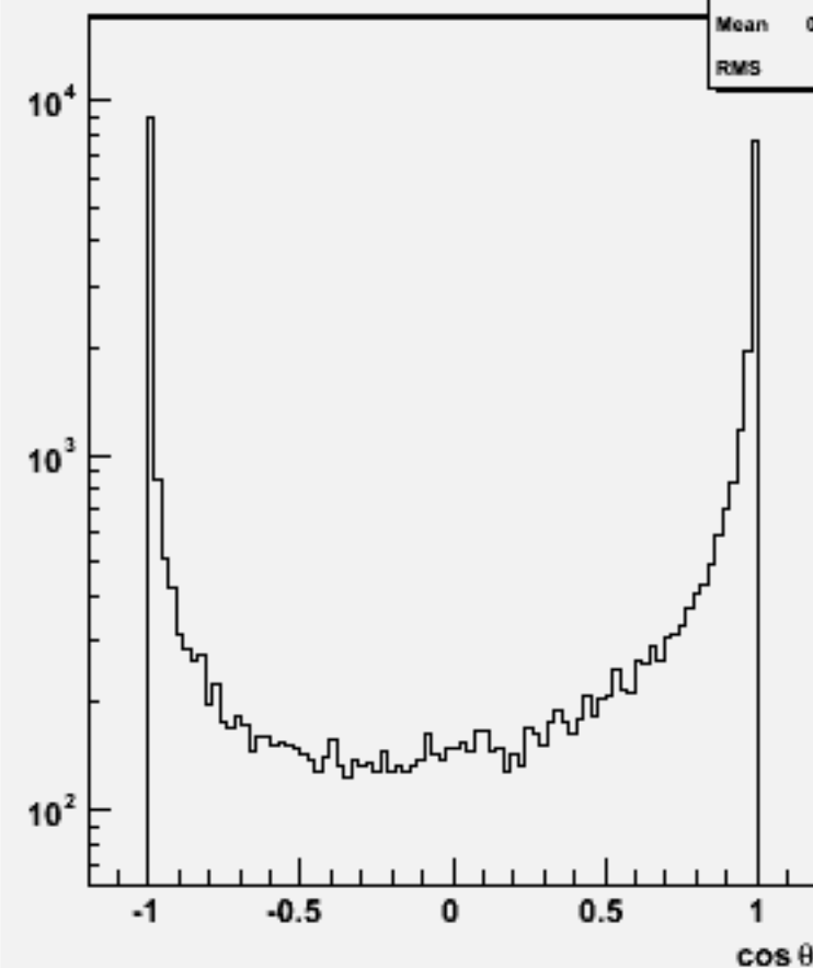
Jet cos \theta (All jets)w103388 e1a_e1e2e2ss_o
