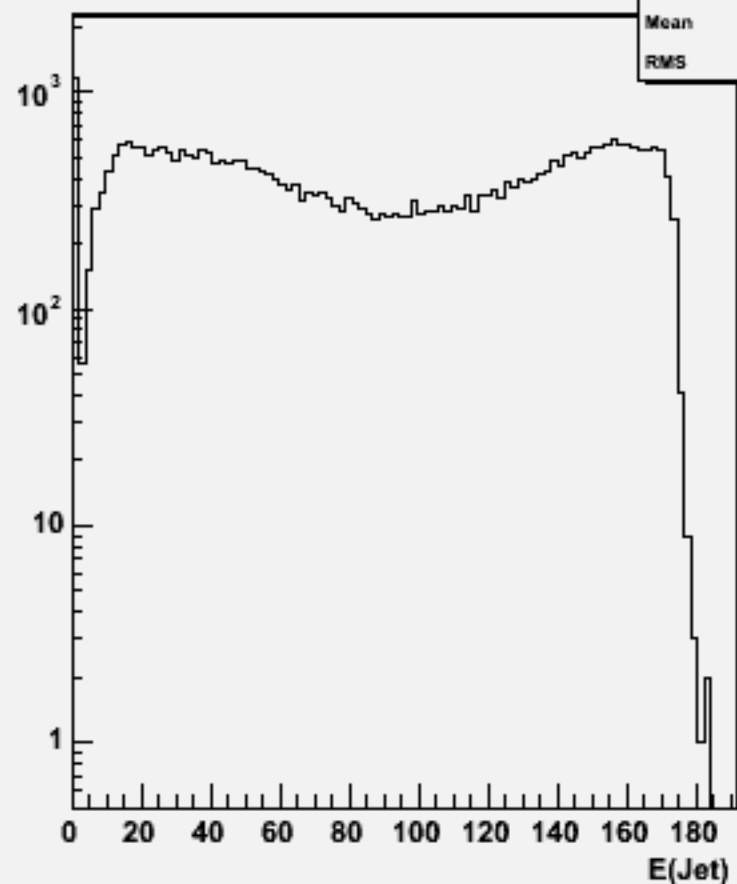
Jet energies(All jets)w103388 e1a_e1e2e2ss_o
