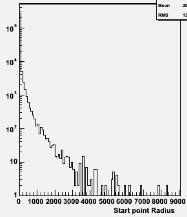
Start point R : w103387 e1a_e1e2e2ss_o
