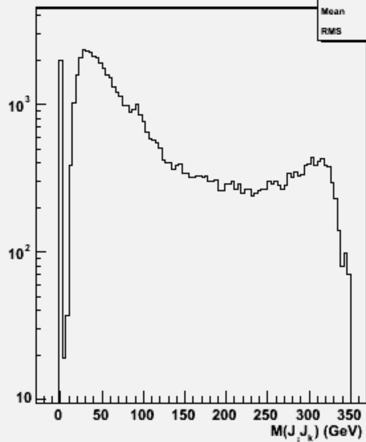
2jets mass(All comb)w103387 e1a_e1e2e2ss_o
