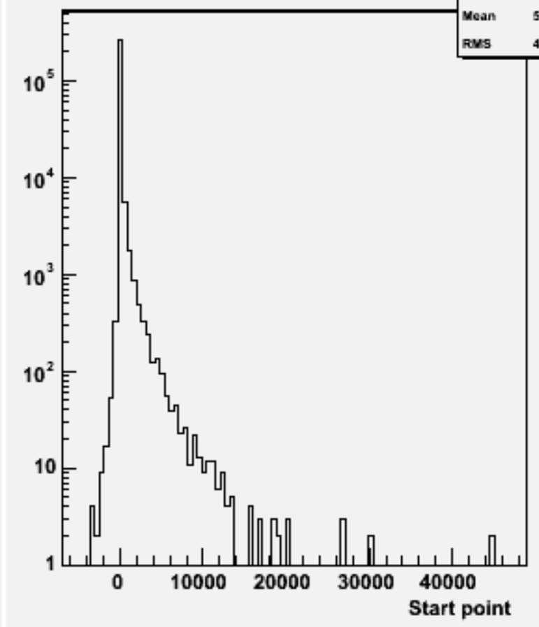
Start point Z : w103387 e1a_e1e2e2ss_o
