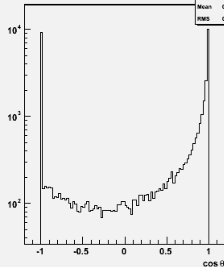
Jet cos \theta (All jets)w103387 e1a_e1e2e2ss_o
