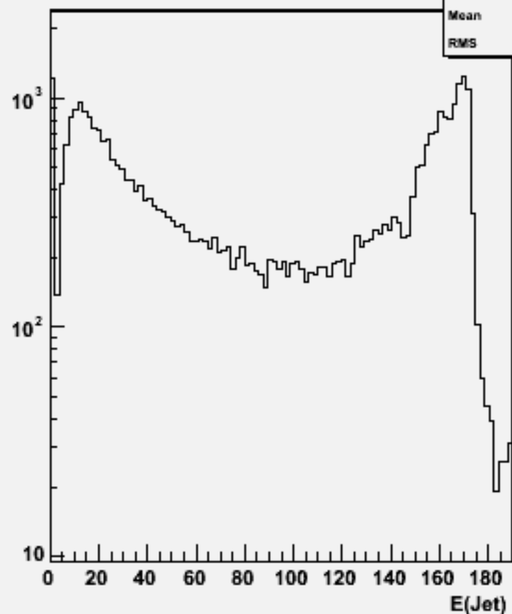
Jet energies(All jets)w103387 e1a_e1e2e2ss_o
