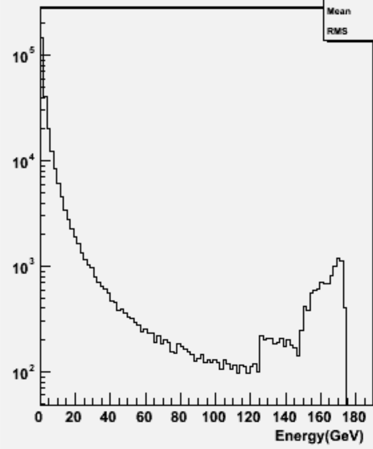
Start point R : w103387 e1a_e1e2e2ss_o
