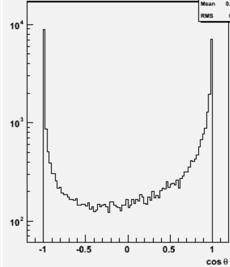
Jet cos \theta (All jets)w103386 e1a_e1e2e2ss_o
