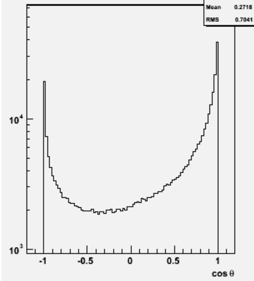
Particle cos θ : w103386 e1a_e1e2e2ss_o
