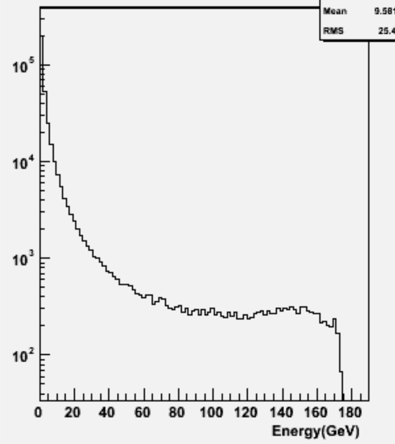
Start point R : w103386 e1a_e1e2e2ss_o
