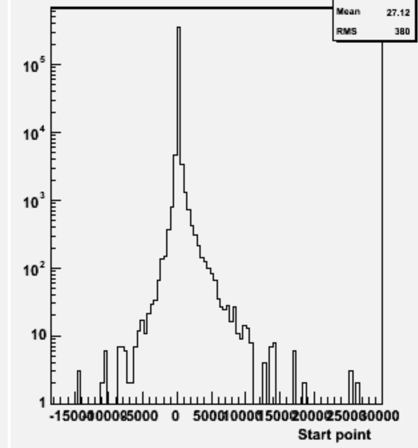
Start point Z : w103386 e1a_e1e2e2ss_o
