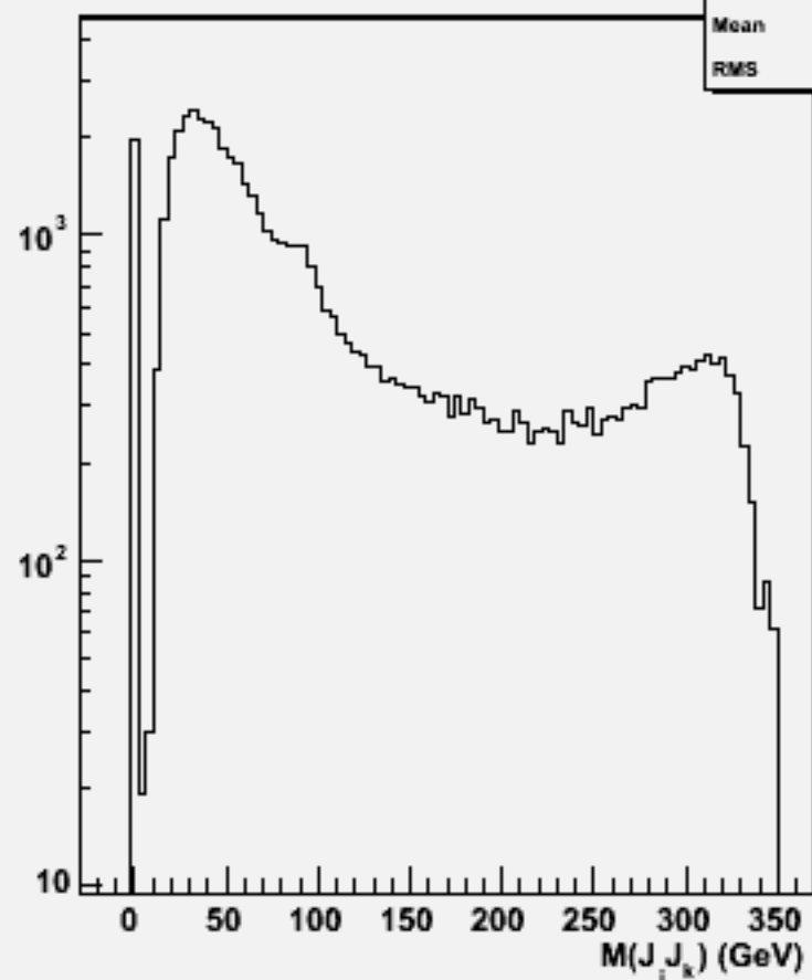
2jets mass(All comb)w103385 e1a_e1e2e2dd_o
