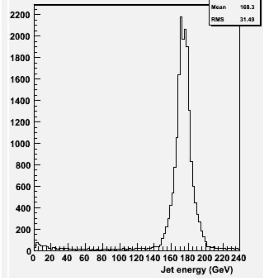
energy for 2-jets : w103385 e1a_e1e2e2dd_o
