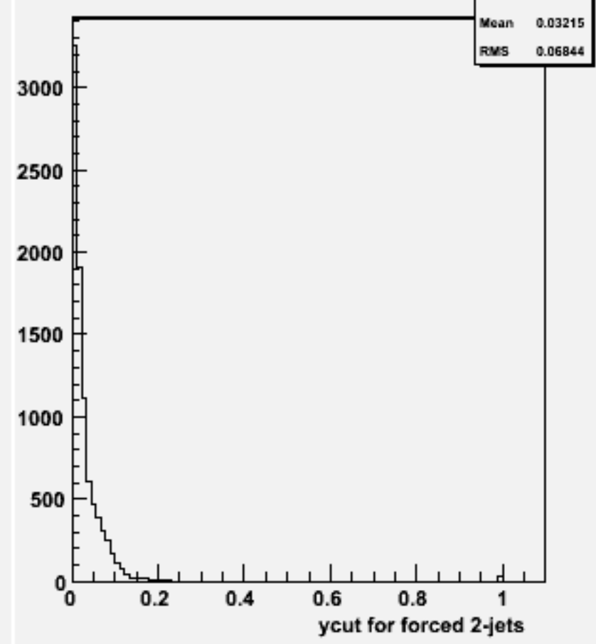
Ycut for 2-jets : w103385 e1a_e1e2e2dd_o
