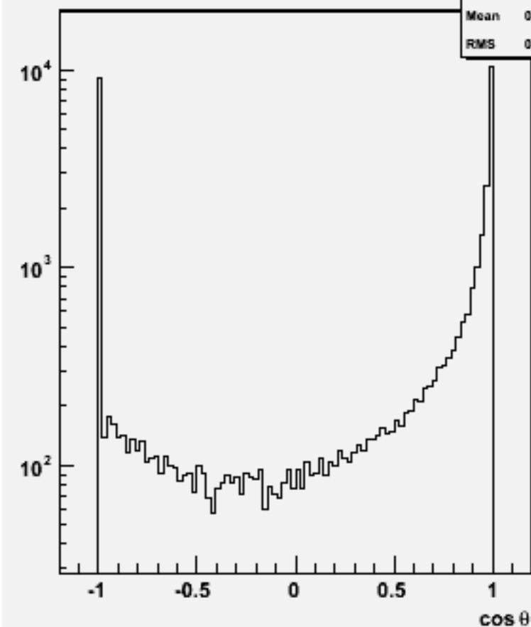
Jet cos \theta (All jets)w103385 e1a_e1e2e2dd_o
