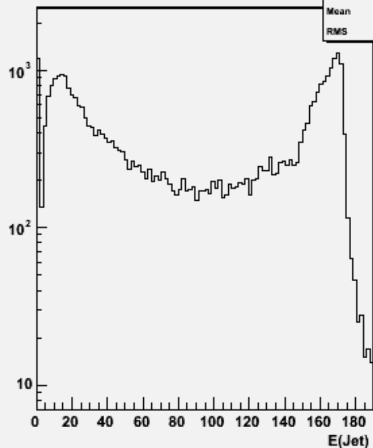
Jet energies(All jets)w103385 e1a_e1e2e2dd_o
