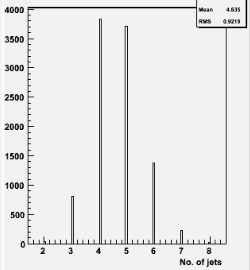
No. jets (ycut=0.001) : w103385 e1a_e1e2e2dd_o
