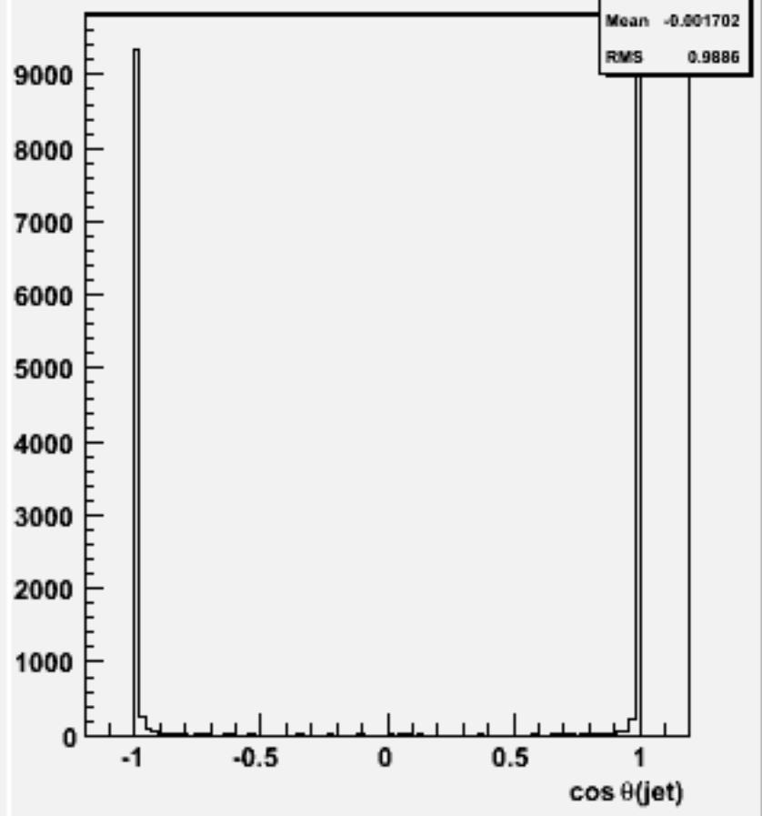
cos \theta for 2-jets : w103385 e1a_e1e2e2dd_o
