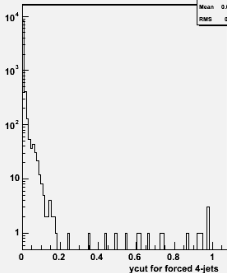
Ycut for 4-jets :w103385 e1a_e1e2e2dd_o
