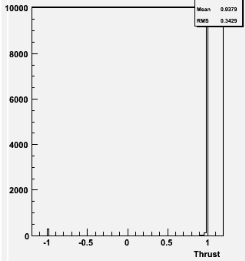
cos \Theta (thrust) w103385 e1a_e1e2e2dd_o
