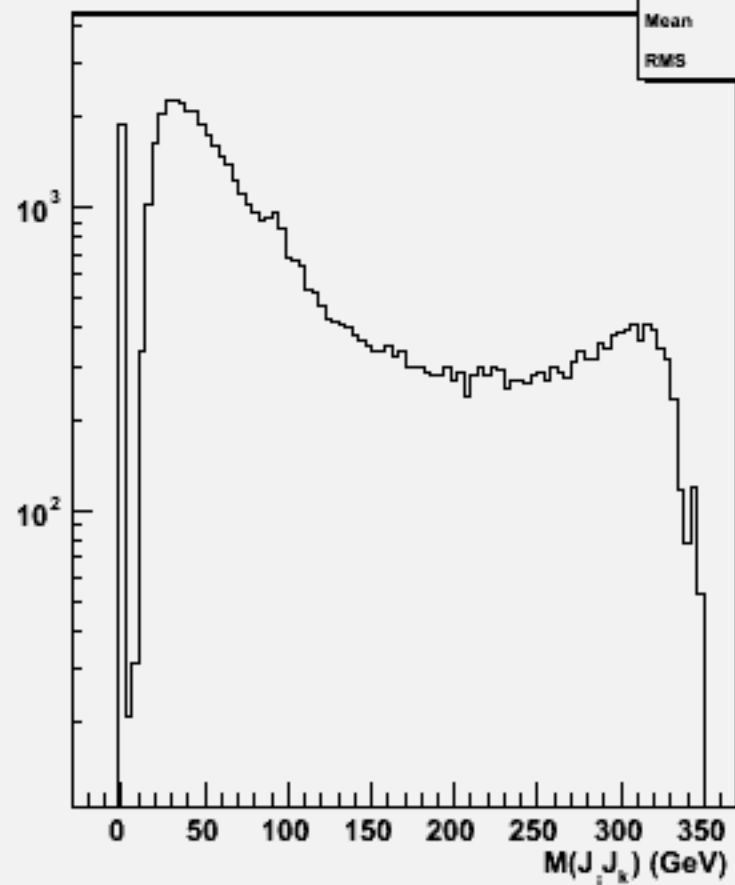
2jets mass(All comb)w103383 e1a_e1e2e2dd_o
