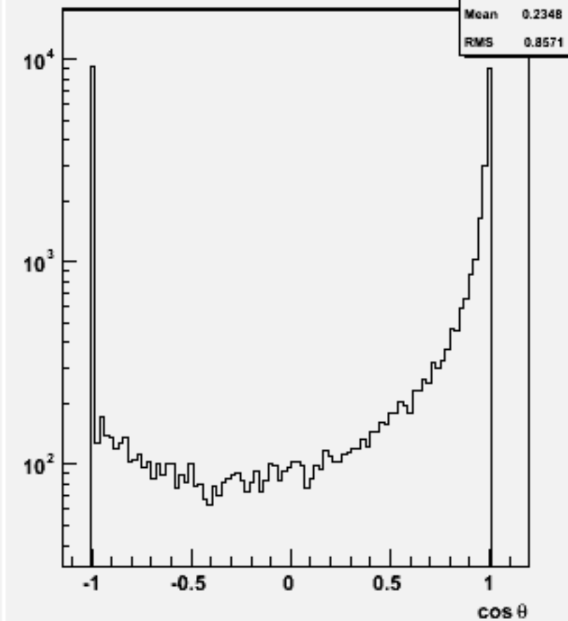
Jet cos \theta (All jets)w103383 e1a_e1e2e2dd_o
