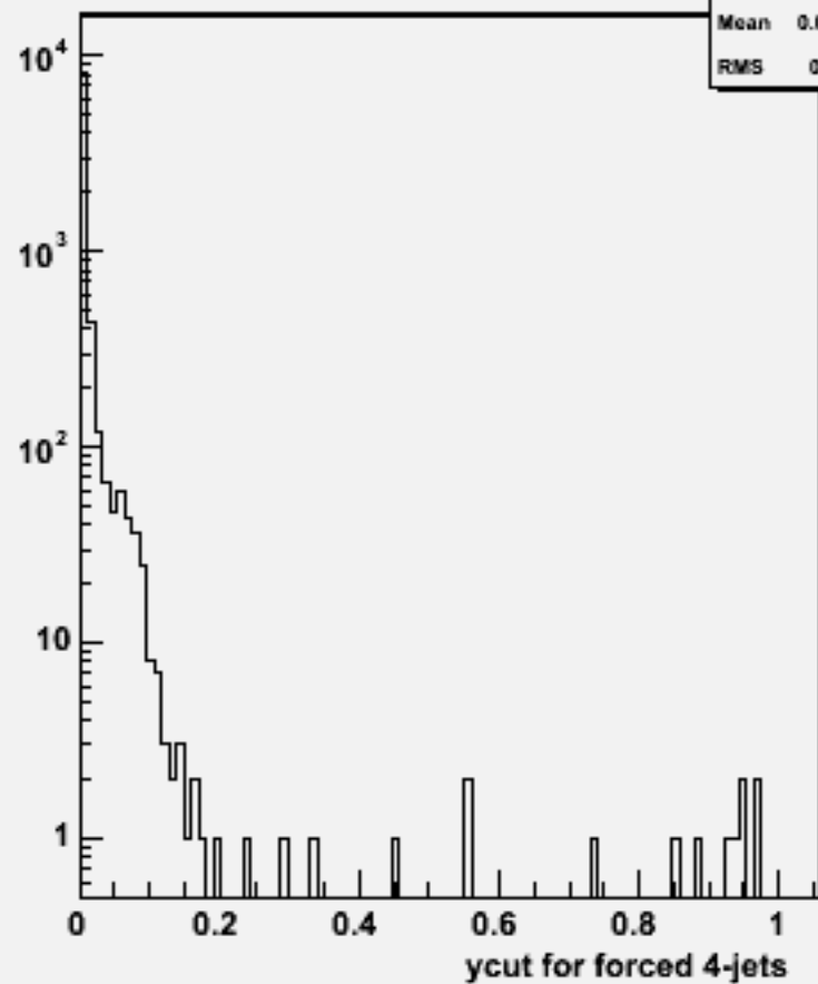
Ycut for 4-jets :w103383 e1a_e1e2e2dd_o
