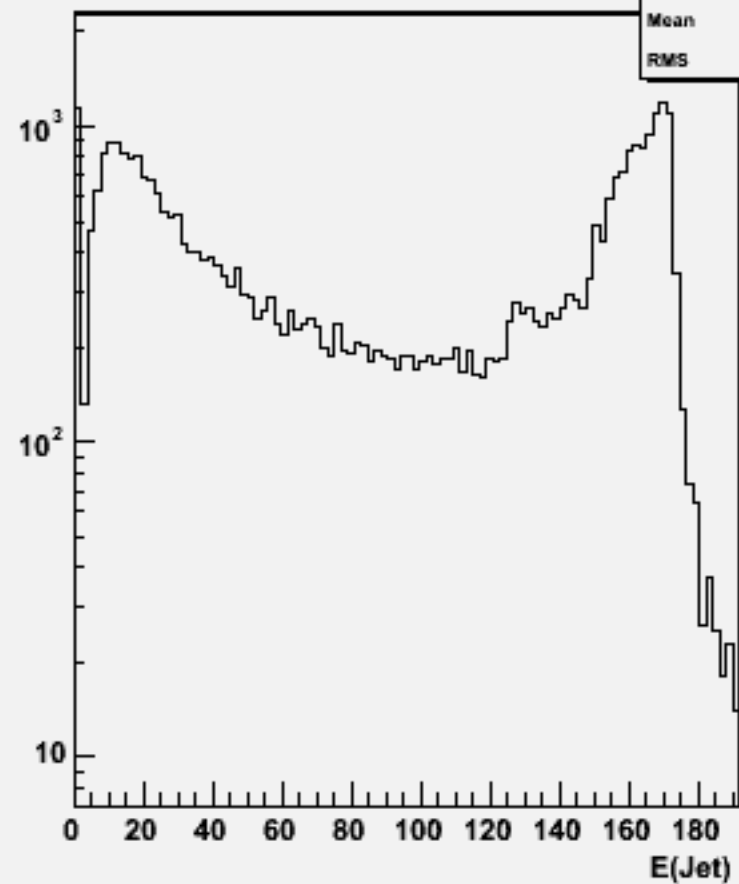
Jet energies(All jets)w103383 e1a_e1e2e2dd_o
