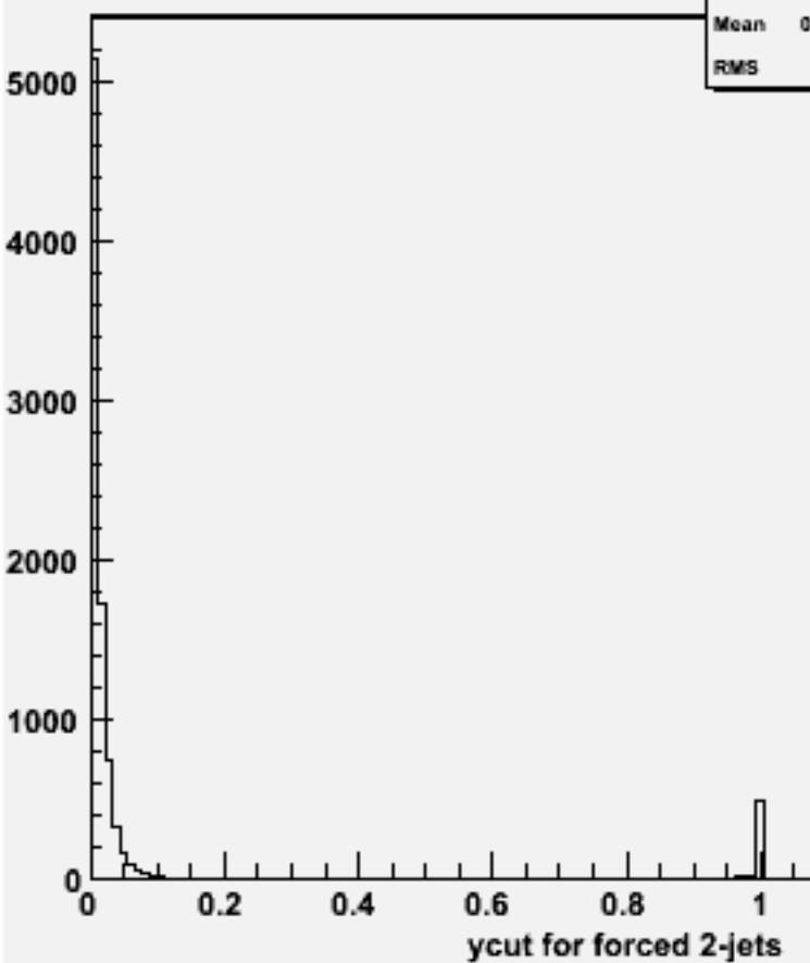
Ycut for 2-jets :w103381 e1a_e1e2e2e3e3_o
