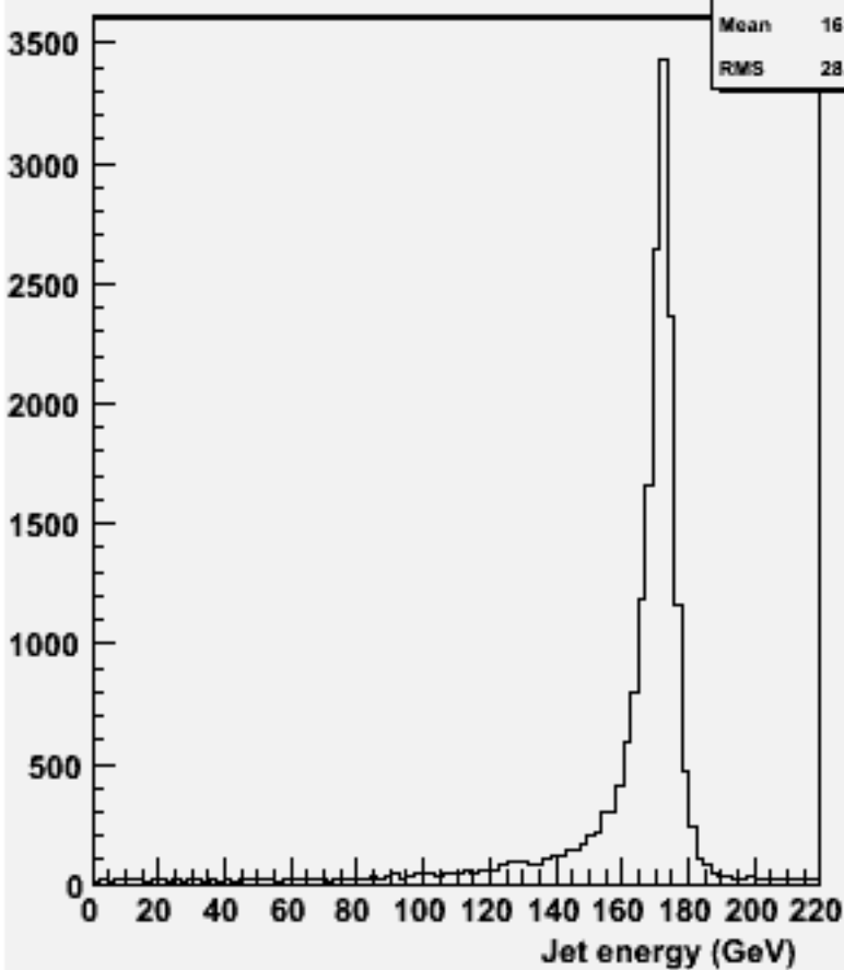
energy for 2-jets :w103381 e1a_e1e2e2e3e3_o
