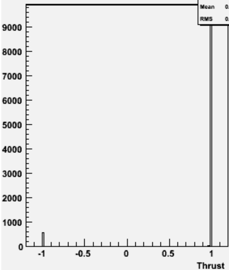
cos \Theta (thrust) w103381 e1a_e1e2e2e3e3_o
