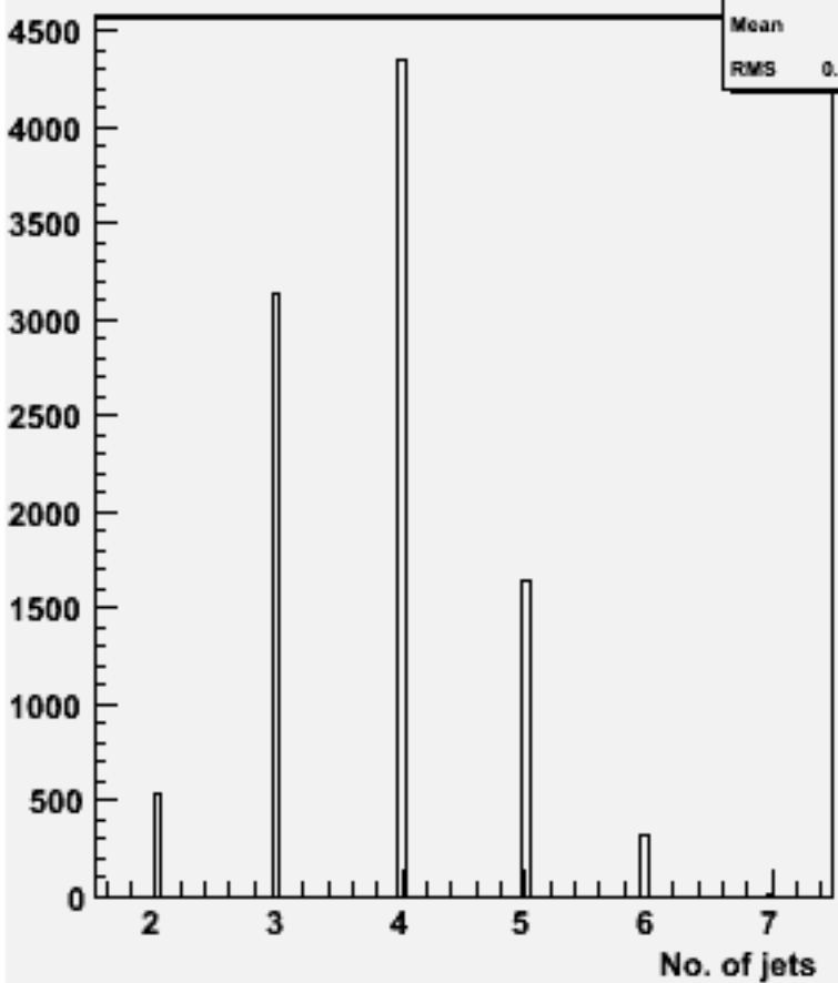
No. jets (ycut=0.001) : w103381 e1a_e1e2e2e3e3_o
