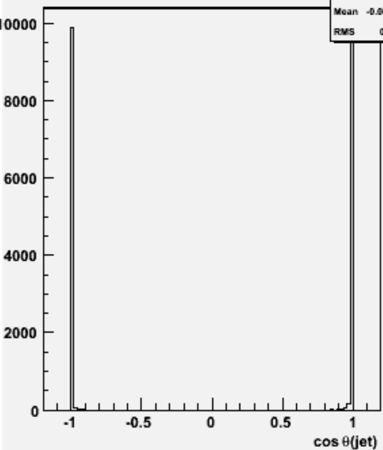
cos \Theta for 2-jets :w103381 e1a_e1e2e2e3e3_o
