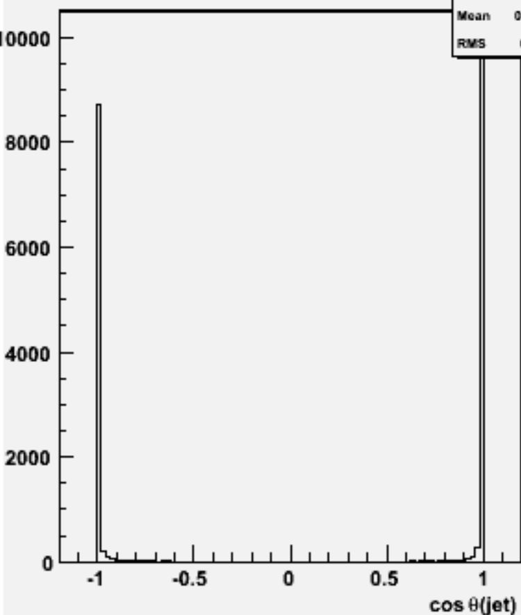
cos \Theta for 2-jets :w103378 e1a_e1e2e2e3e3_o
