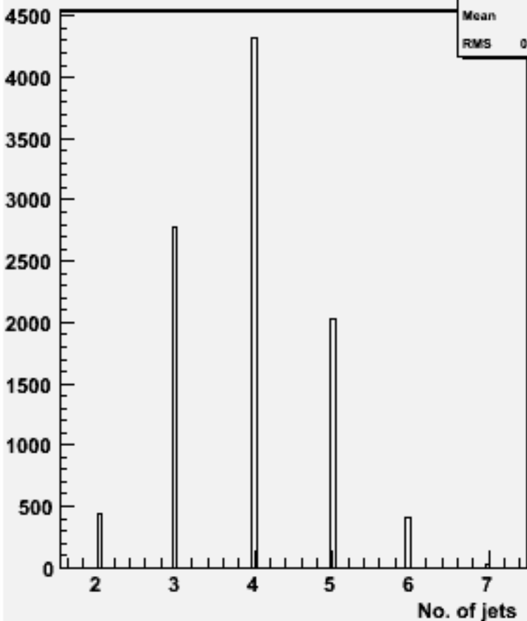
No. jets (ycut=0.001) : w103378 e1a_e1e2e2e3e3_o
