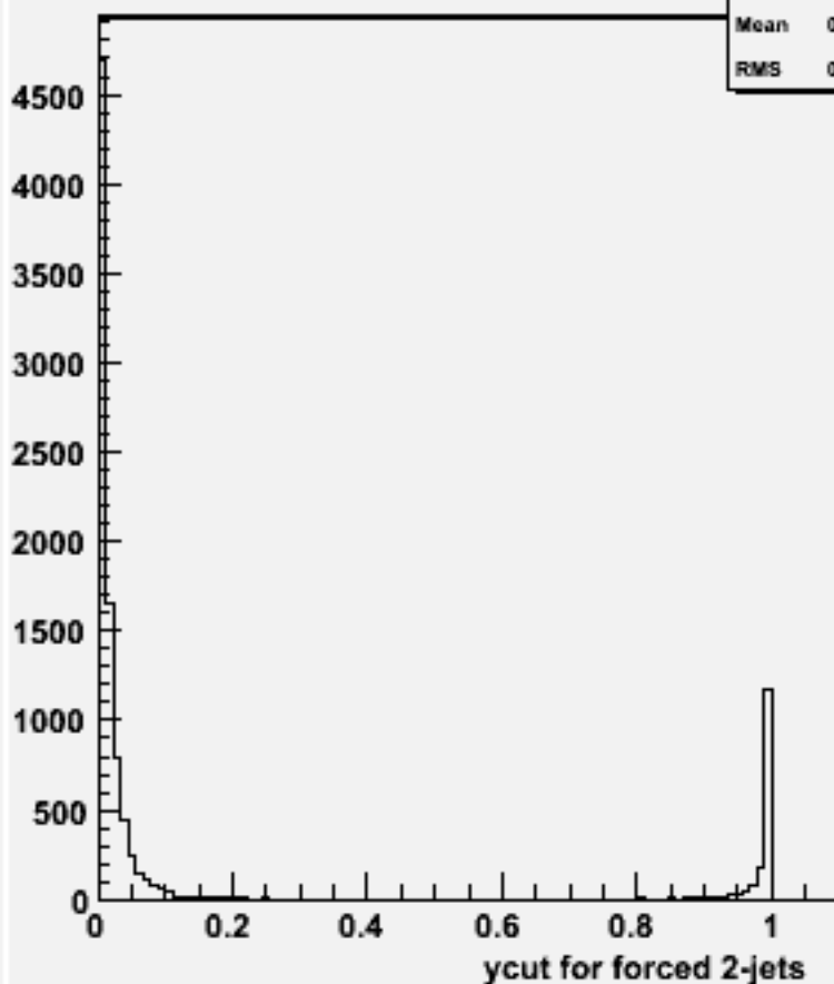
Ycut for 2-jets :w103378 e1a_e1e2e2e3e3_o
