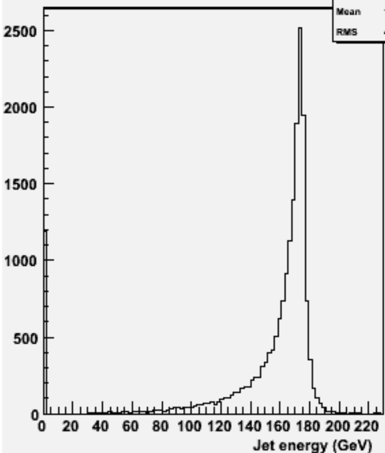
energy for 2-jets :w103378 e1a_e1e2e2e3e3_o
