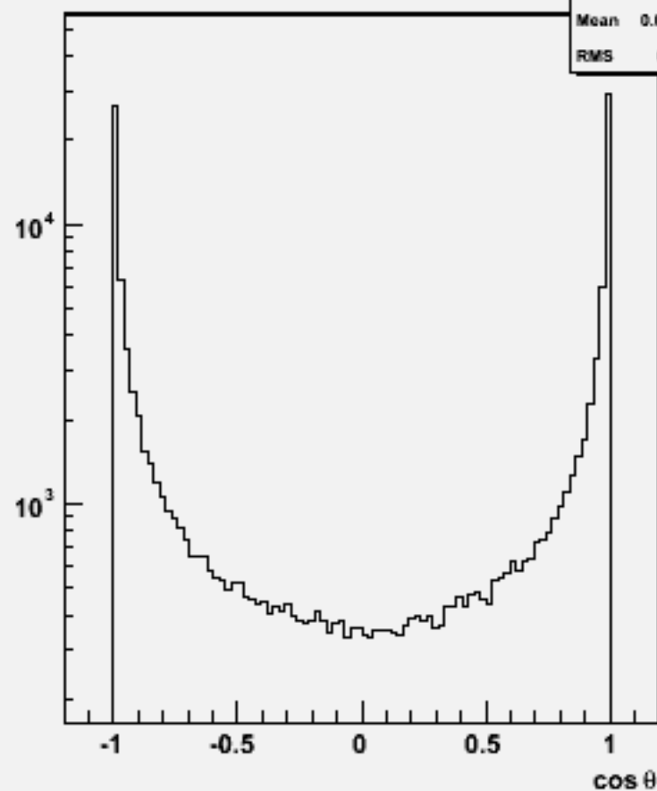
Particle cos \theta : w103378 e1a_e1e2e2e3e3_o
