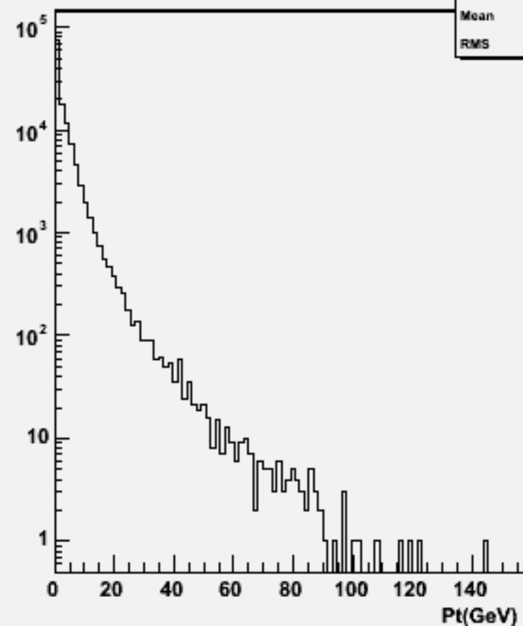
Particle Pt : w103378 e1a_e1e2e2e3e3_o
