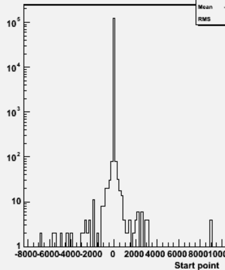
Start point Z : w103378 e1a_e1e2e2e3e3_o
