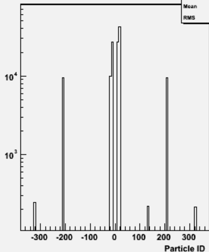
Particle ID : w103378 e1a_e1e2e2e3e3_o
