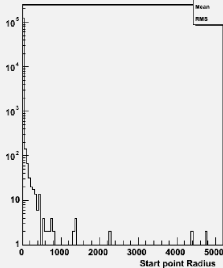
Start point R : w103378 e1a_e1e2e2e3e3_o
