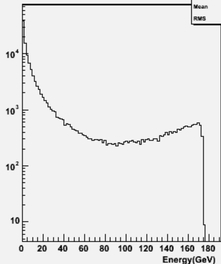
Particle Energy : w103378 e1a_e1e2e2e3e3_o
