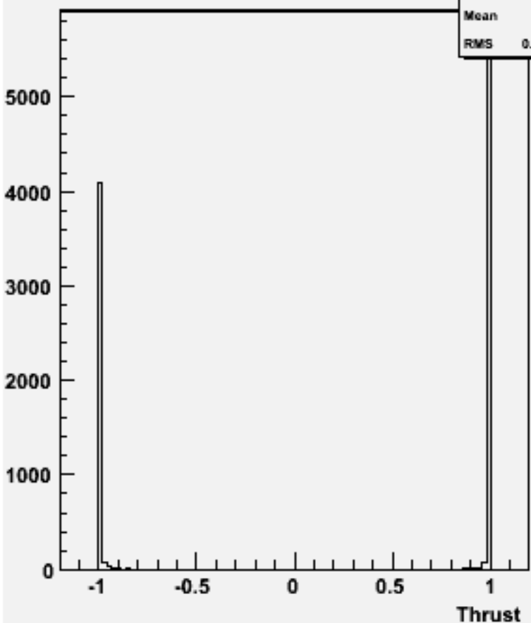
cos \Theta (thrust) w103378 e1a_e1e2e2e3e3_o
