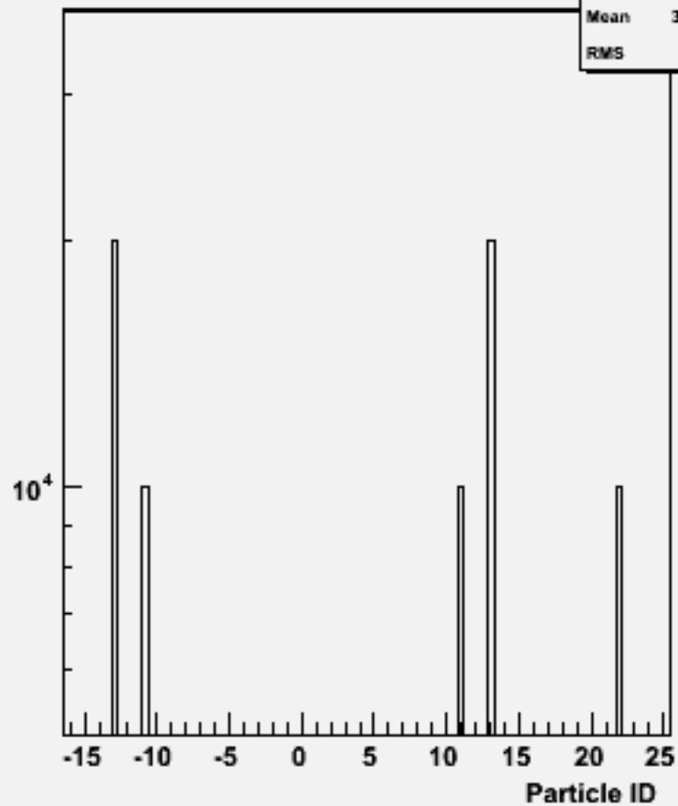
Particle ID : w103375 e1a_e1e2e2e2_o
