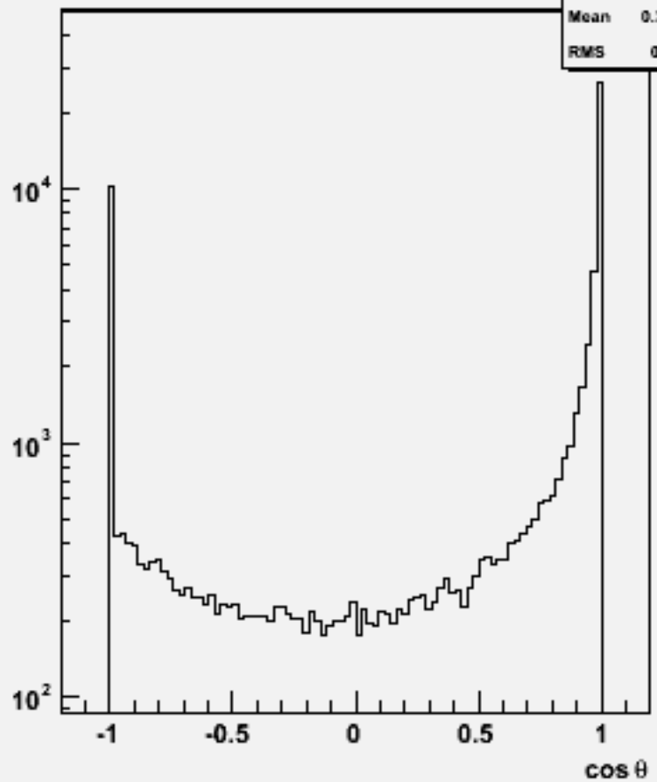
Particle cos \theta : w103375 e1a_e1e2e2e2_o
