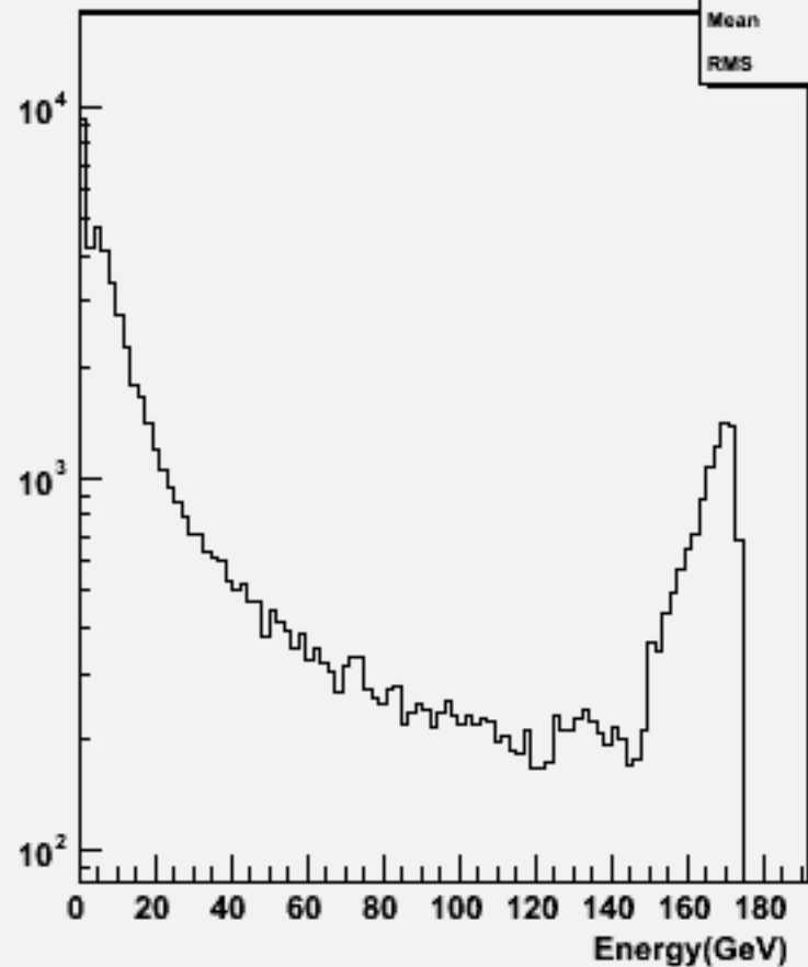
Particle Energy : w103375 e1a_e1e2e2e2_o
