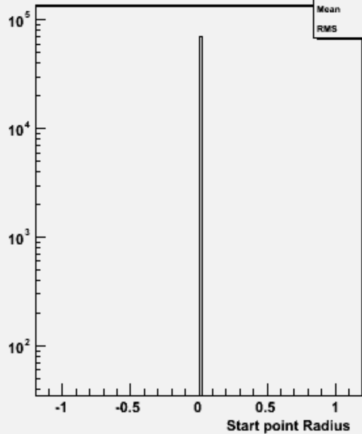
Start point R : w103375 e1a_e1e2e2e2_o
