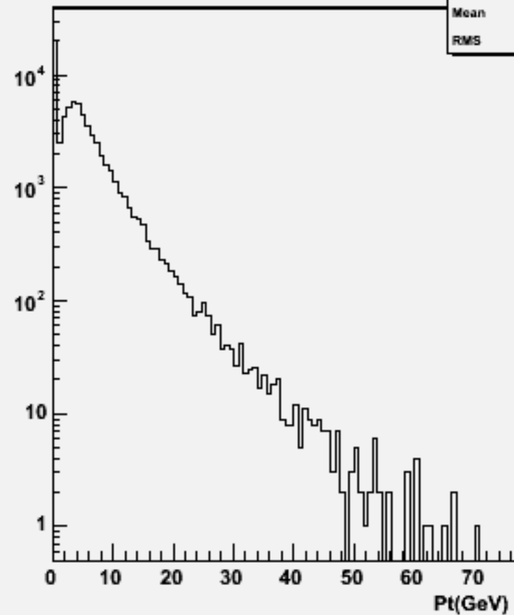
Particle Pt : w103375 e1a_e1e2e2e2_o
