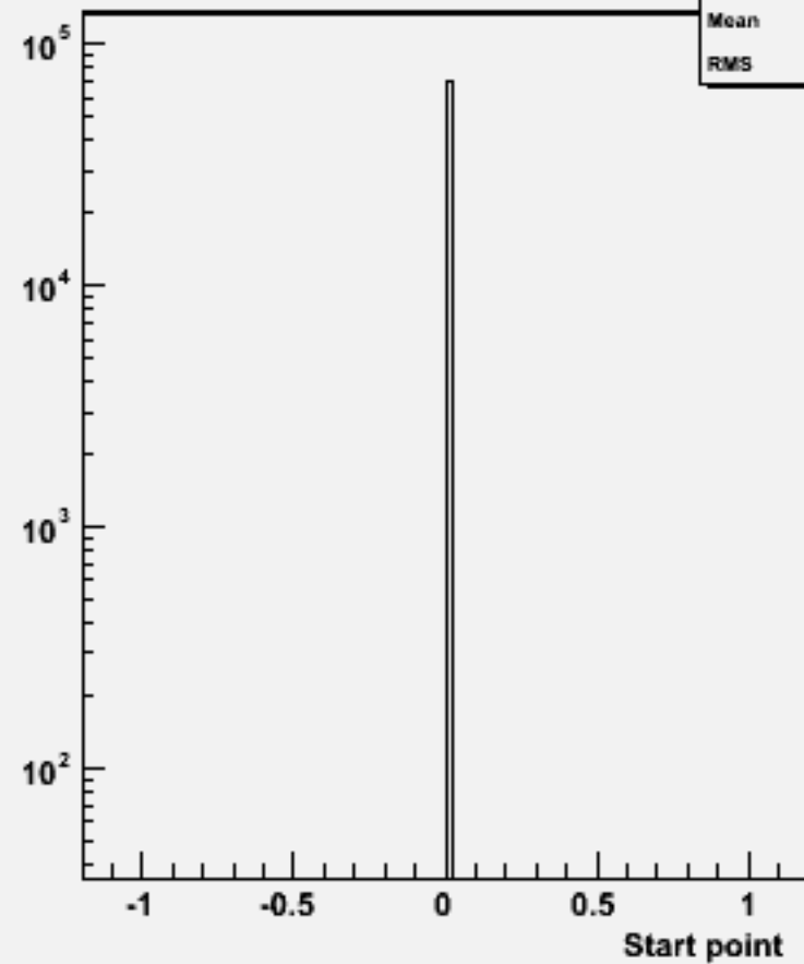
Start point Z : w103375 e1a_e1e2e2e2_o
