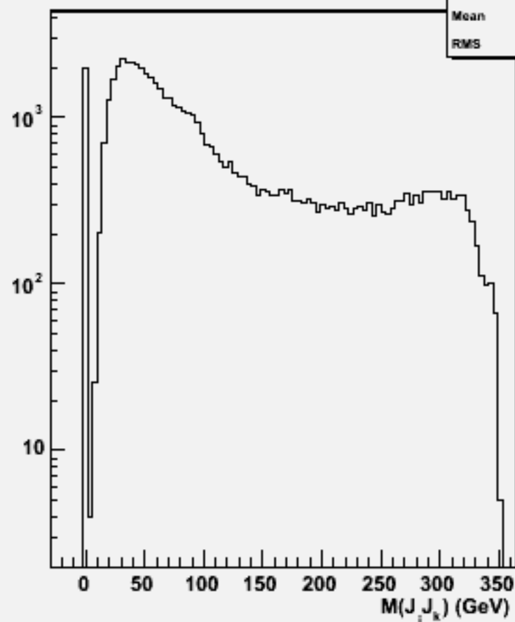
2jets mass(All comb)w103371 e1a_e1e1e1bb_o
