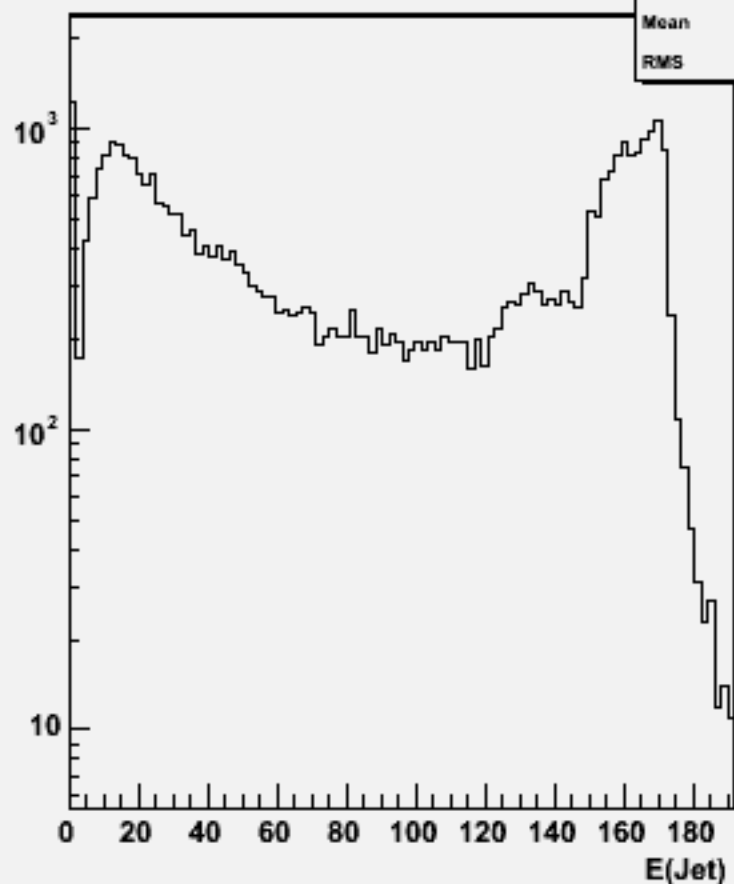
Jet energies(All jets)w103371 e1a_e1e1e1bb_o
