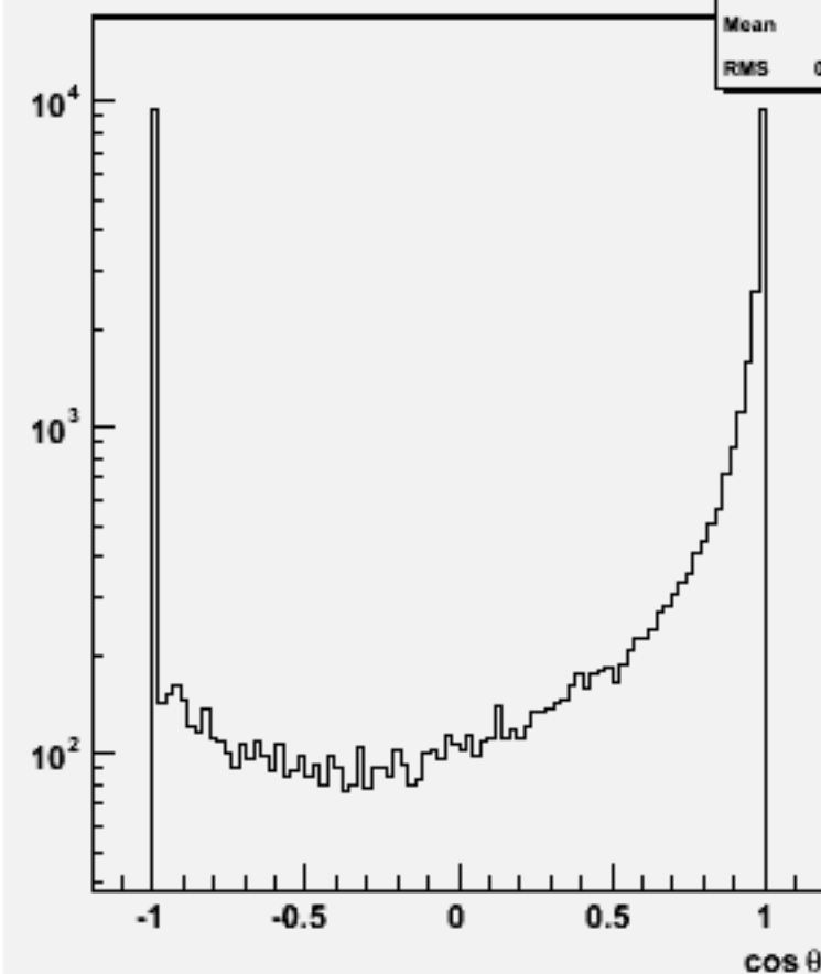
Jet cos \theta (All jets)w103371 e1a_e1e1e1bb_o
