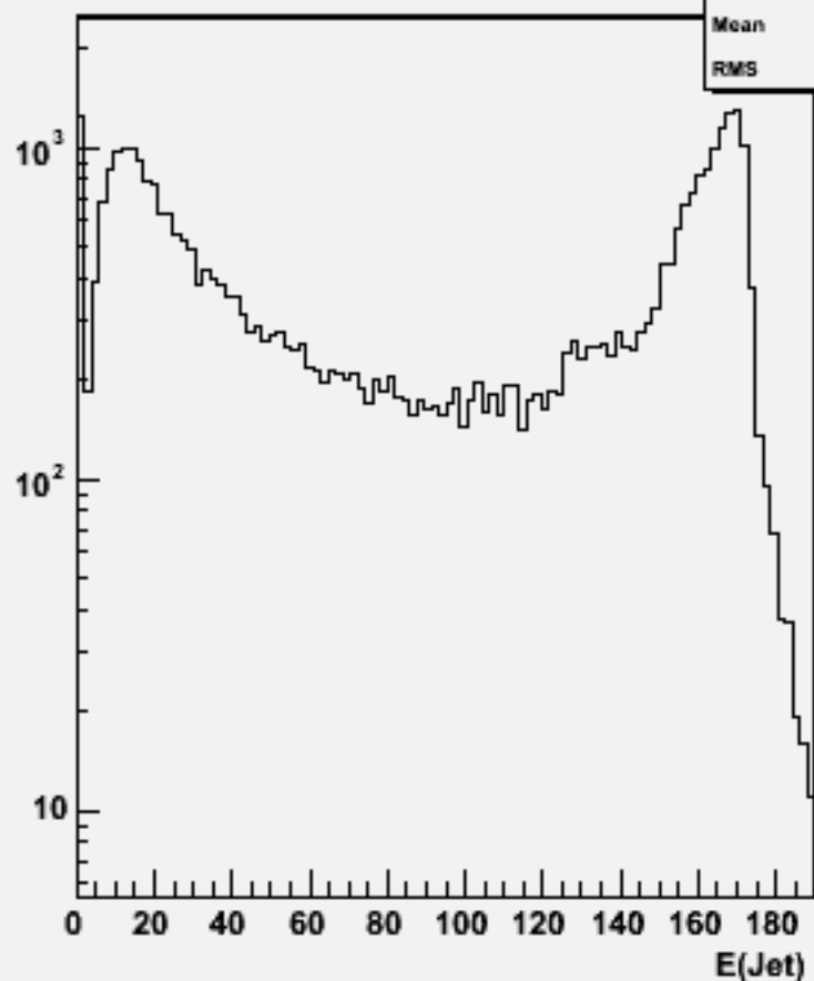
Jet energies(All jets)w103369 e1a_e1e1e1ss_o
