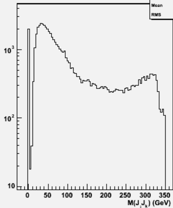
2jets mass(All comb)w103369 e1a_e1e1e1ss_o
