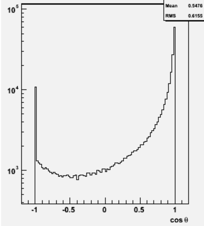
Particle cos \theta : w103369 e1a_e1e1e1ss_o
