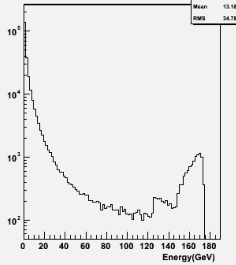
Start point R : w103369 e1a_e1e1e1ss_o
