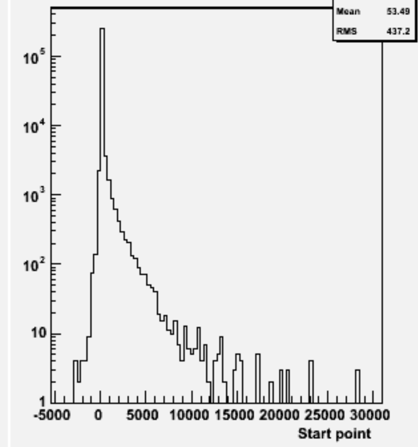
Start point Z : w103369 e1a_e1e1e1ss_o
