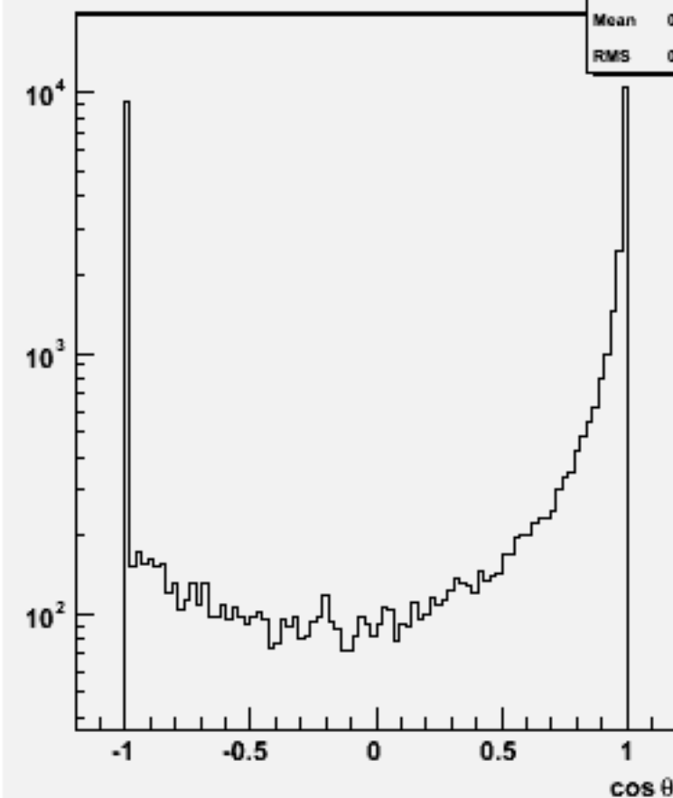
Jet cos \theta (All jets)w103369 e1a_e1e1e1ss_o
