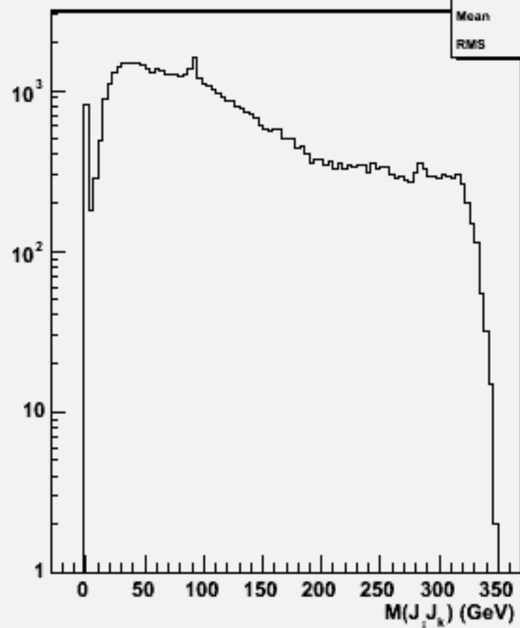
2jets mass(All comb)w103368 e1a_e1e1e1ss_o
