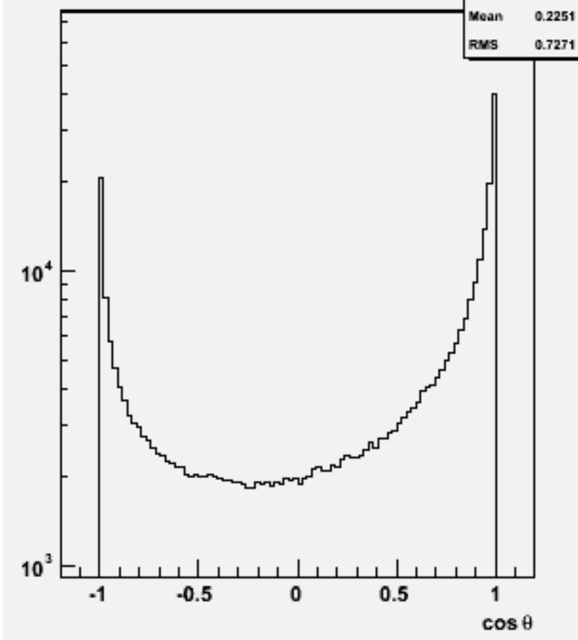
Particle cos \theta : w103368 e1a_e1e1e1ss_o
