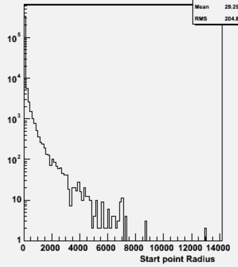
Start point R : w103368 e1a_e1e1e1ss_o
