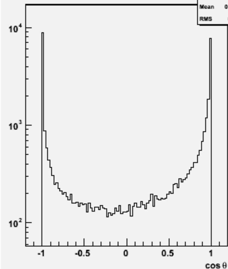
Jet cos \theta (All jets)w103368 e1a_e1e1e1ss_o
