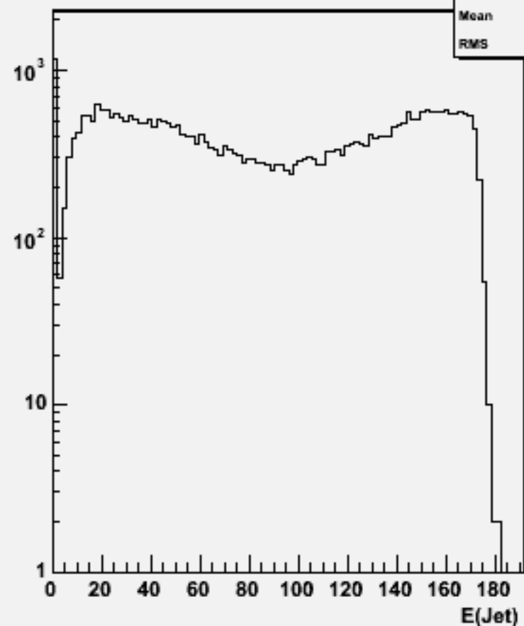
Jet energies(All jets)w103368 e1a_e1e1e1ss_o
