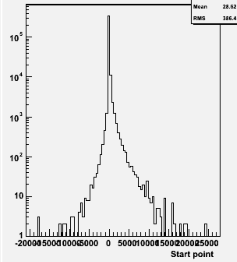
Start point Z : w103366 e1a_e1e1e1ss_o
