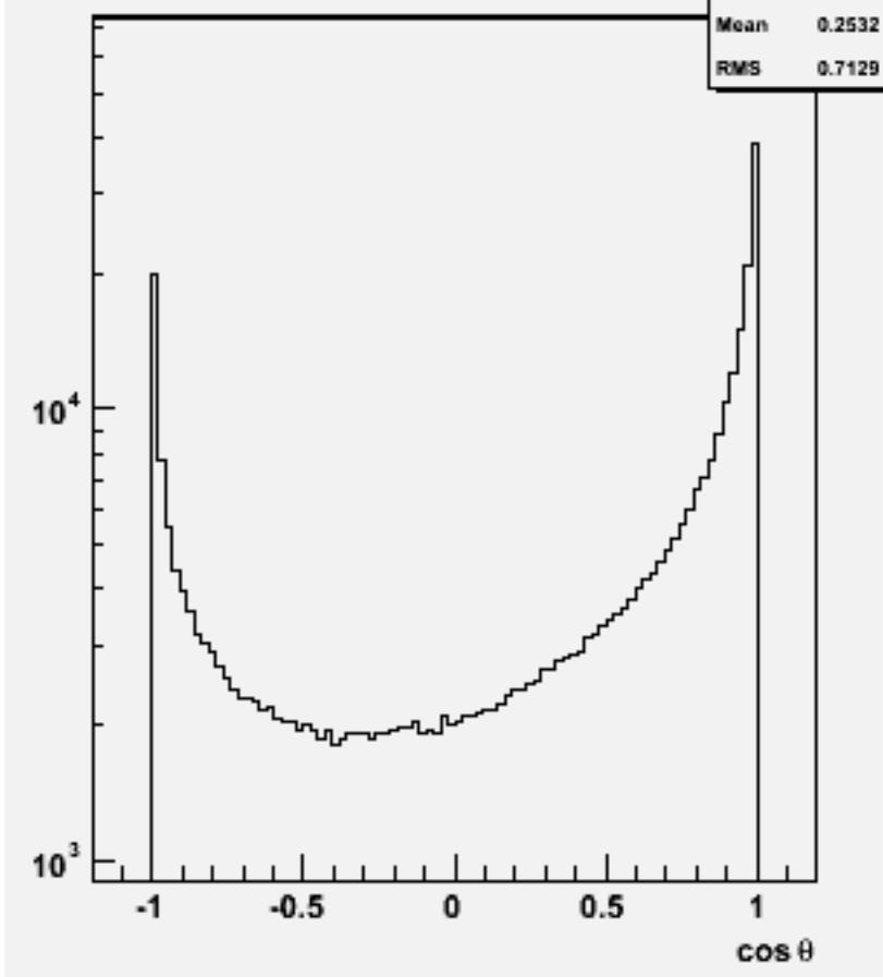
Particle cos \theta : w103366 e1a_e1e1e1ss_o
