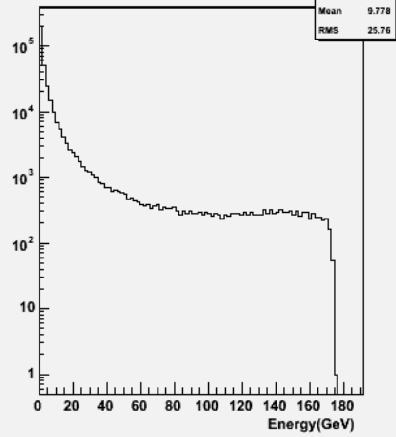
Start point R : w103366 e1a_e1e1e1ss_o
