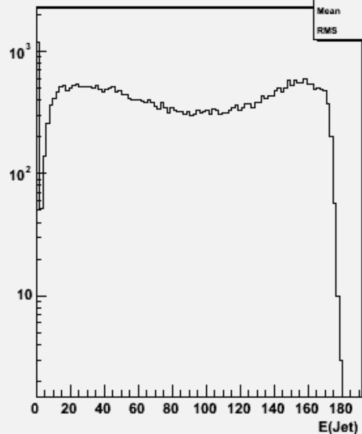
Jet energies(All jets)w103366 e1a_e1e1e1ss_o
