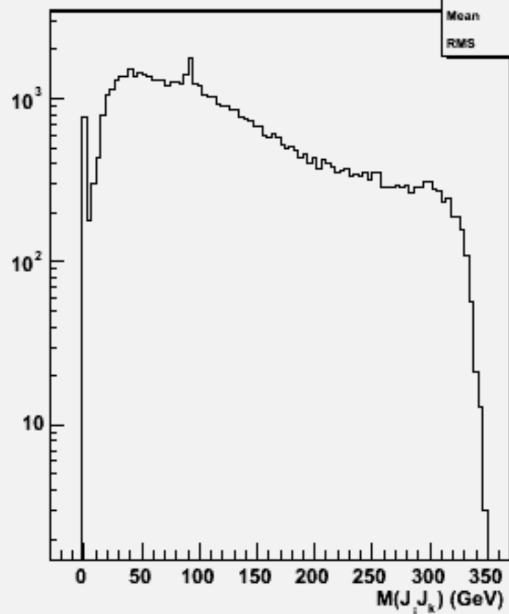
2jets mass(All comb)w103366 e1a_e1e1e1ss_o
