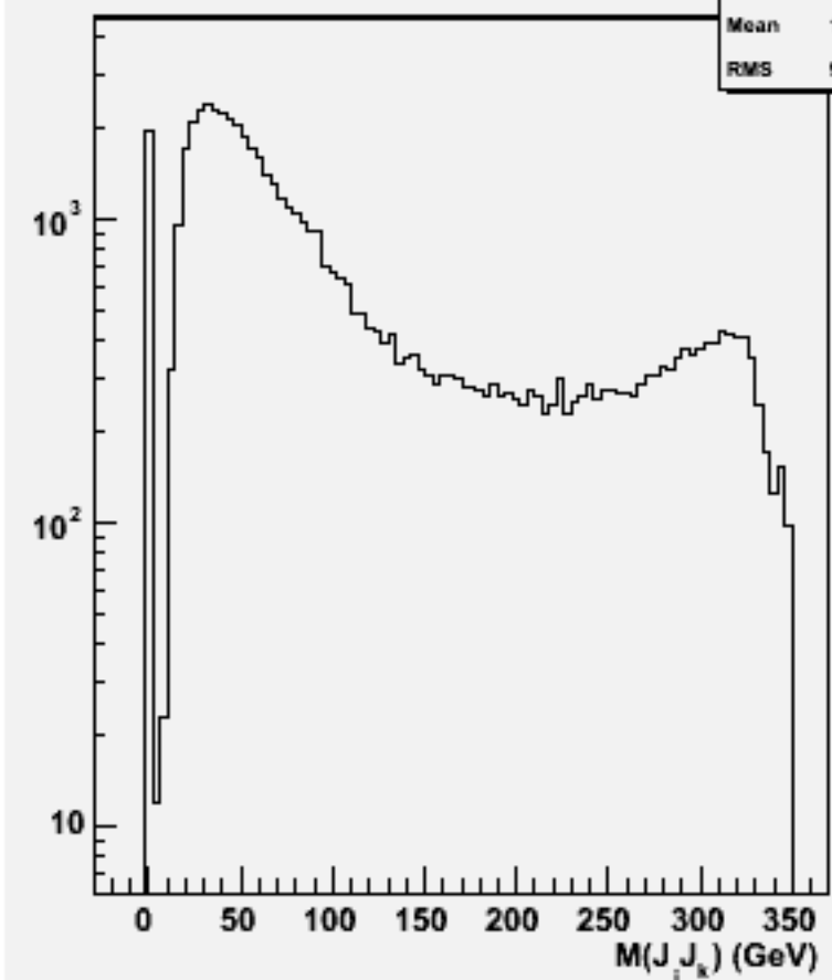
2jets mass(All comb)w103365 e1a_e1e1e1dd_o
