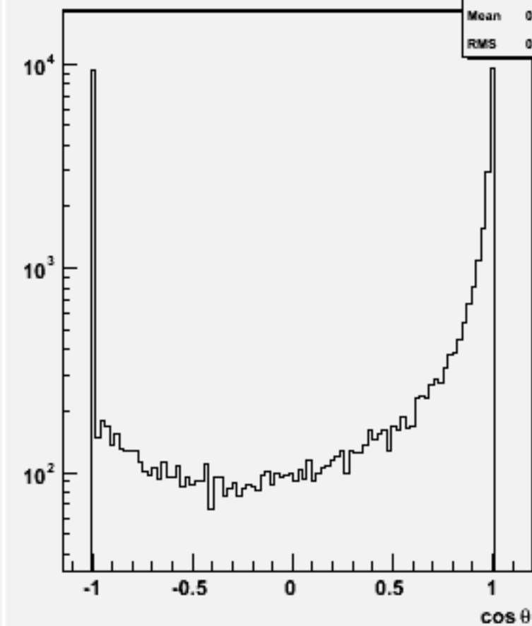
Jet cos \theta (All jets)w103365 e1a_e1e1e1dd_o
