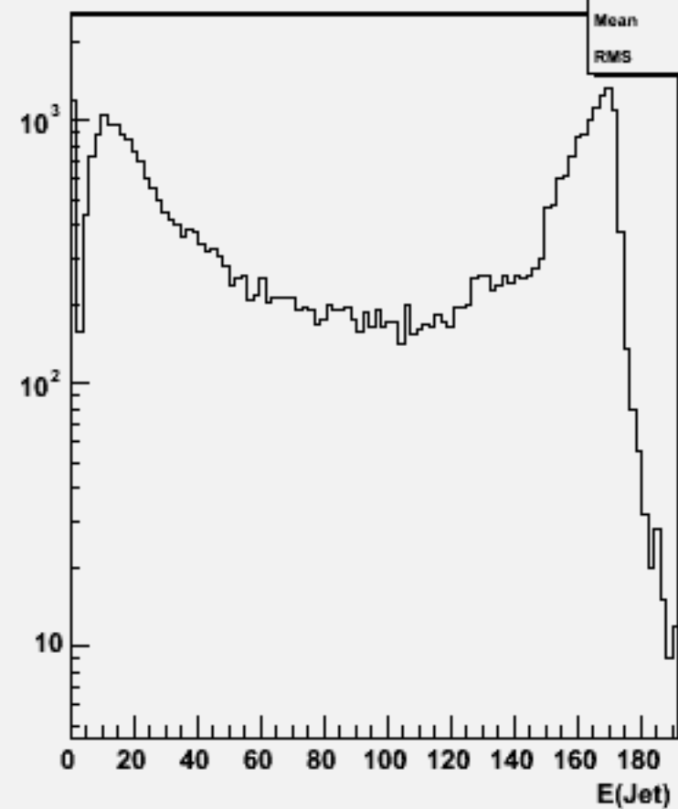
Jet energies(All jets)w103365 e1a_e1e1e1dd_o
