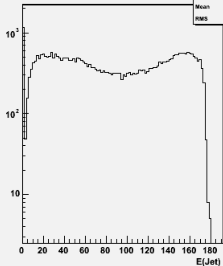
Jet energies(All jets)w103362 e1a_e1e1e1dd_o
