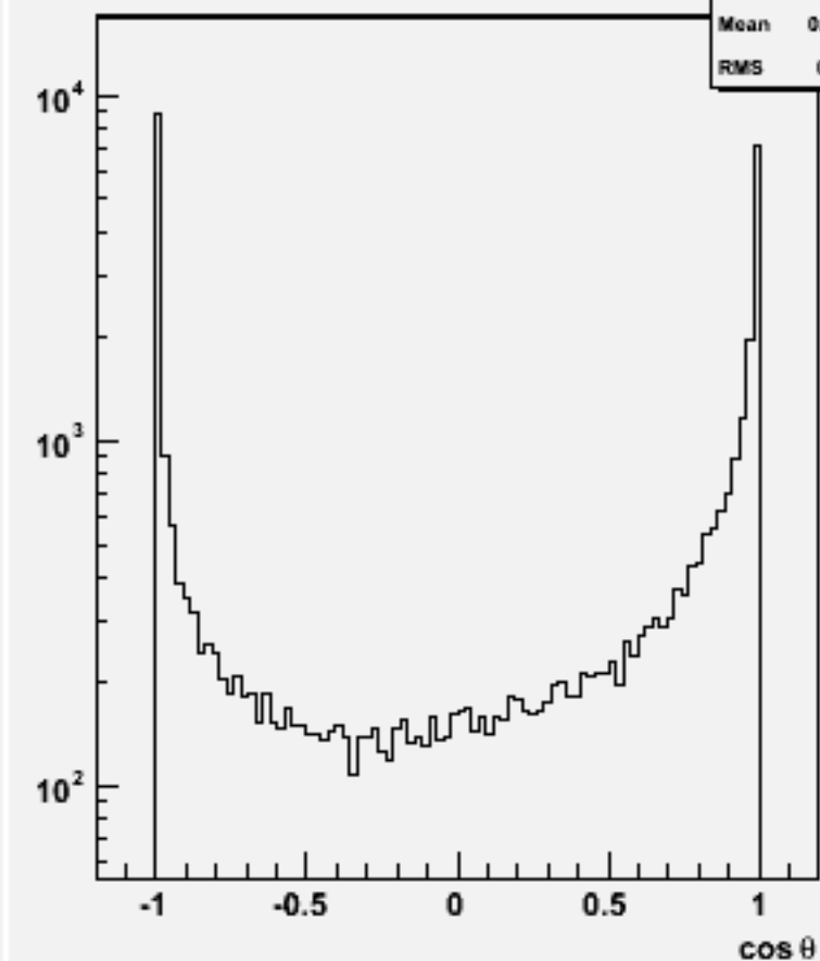
Jet cos \theta (All jets)w103362 e1a_e1e1e1dd_o
