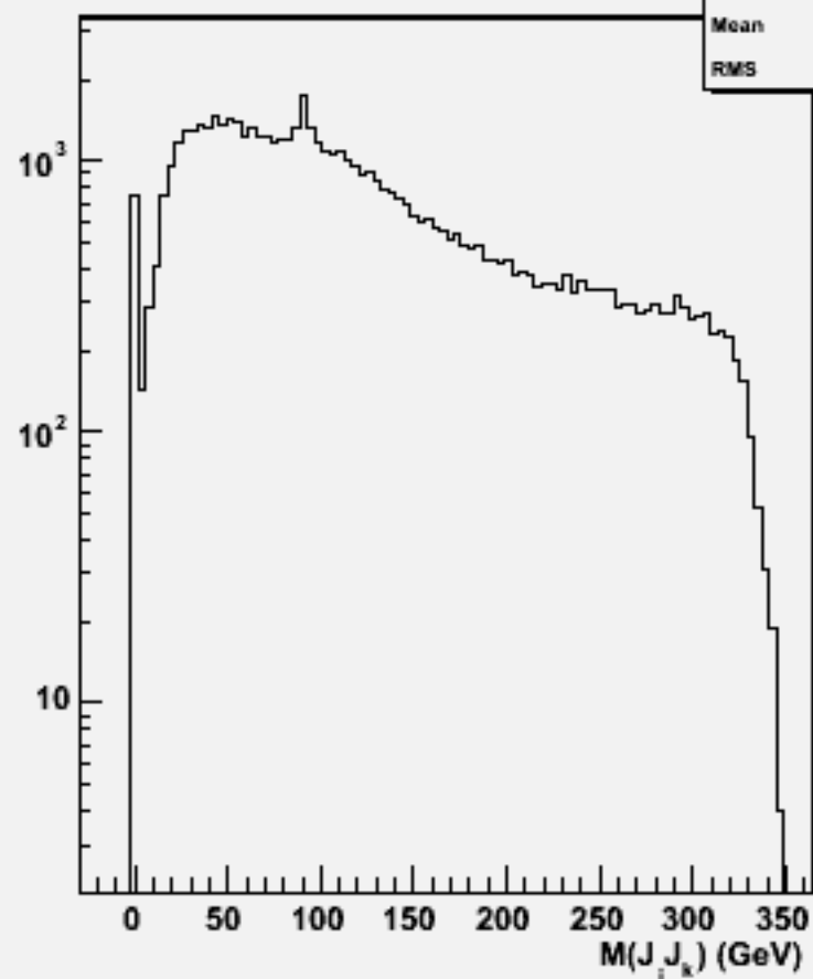
2jets mass(All comb)w103362 e1a_e1e1e1dd_o
