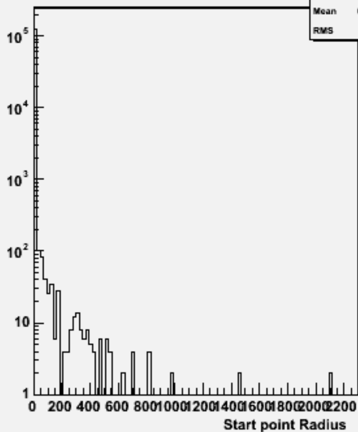
Start point R : w103359 e1a_e1e1e1e3e3_o
