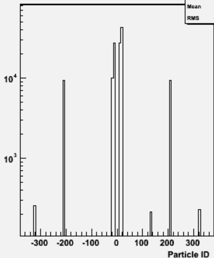
Particle ID : w103359 e1a_e1e1e1e3e3_o
