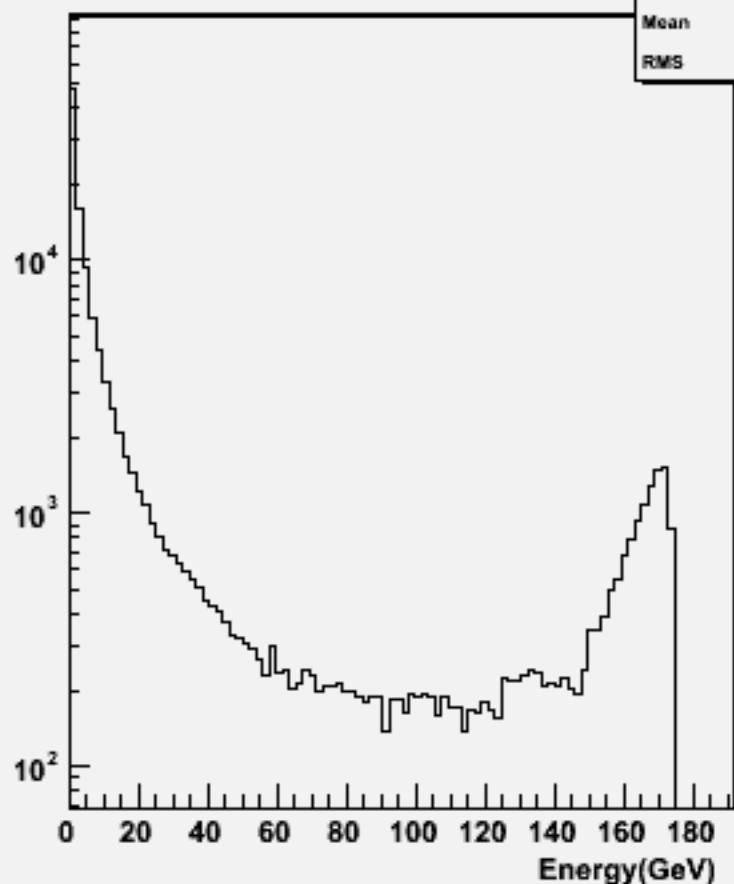
Particle Energy : w103359 e1a_e1e1e1e3e3_o
