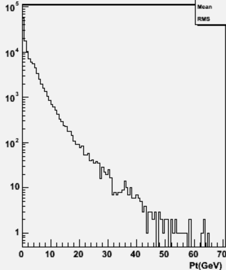
Particle Pt : w103359 e1a_e1e1e1e3e3_o
