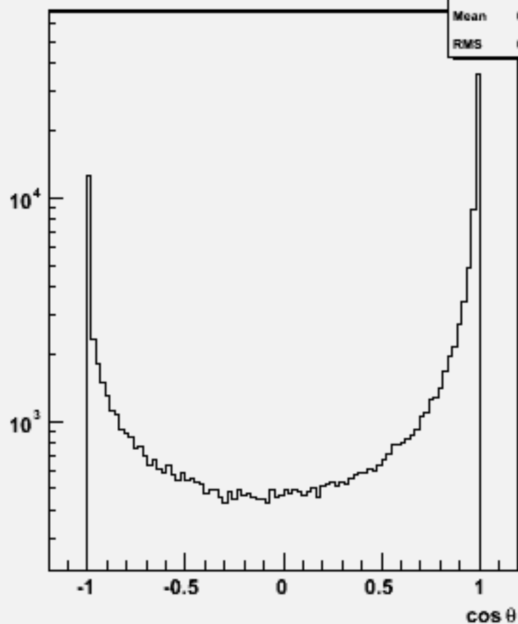
Particle cos \theta : w103359 e1a_e1e1e1e3e3_o
