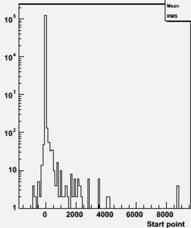
Start point Z : w103359 e1a_e1e1e1e3e3_o
