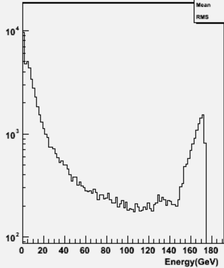
Particle Energy : w103355 e1a_e1e1e1e2e2_o
