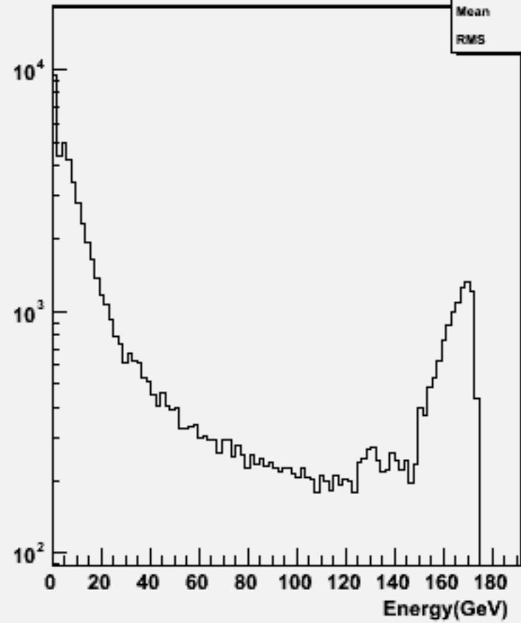
Particle Energy : w103351 e1a_e1e1e1e1e1_o
