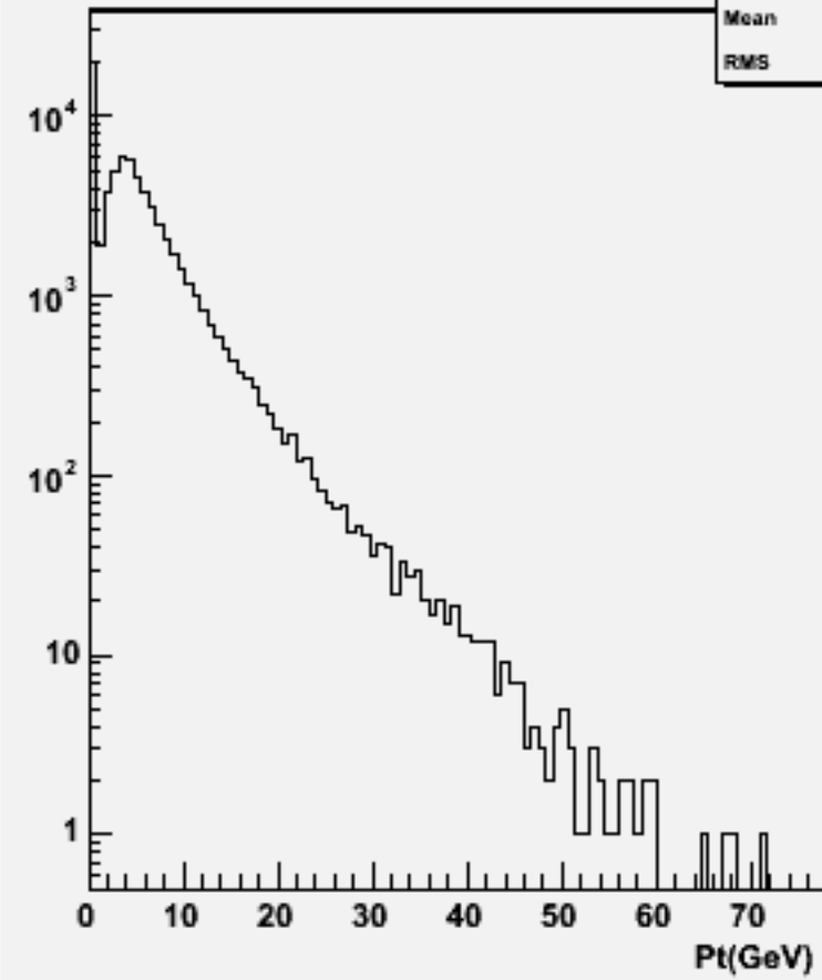
Particle Pt : w103351 e1a_e1e1e1e1e1_o
