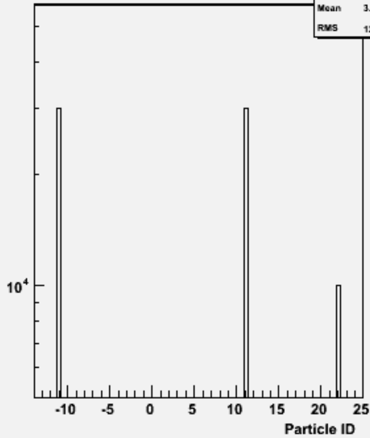
Particle ID : w103351 e1a_e1e1e1e1e1_o
