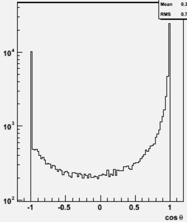
Particle cos \theta : w103351 e1a_e1e1e1e1e1_o
