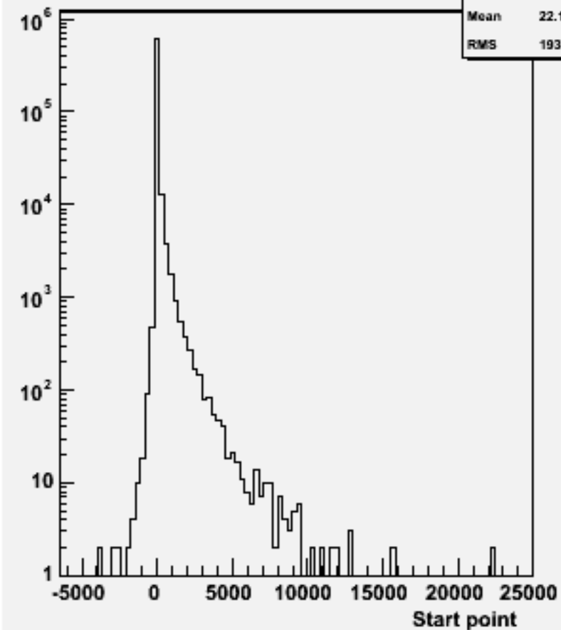
Start point Z : w103349 e1a_e1ccbb_o
