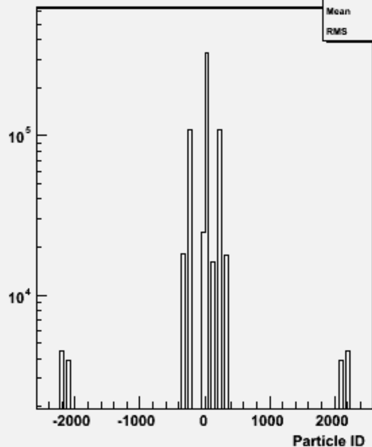
Particle ID : w103349 e1a_e1ccbb_o
