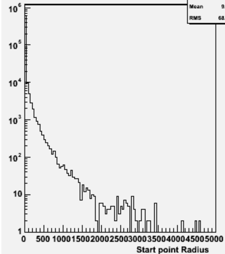
Start point R : w103349 e1a_e1ccbb_o
