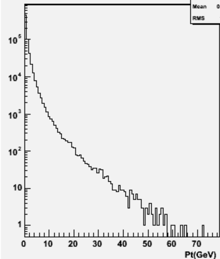
Particle Pt : w103347 e1a_e1ccbb_o
