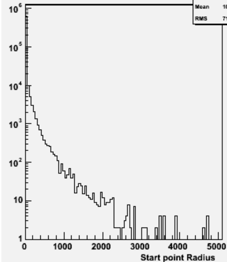
Start point R : w103347 e1a_e1ccbb_o
