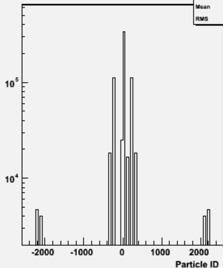
Particle ID : w103347 e1a_e1ccbb_o
