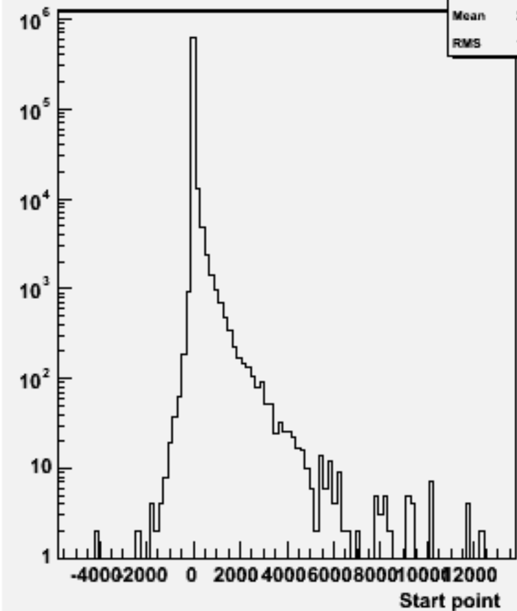
Start point Z : w103347 e1a_e1ccbb_o
