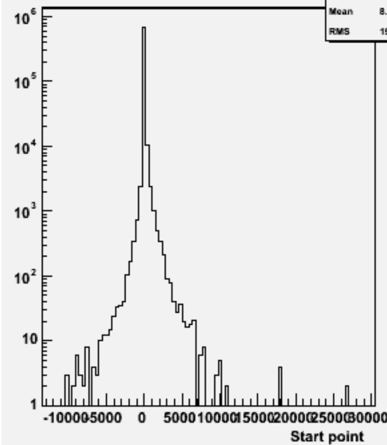
Start point Z : w103344 e1a_e1ccdd_o
