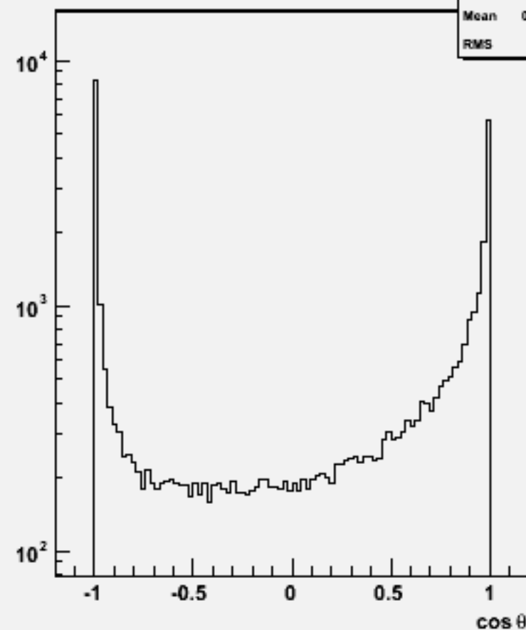
Jet cos \theta (All jets)w103344 e1a_e1ccdd_o
