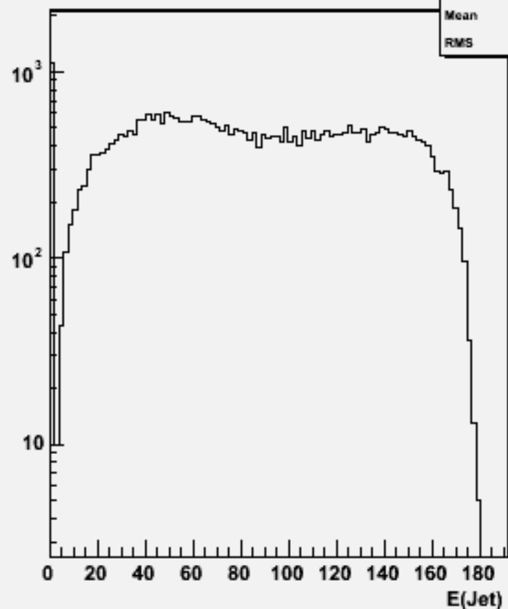
Jet energies(All jets)w103344 e1a_e1ccdd_o
