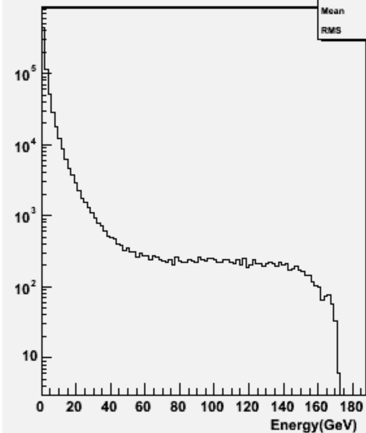
Particle Energy : w103344 e1a_e1ccdd_o
