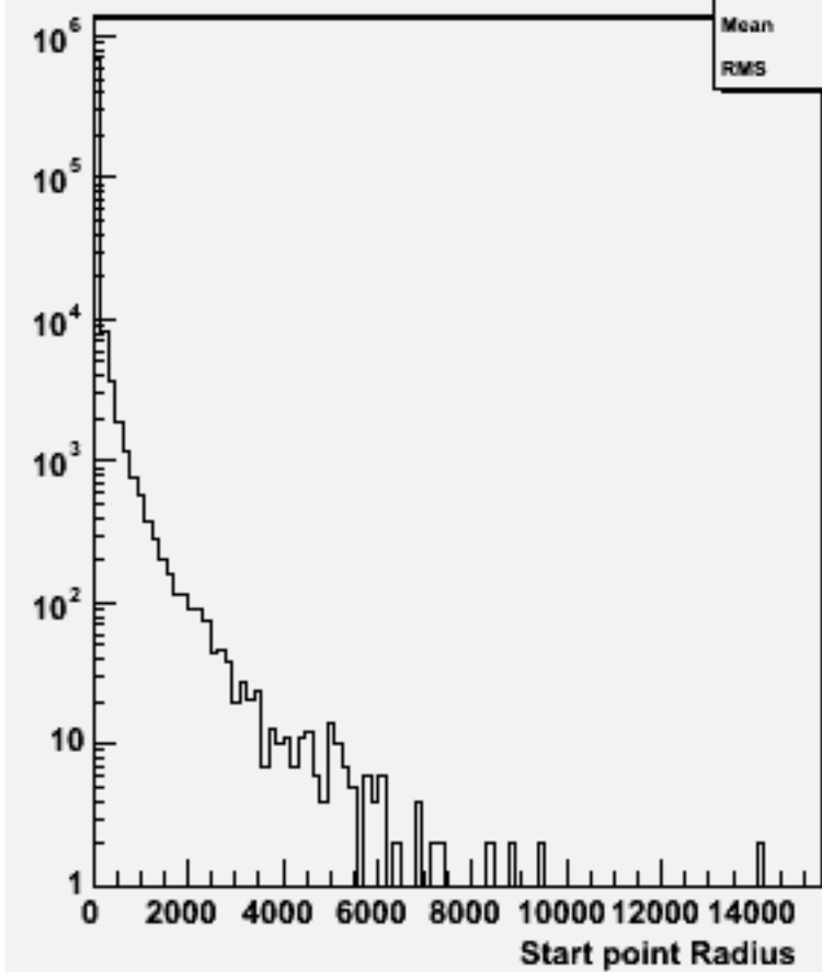
Start point R : w103344 e1a_e1ccdd_o
