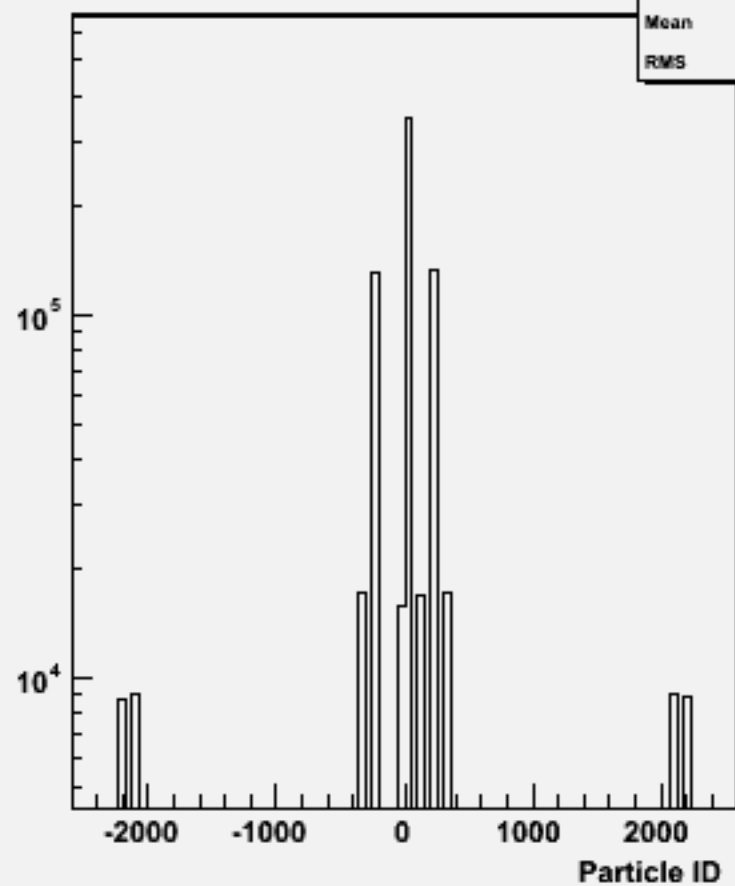
Particle ID : w103344 e1a_e1ccdd_o
