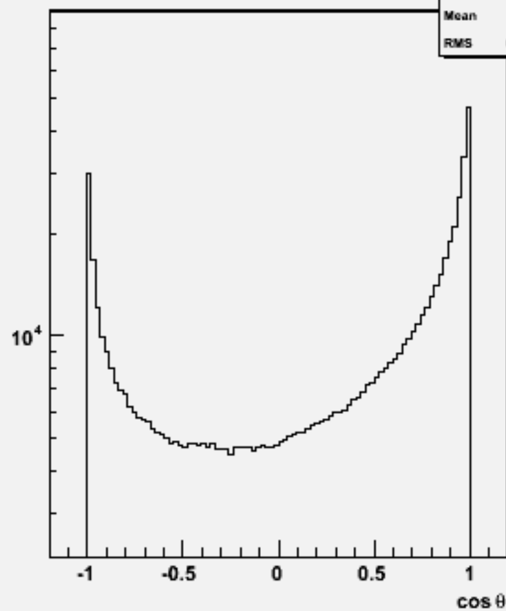
Particle cosθ : w103344 e1a_e1ccdd_o
