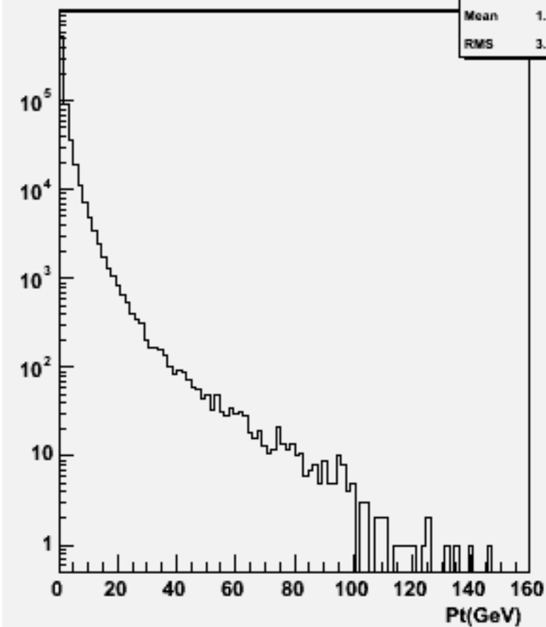
Particle Pt : w103344 e1a_e1ccdd_o
