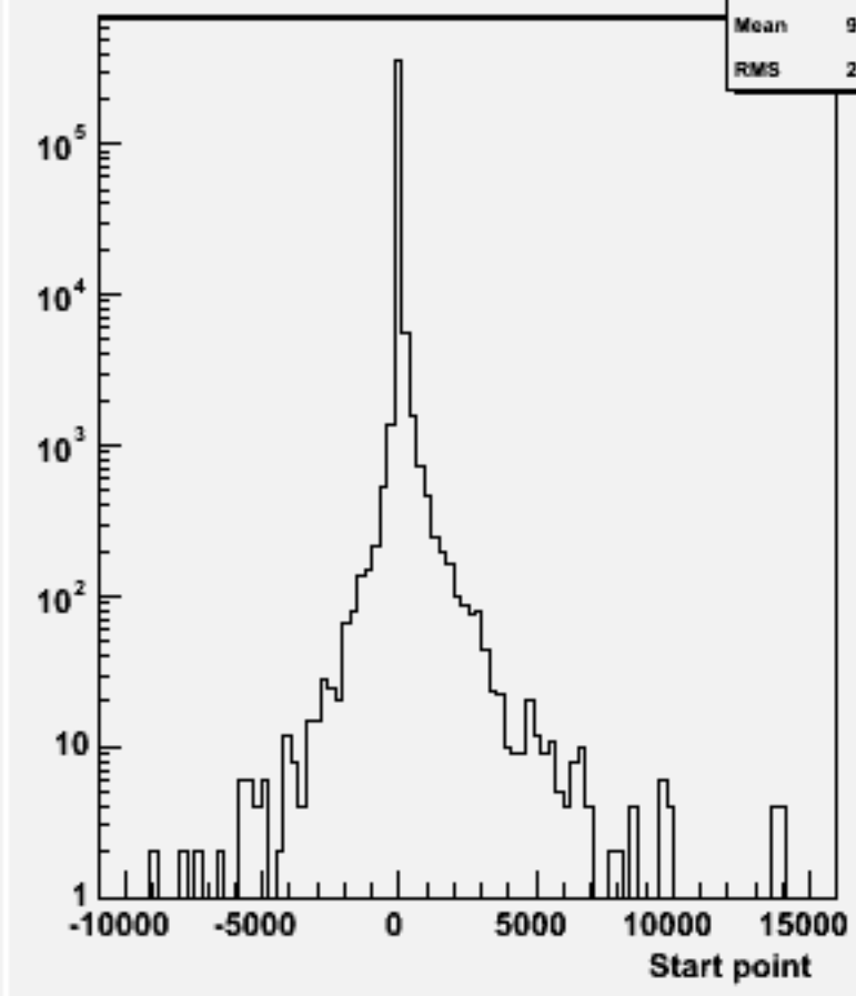
Start point Z : w103340 e1a_e1cce3e3_o
