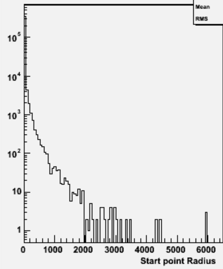
Start point R : w103340 e1a_e1cce3e3_o
