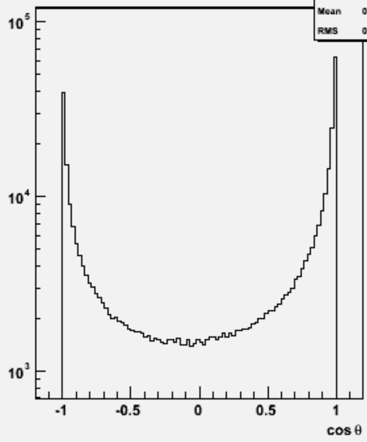
Particle cos \theta : w103340 e1a_e1cce3e3_o
