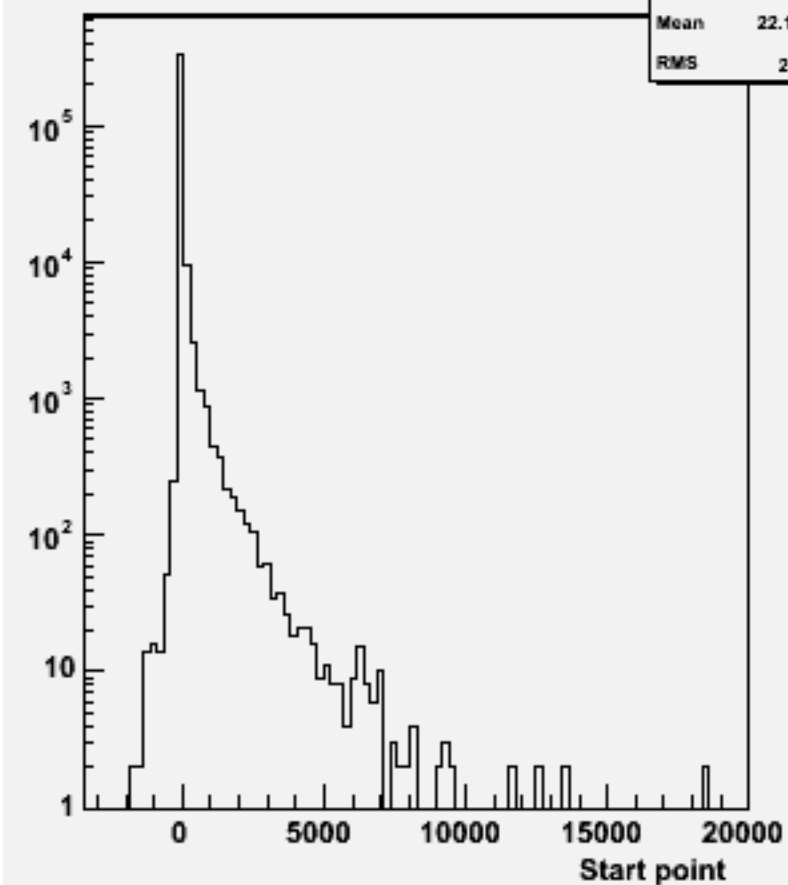
Start point Z : w103339 e1a_e1cce3e3_o
