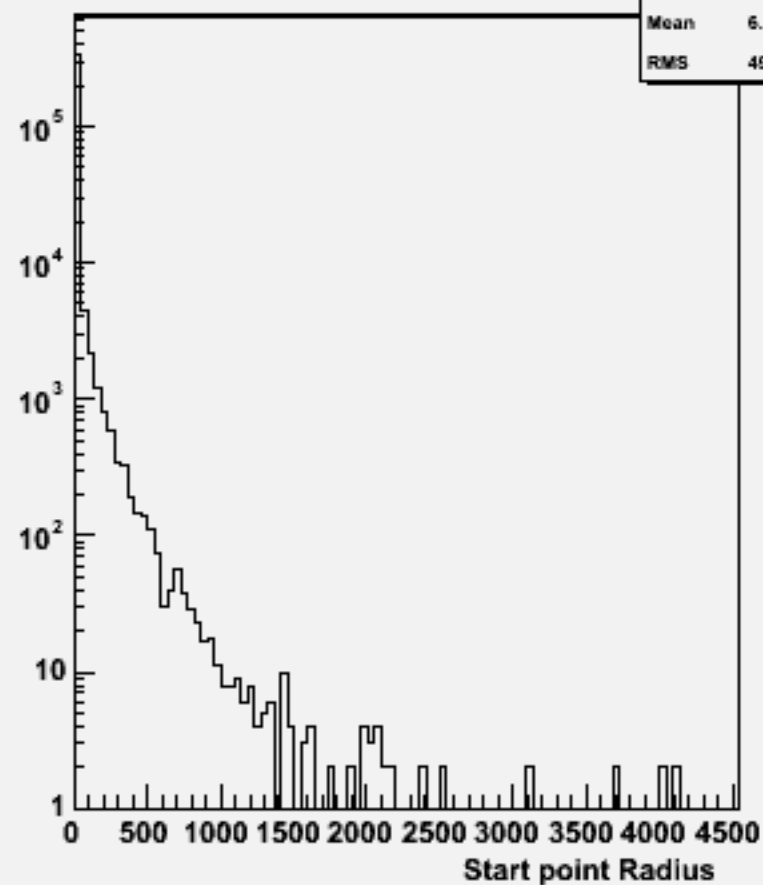
Start point R : w103339 e1a_e1cce3e3_o
