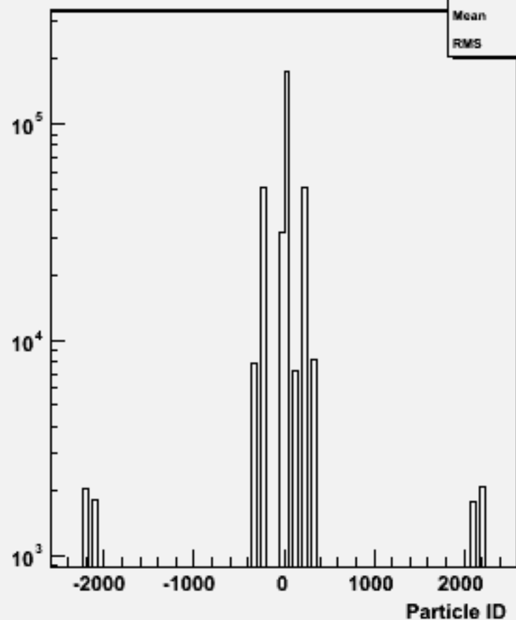
Particle ID : w103339 e1a_e1cce3e3_o
