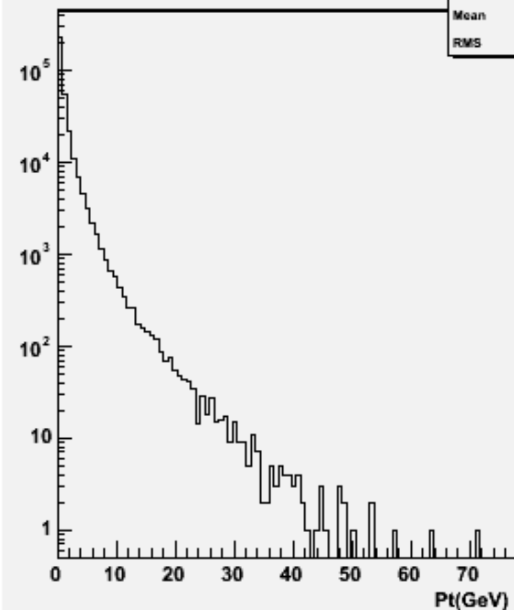
Particle Pt : w103339 e1a_e1cce3e3_o
