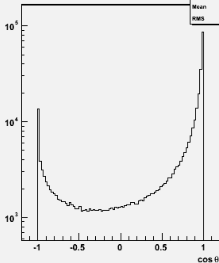
Particle cos \theta : w103339 e1a_e1cce3e3_o
