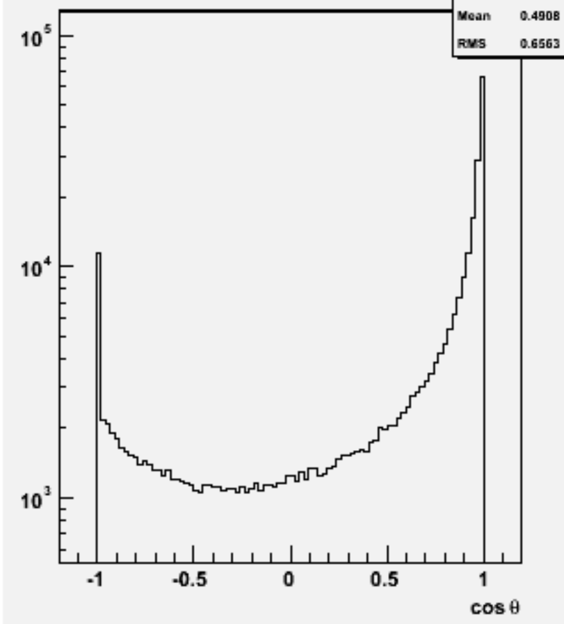
Particle cos θ : w103337 e1a_e1cce2e2_o
