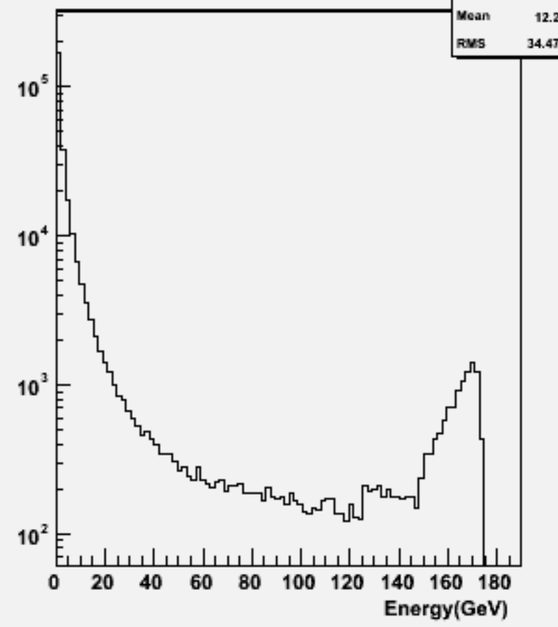
Start point R : w103337 e1a_e1cce2e2_o
