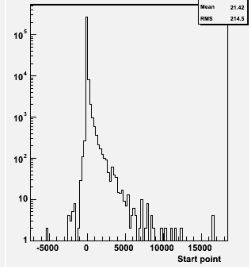
Start point Z : w103337 e1a_e1cce2e2_o
