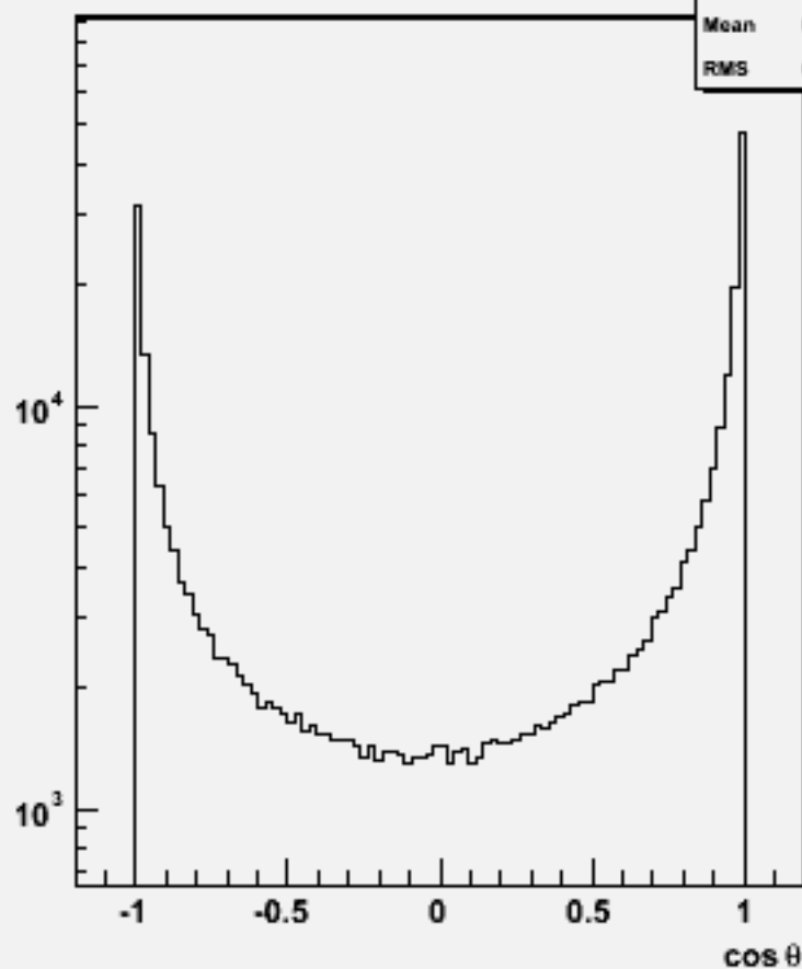
Particle cos \theta : w103336 e1a_e1cce2e2_o
