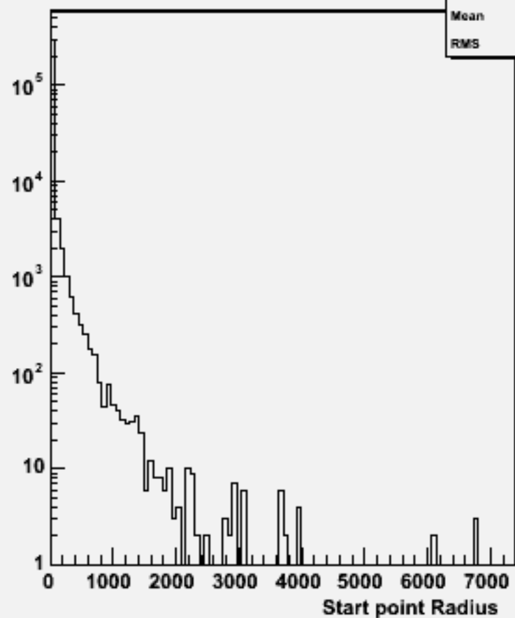
Start point R : w103336 e1a_e1cce2e2_o
