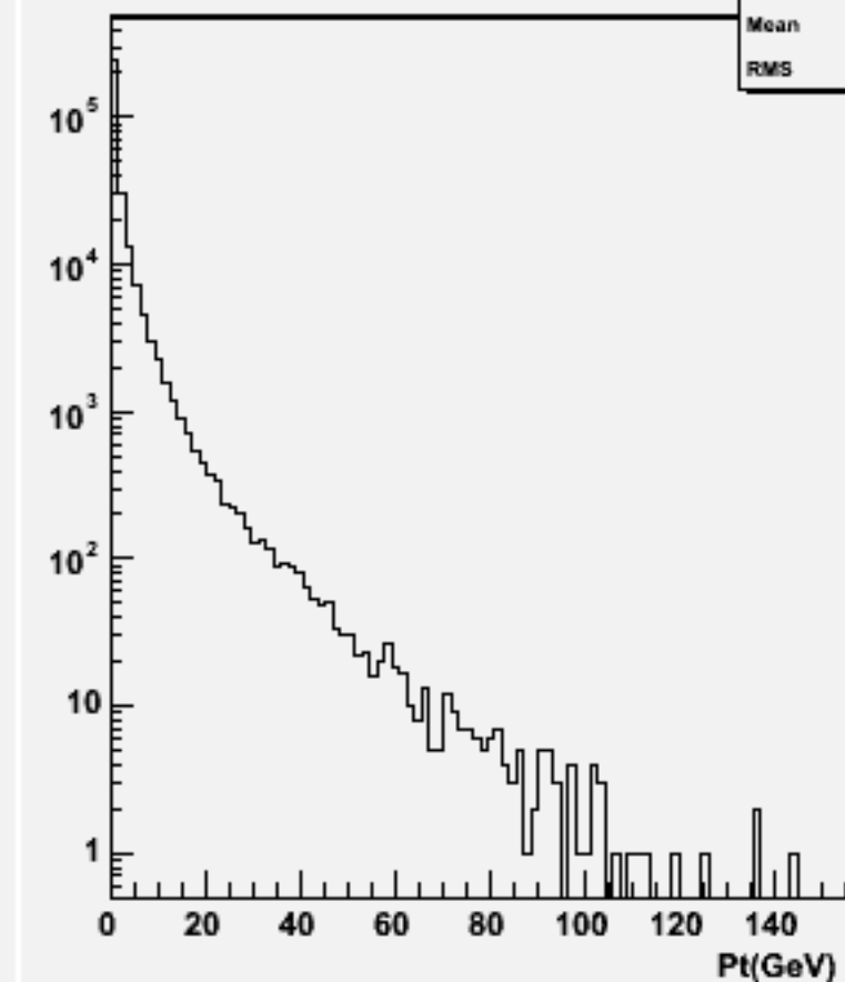
Particle Pt : w103336 e1a_e1cce2e2_o
