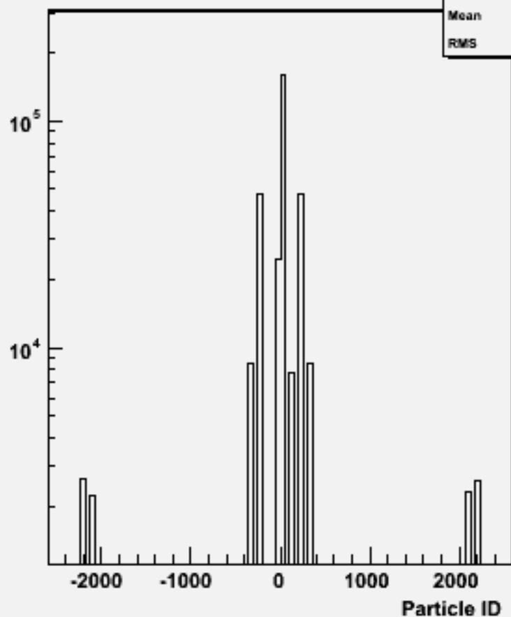
Particle ID : w103336 e1a_e1cce2e2_o
