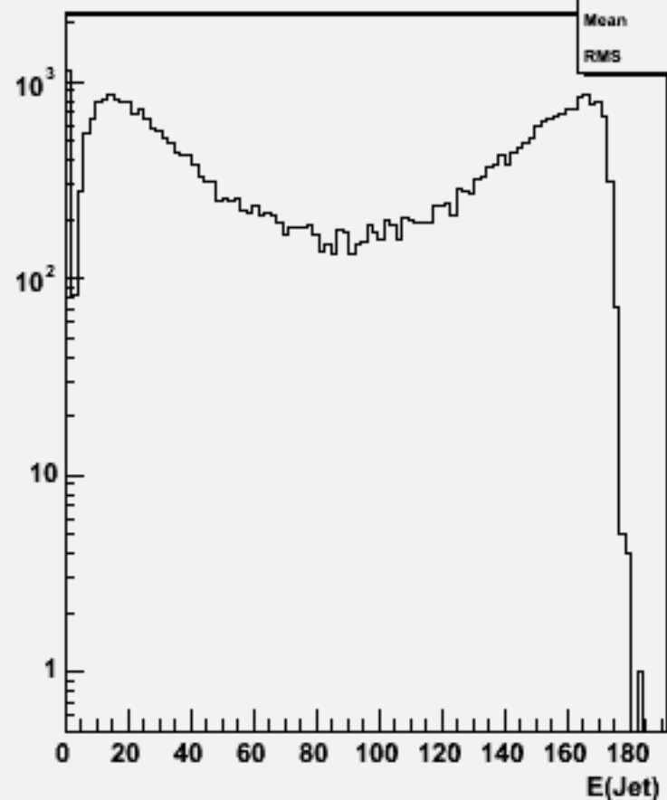
Jet energies(All jets)w103336 e1a_e1cce2e2_o
