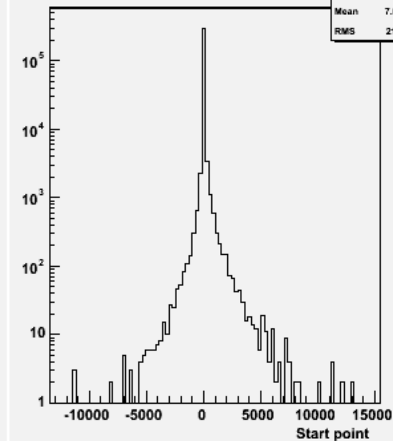
Start point Z : w103336 e1a_e1cce2e2_o
