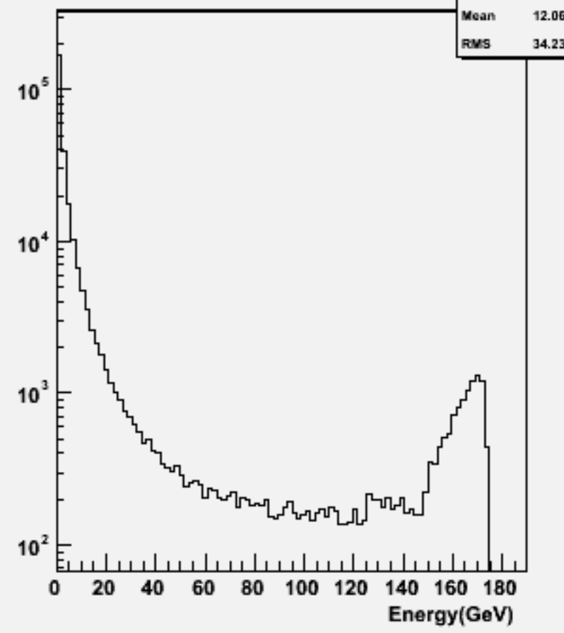
Start point R : w103335 e1a_e1cce2e2_o
