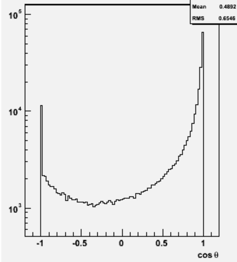
Particle cos \theta : w103335 e1a_e1cce2e2_o
