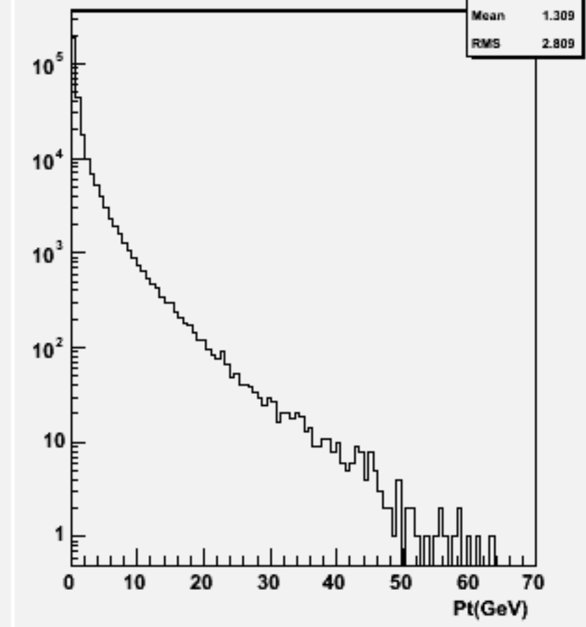
Start point Z : w103335 e1a_e1cce2e2_o
