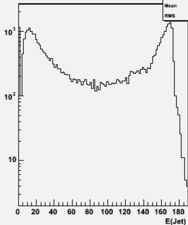
Jet energies(All jets)w103335 e1a_e1cce2e2_o
