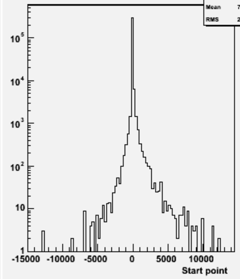
Start point Z : w103334 e1a_e1cce2e2_o
