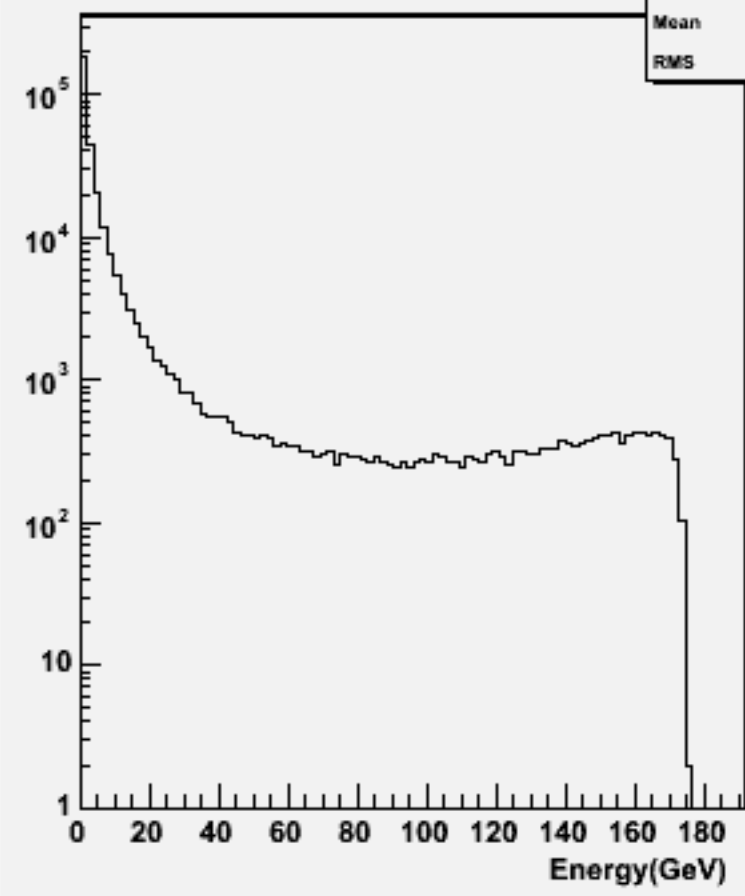
Start point R : w103334 e1a_e1cce2e2_o
