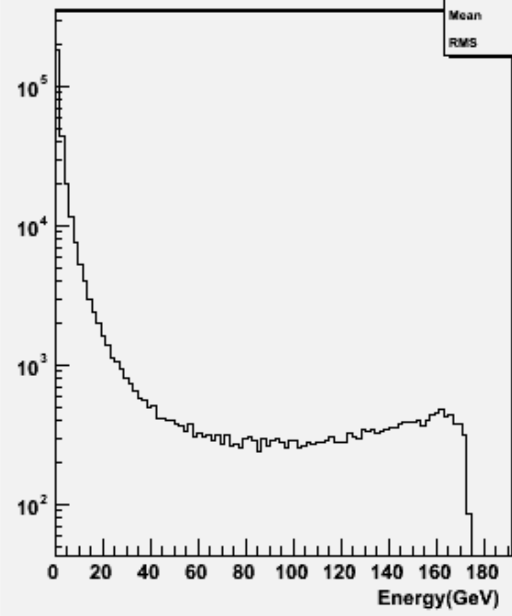
Start point R : w103332 e1a_e1cce1e1_o
