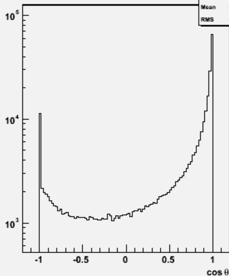
Particle cos \theta : w103331 e1a_e1cce1e1_o
