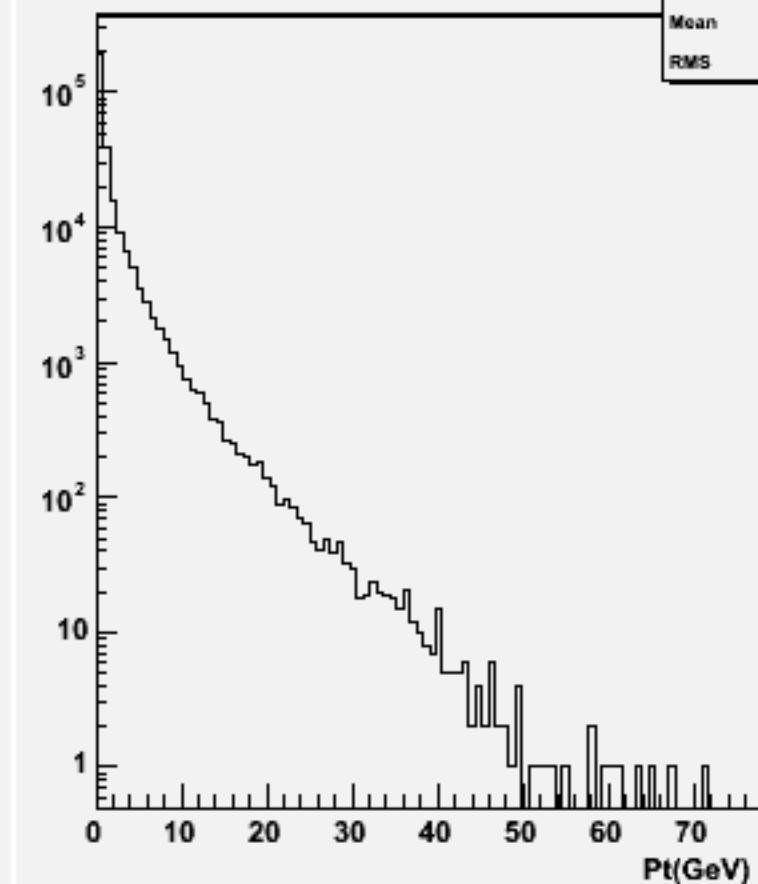
Particle Pt : w103331 e1a_e1cce1e1_o
