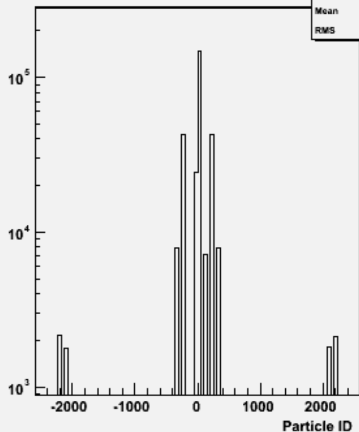
Particle ID : w103331 e1a_e1cce1e1_o
