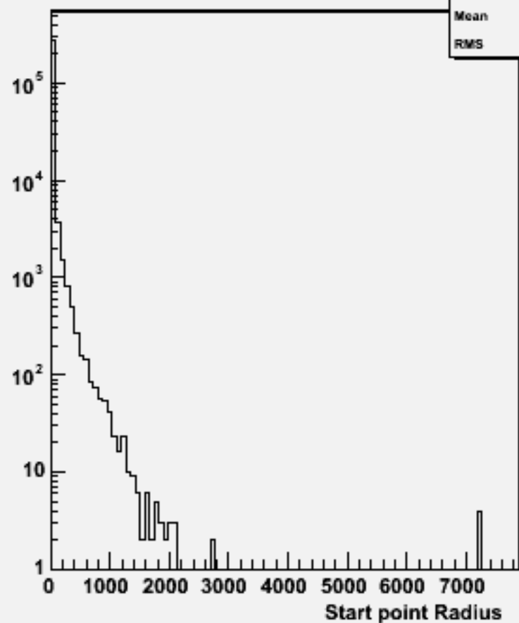
Start point R : w103331 e1a_e1cce1e1_o
