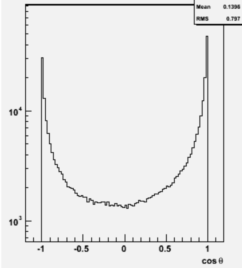
Particle cos θ : w103330 e1a_e1cce1e1_o
