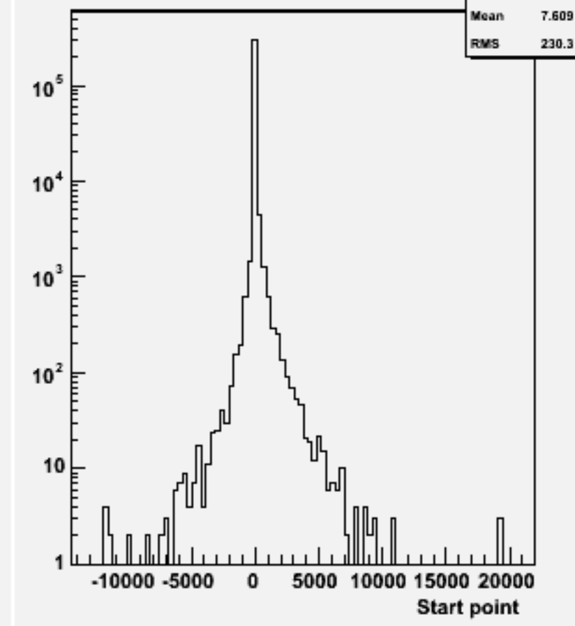
Start point Z : w103330 e1a_e1cce1e1_o
