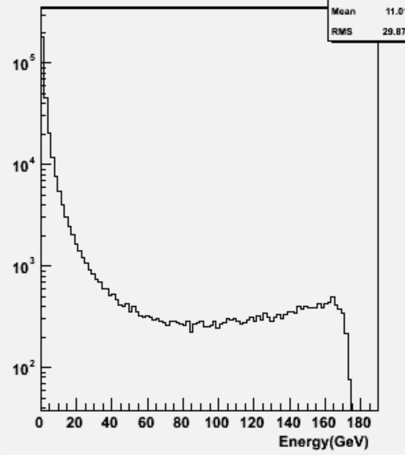
Start point R : w103330 e1a_e1cce1e1_o
