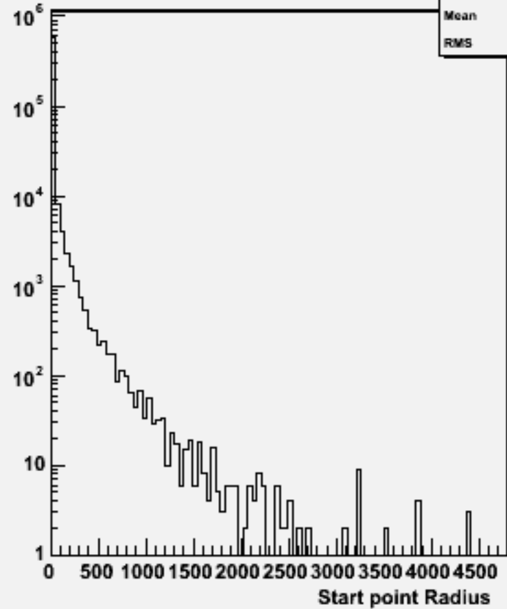
Start point R : w103329 e1a_e1uubb_o
