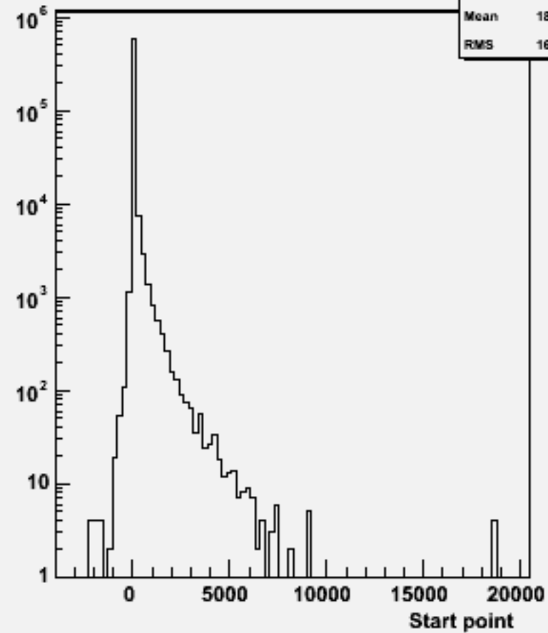
Start point Z : w103329 e1a_e1uubb_o
