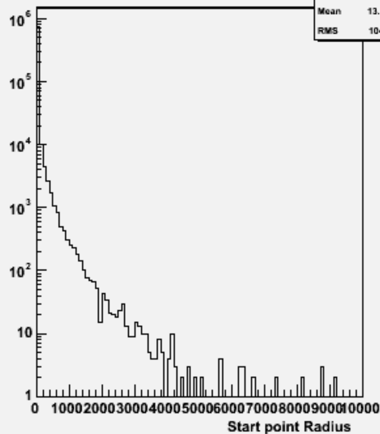
Start point R : w103328 e1a_e1uubb_o
