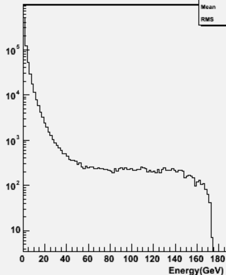
Start point R : w103328 e1a_e1uubb_o
